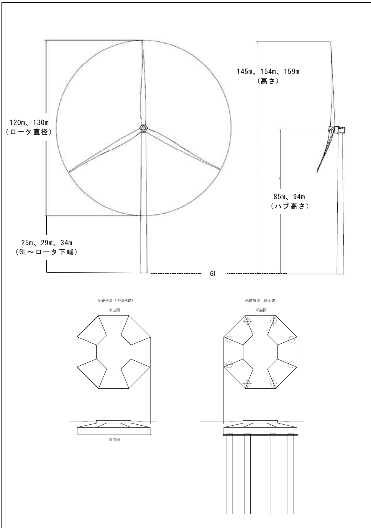
第 2.2-9 図 風力発電機の外形図及び基礎構造
