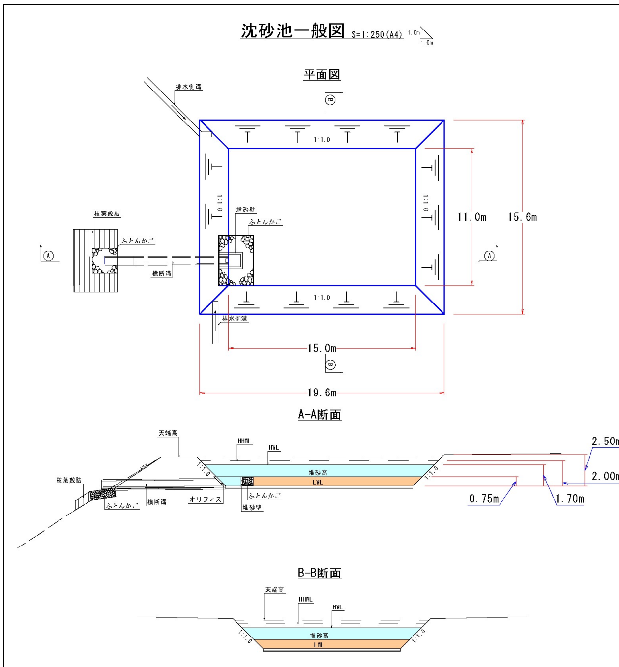
第 2.2-8 図 沈砂池の構造 (例)
