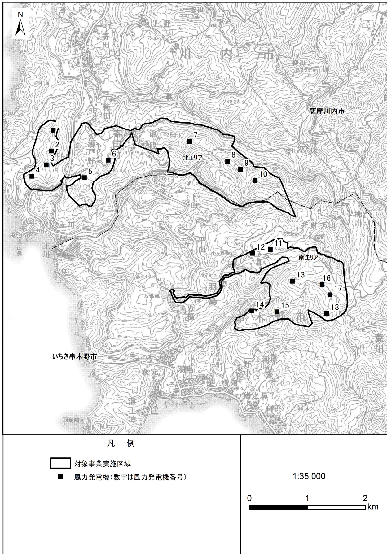
第 2.2-3 図 風力発電機の配置計画
