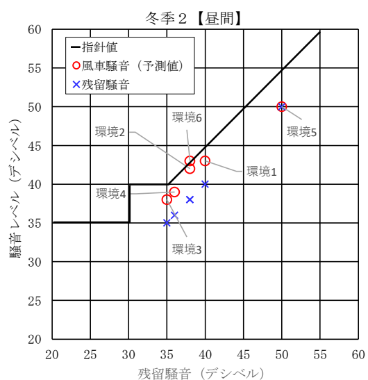
第 10.1.1-33 図 残留騒音、風車騒音（予測値）、指針値の関係（累積的な影響）
