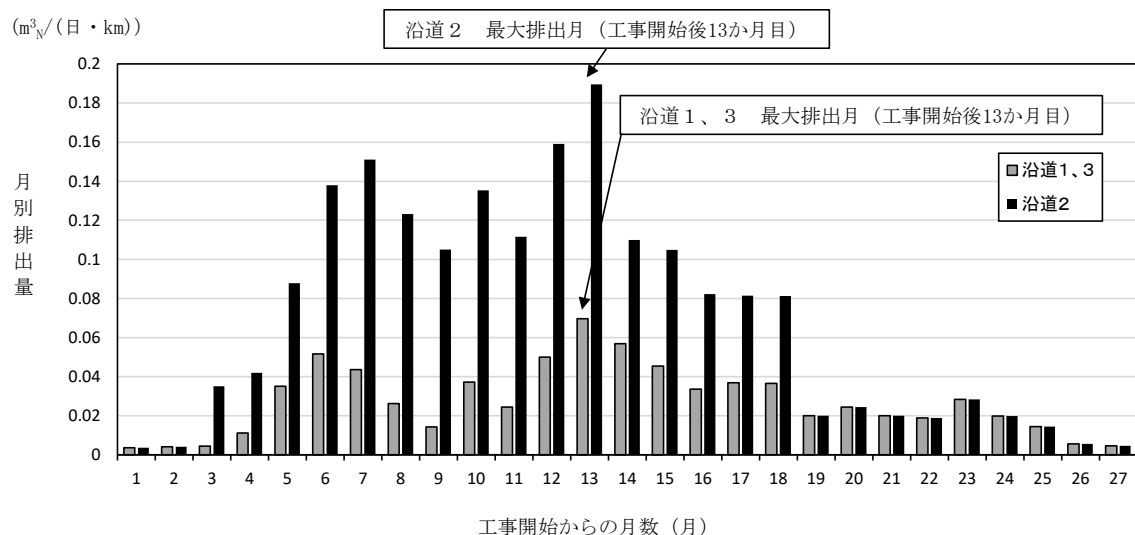
第10.1.1-6図 工事関係車両による窒素酸化物の月別排出量
