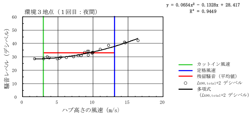
第 10.1.1-22 図(3) ハブ高さ風速と騒音レベル ( L_{A90+2} ) (1 回目：環境3地点)
