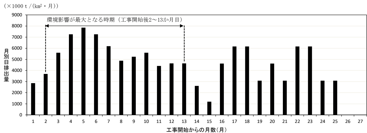
第 10.1.1-16 図 建設機械の稼働による粉じん等の月別排出量
