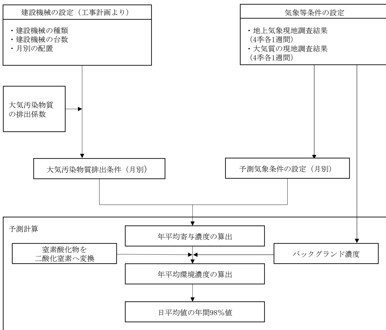
第10.1.1-14図 建設機械の稼働に伴う二酸化窒素濃度の予測手順
