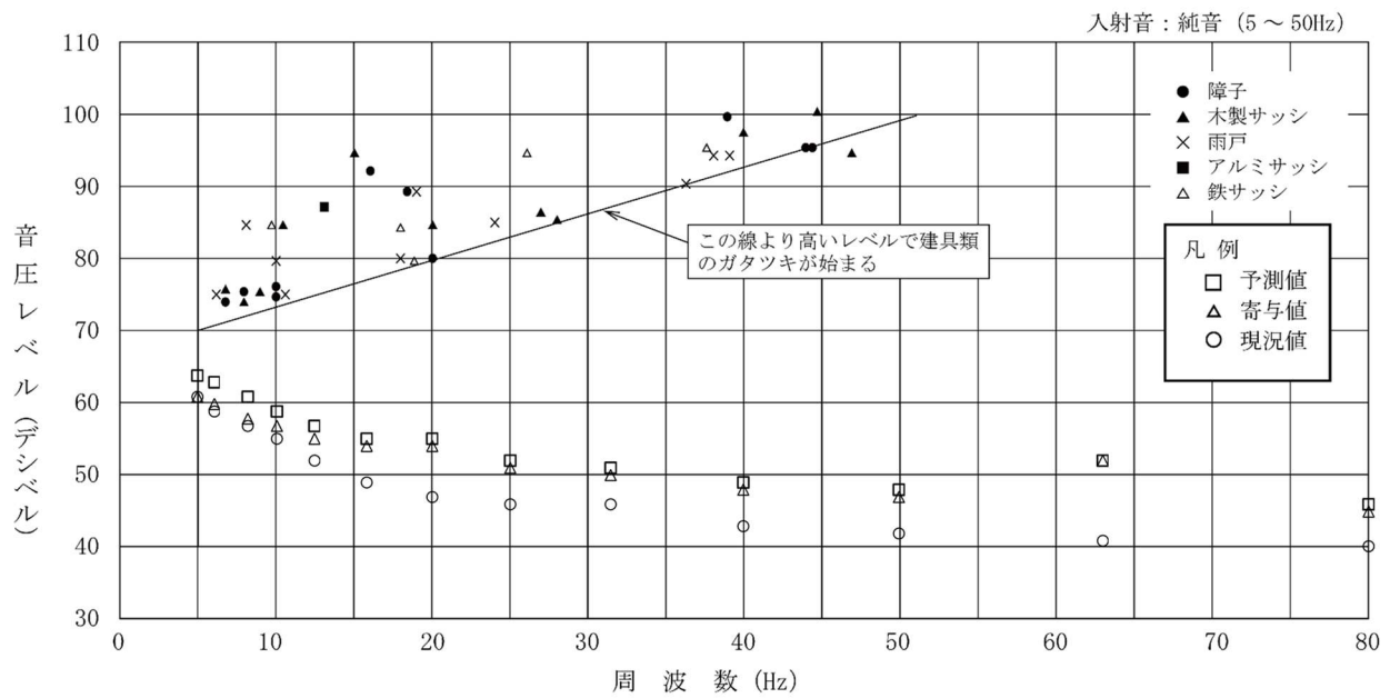
第 10.1.1-38 図(2) 建具のがたつきが始まるレベルとの比較結果 (本事業：環境2地点、冬季1)
