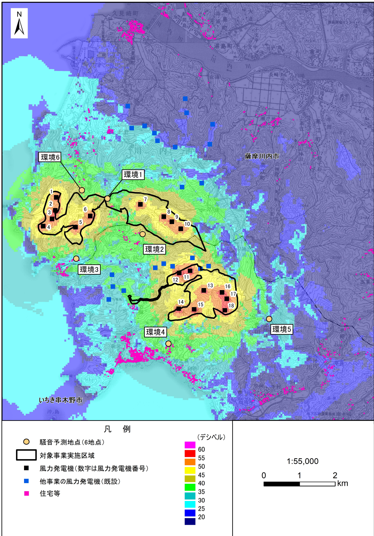
第 10.1.1-30 図(1) 風力発電機から発生する騒音の寄与の状況 (本事業、冬季1昼間、環境1～5調査時)
