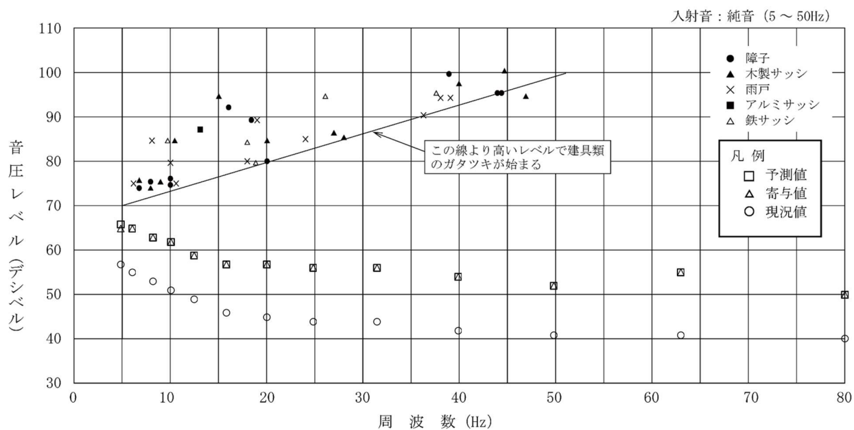
第 10.1.1-45 図(2) 建具のがたつきが始まるレベルとの比較結果 (累積的な影響：環境2地点、冬季2)
