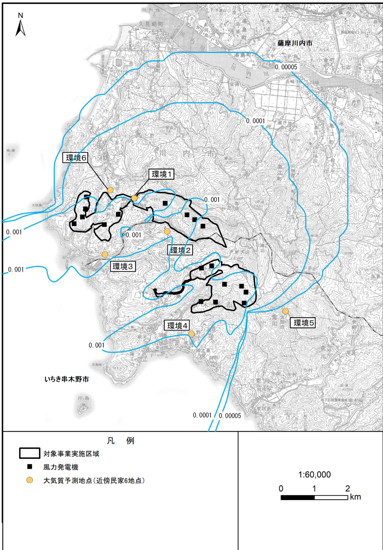
第 10.1.1-15 図(1) 建設機械の稼働に伴う二酸化窒素濃度の予測結果 (予測地点環境 1 が最大となった月：工事開始後 8 か月目、気象条件：夏季)
