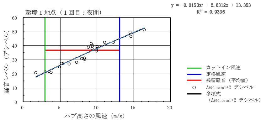
第 10.1.1-22 図(1) ハブ高さ風速と騒音レベル ( L_{A90}+2 ) (1 回目：環境1地点)
