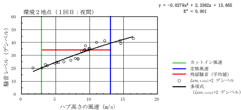
第 10.1.1-22 図(2) ハブ高さ風速と騒音レベル ( L_{A90}+2 ) (1 回目：環境2地点)
