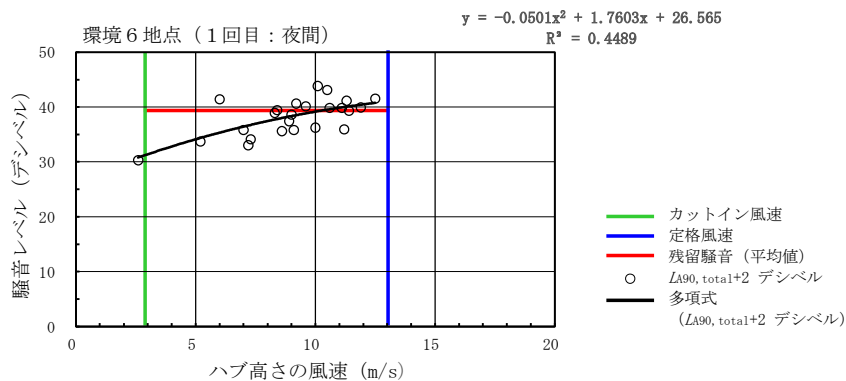
第 10.1.1-22 図(6) ハブ高さ風速と騒音レベル ( L_{A90}+2 ) (1回目：環境6地点)
