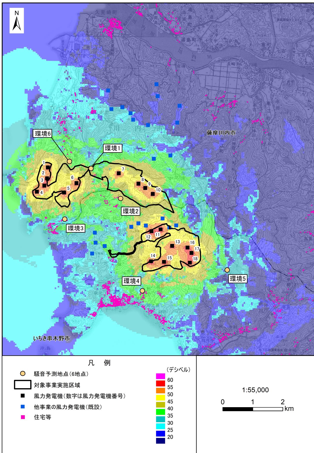
第 10.1.1-30 図(4) 風力発電機から発生する騒音の寄与の状況 (本事業、冬季2夜間、環境1～5調査時)
