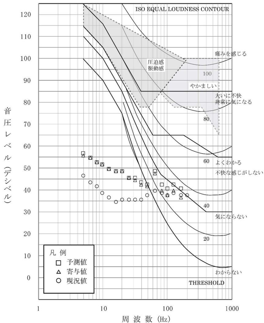
第 10.1.1-39 図(5) 圧迫感・振動感を感じる音圧レベルとの比較結果 (本事業：環境 5 地点、冬季 1)
