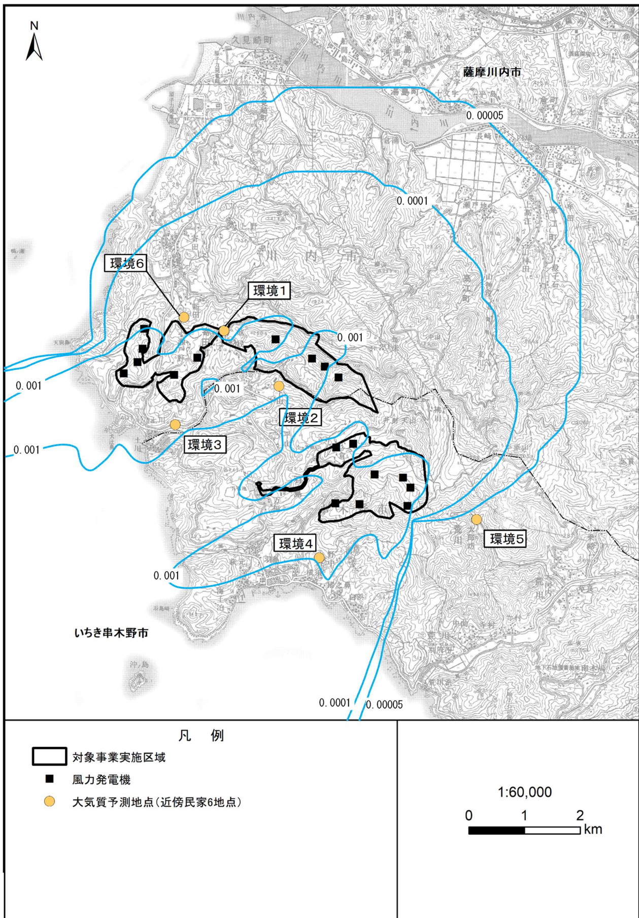
第 10.1.1-15 図 (3) 建設機械の稼働に伴う二酸化窒素濃度の予測結果 (予測地点環境 3 が最大となった月：工事開始後 8 か月目、気象条件：夏季)
