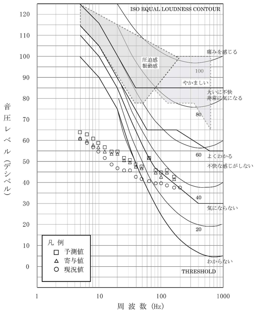
第 10.1.1-39 図(2) 圧迫感・振動感を感じる音圧レベルとの比較結果 (本事業：環境2地点、冬季1)
