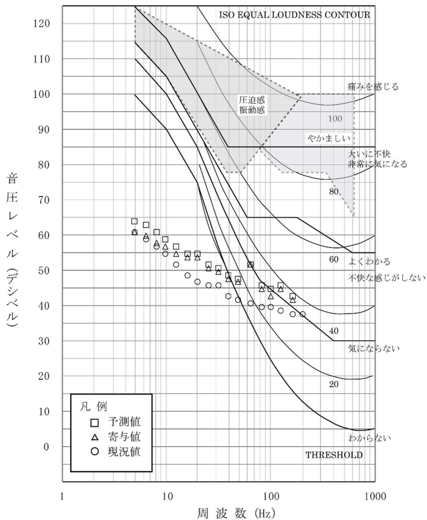
第 10.1.1-39 図 (3) 圧迫感・振動感を感じる音圧レベルとの比較結果 (本事業：環境 3 地点、冬季 1)
