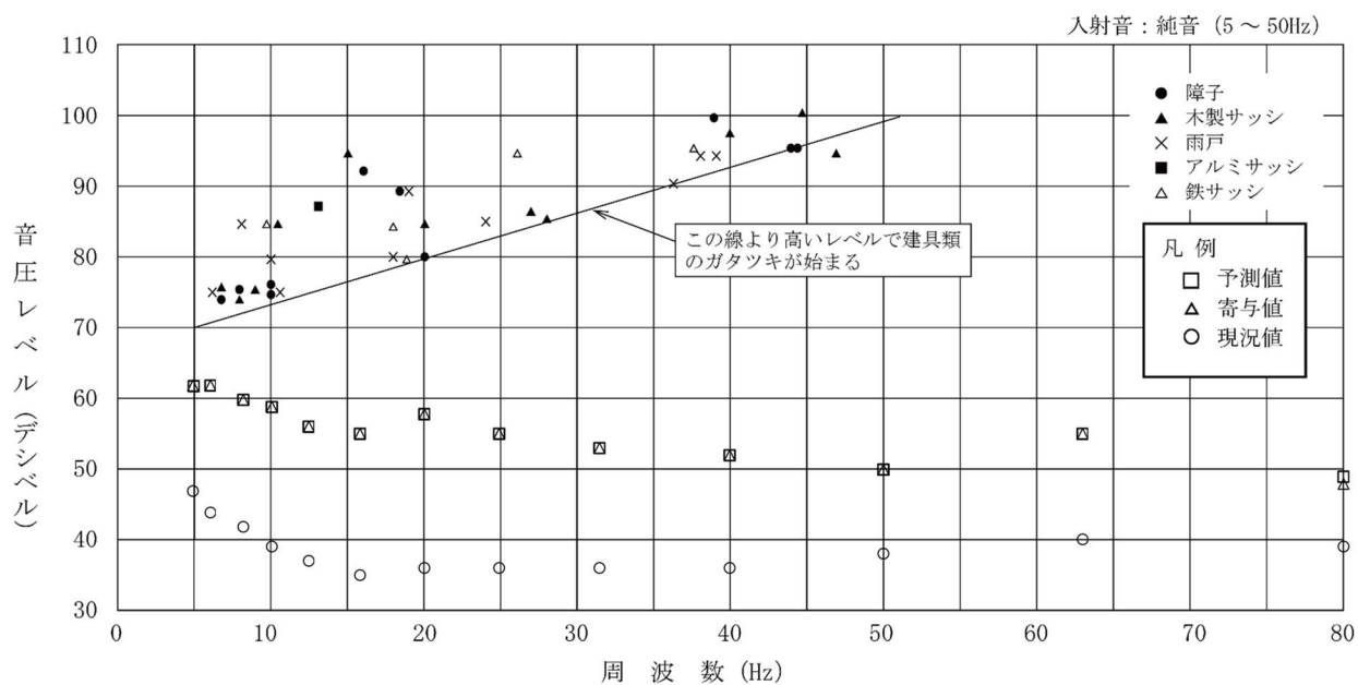
第 10.1.1-43 図(5) 建具のがたつきが始まるレベルとの比較結果 (累積的な影響：環境 5 地点、冬季 1)
