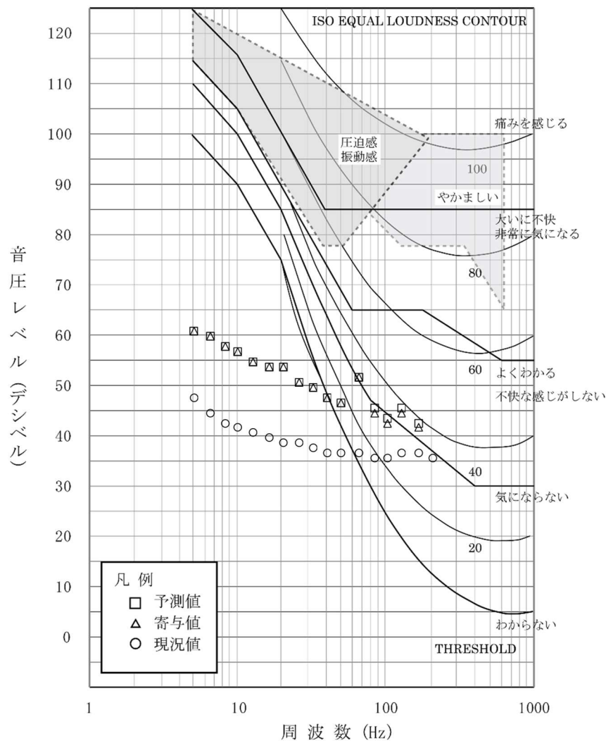
第 10.1.1-41 図(6) 圧迫感・振動感を感じる音圧レベルとの比較結果 (本事業：環境 6 地点、冬季 2)
