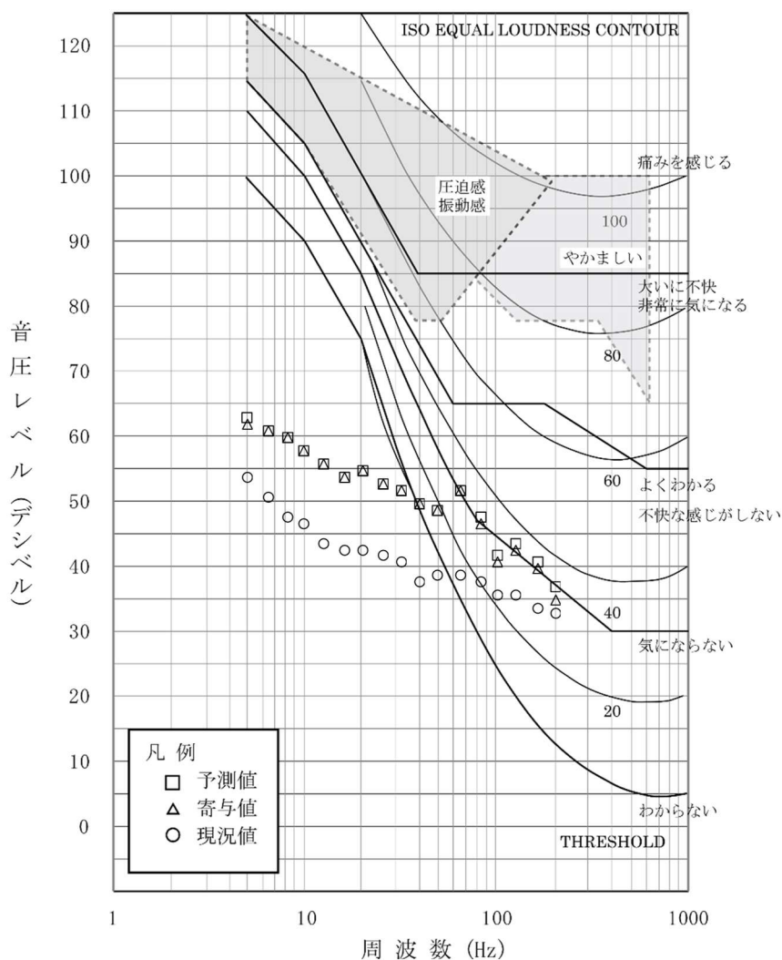
第 10.1.1-46 図(4) 圧迫感・振動感を感じる音圧レベルとの比較結果 (累積的な影響：環境4地点、冬季2)
