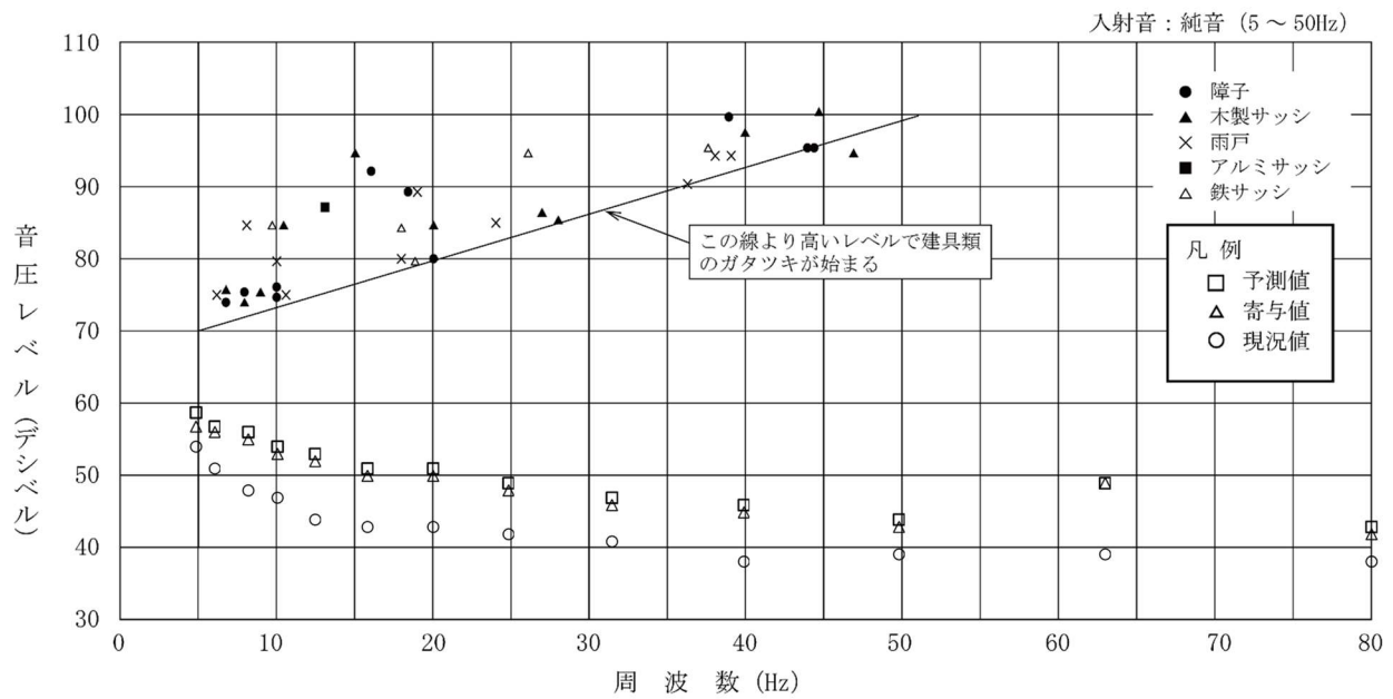
第 10.1.1-40 図(4) 建具のがたつきが始まるレベルとの比較結果 (本事業：環境4地点、冬季2)
