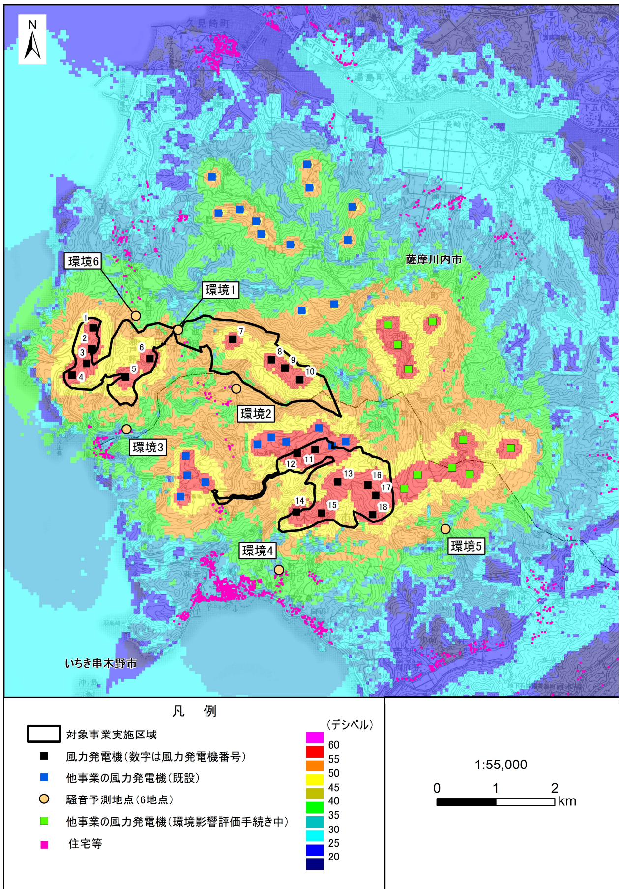
第 10.1.1-32 図(3) 風力発電機から発生する騒音の寄与の状況 (累積的な影響、冬季2昼間、環境1～5調査時)
