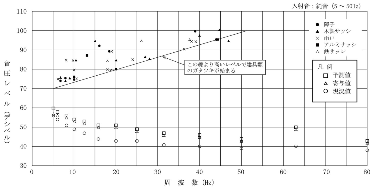
第 10. 1. 1-38 図(4) 建具のがたつきが始まるレベルとの比較結果 (本事業：環境4地点、冬季1)
