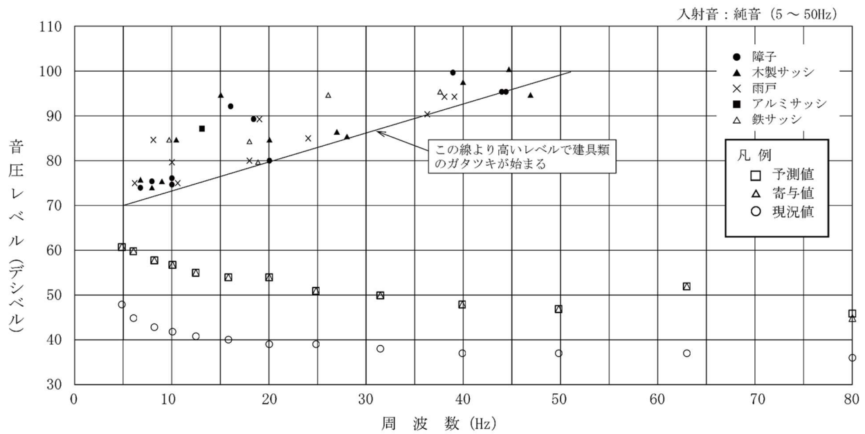
第 10.1.1-40 図(6) 建具のがたつきが始まるレベルとの比較結果 (本事業：環境 6 地点、冬季 2)
