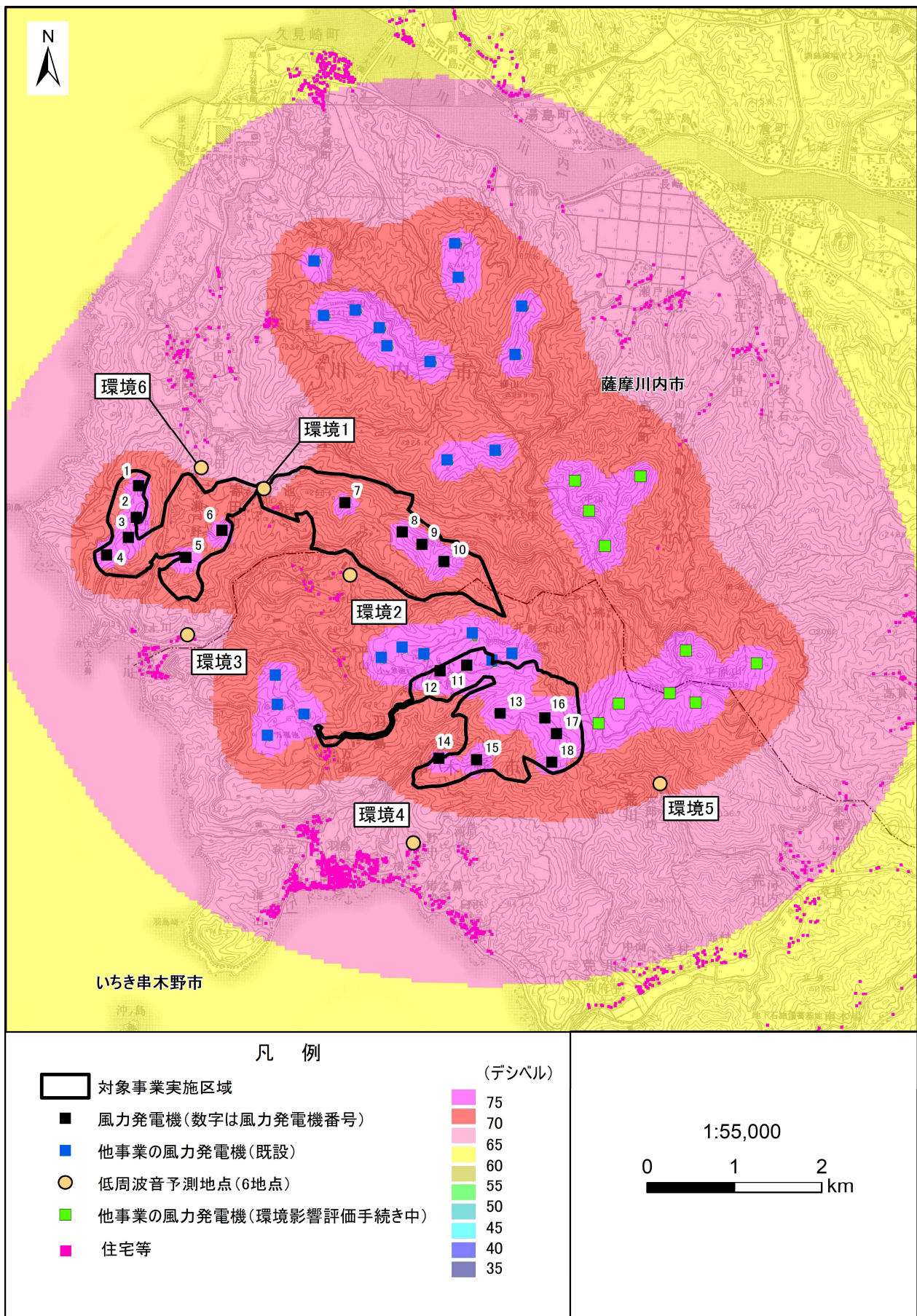
第 10.1.1-42 図 風力発電機から発生する G 特性音圧レベルの寄与値（累積的な影響）
