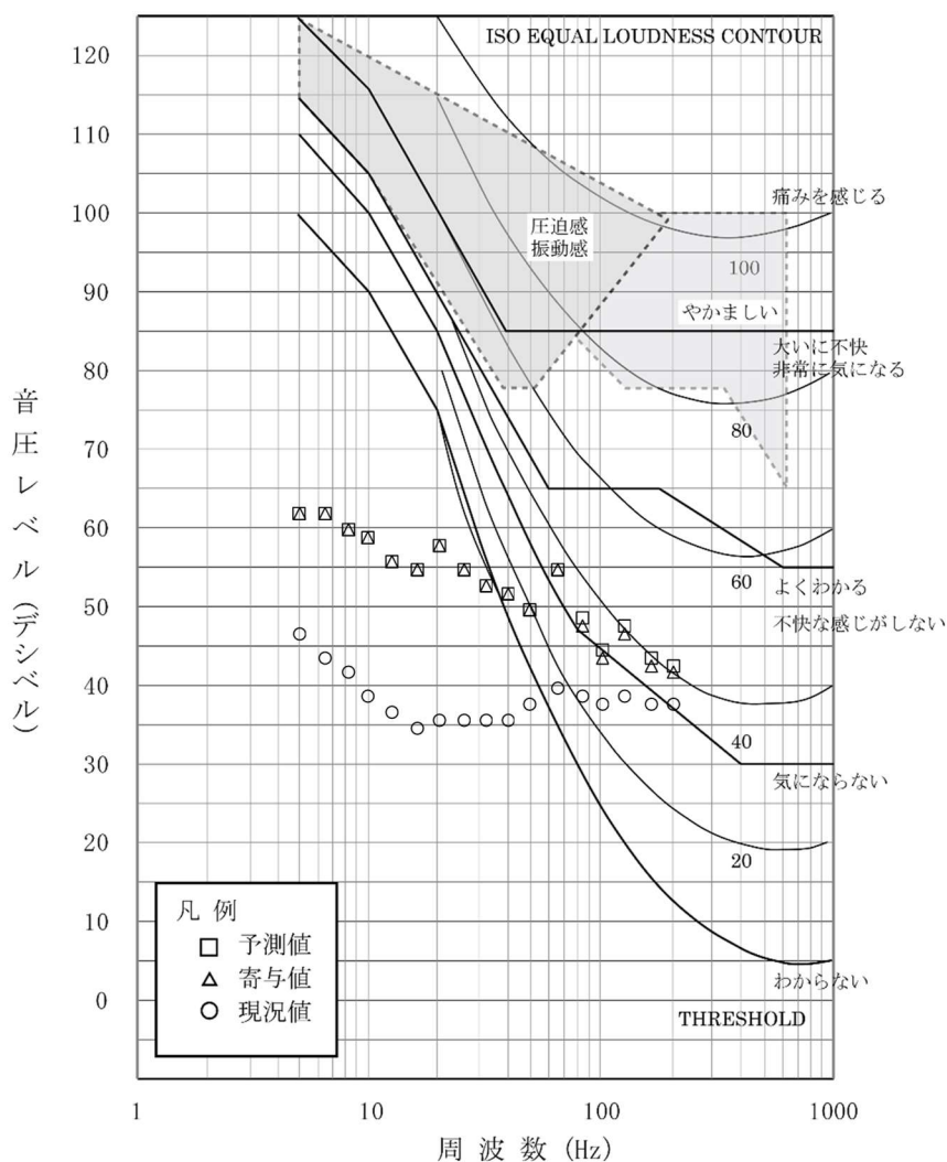
第 10.1.1-44 図(5) 圧迫感・振動感を感じる音圧レベルとの比較結果 (累積的な影響：環境 5 地点、冬季 1)
