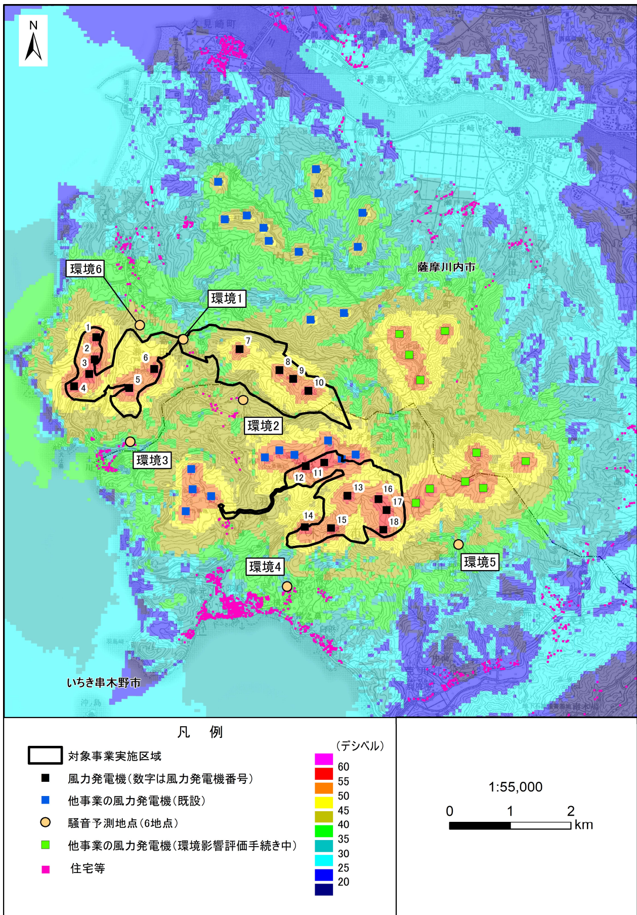
第 10.1.1-32 図(6) 風力発電機から発生する騒音の寄与の状況 (累積的な影響、冬季 1 夜間、環境 6 調査時)
