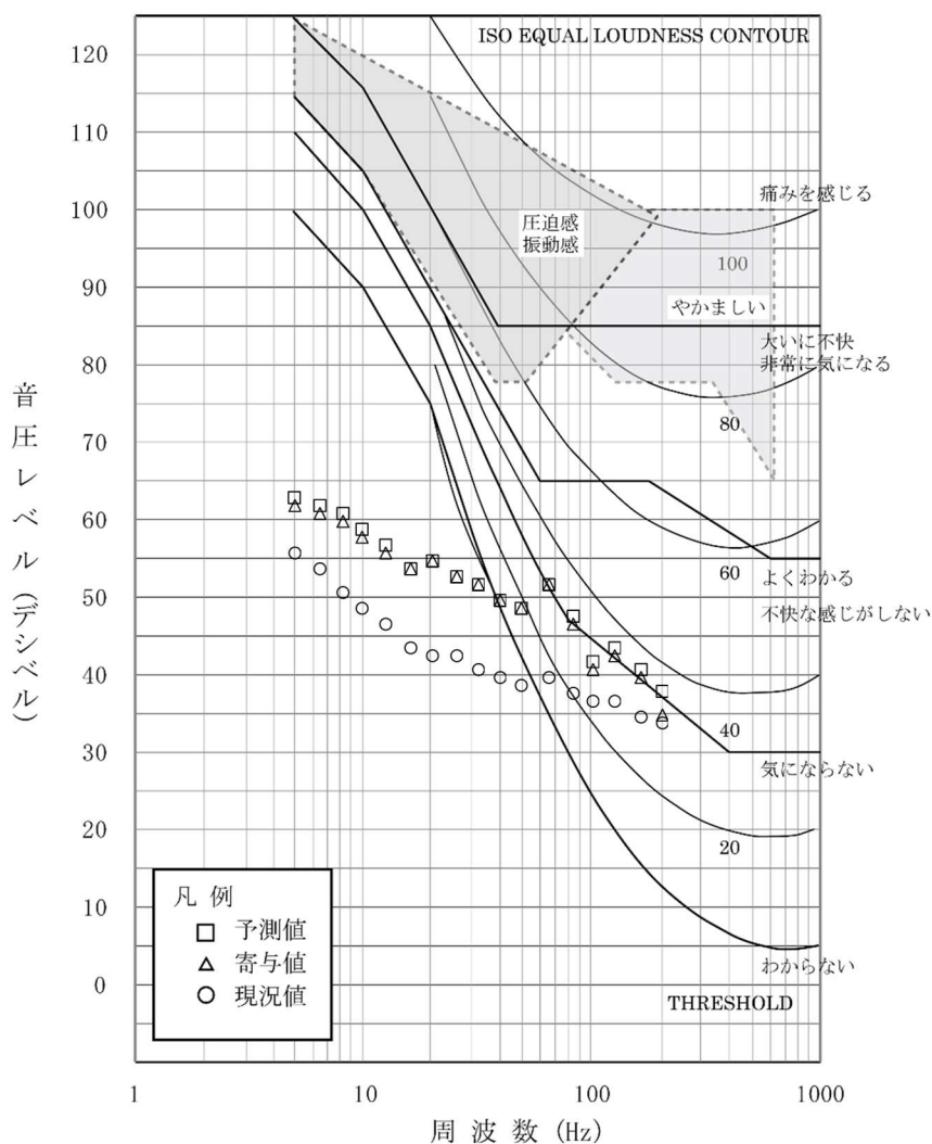
第 10.1.1-44 図(4) 圧迫感・振動感を感じる音圧レベルとの比較結果 (累積的な影響：環境 4 地点、冬季 1)
