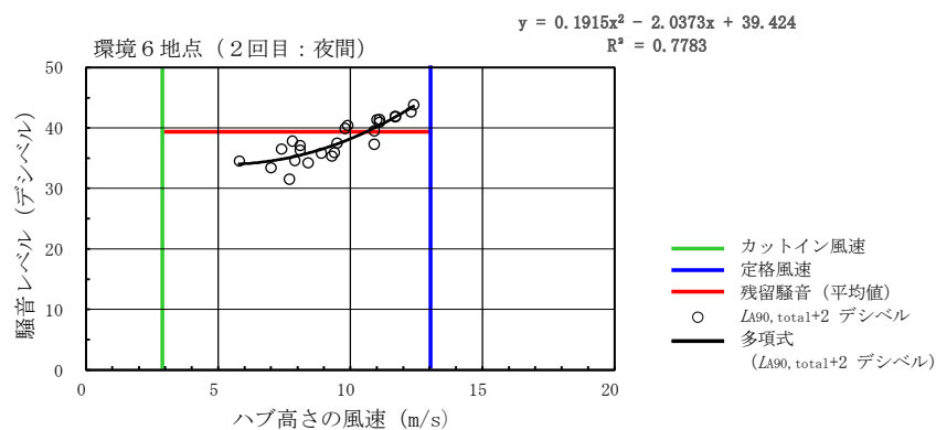
第 10.1.1-23 図(6) ハブ高さ風速と騒音レベル ( L_{A90} + 2 ) (2回目：環境6地点)
