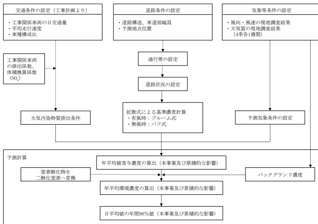
第10.1.1-7図 工事用資材等の搬出入に伴う二酸化窒素濃度の予測手順
