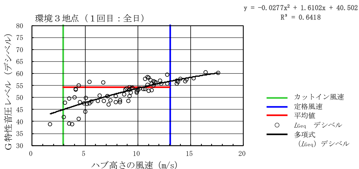
第 10. 1. 1-34 図(1) ハブ高さ風速と G 特性音圧レベル ( L_{Geq} ) (1 回目)
