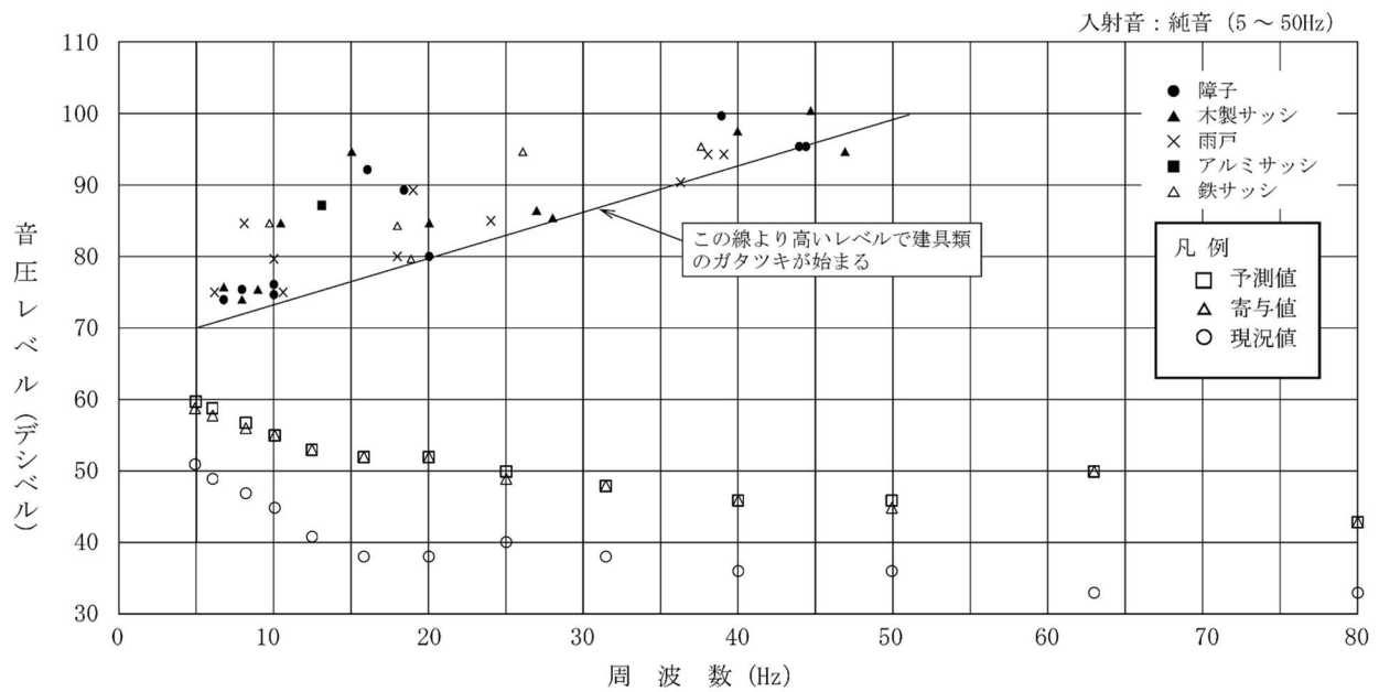
第 10.1.1-38 図 (3) 建具のがたつきが始まるレベルとの比較結果 (本事業：環境 3 地点、冬季 1)
