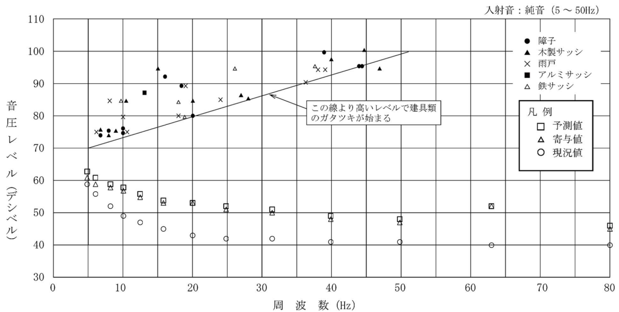
第 10.1.1-40 図(1) 建具のがたつきが始まるレベルとの比較結果 (本事業：環境 1 地点、冬季 2)
