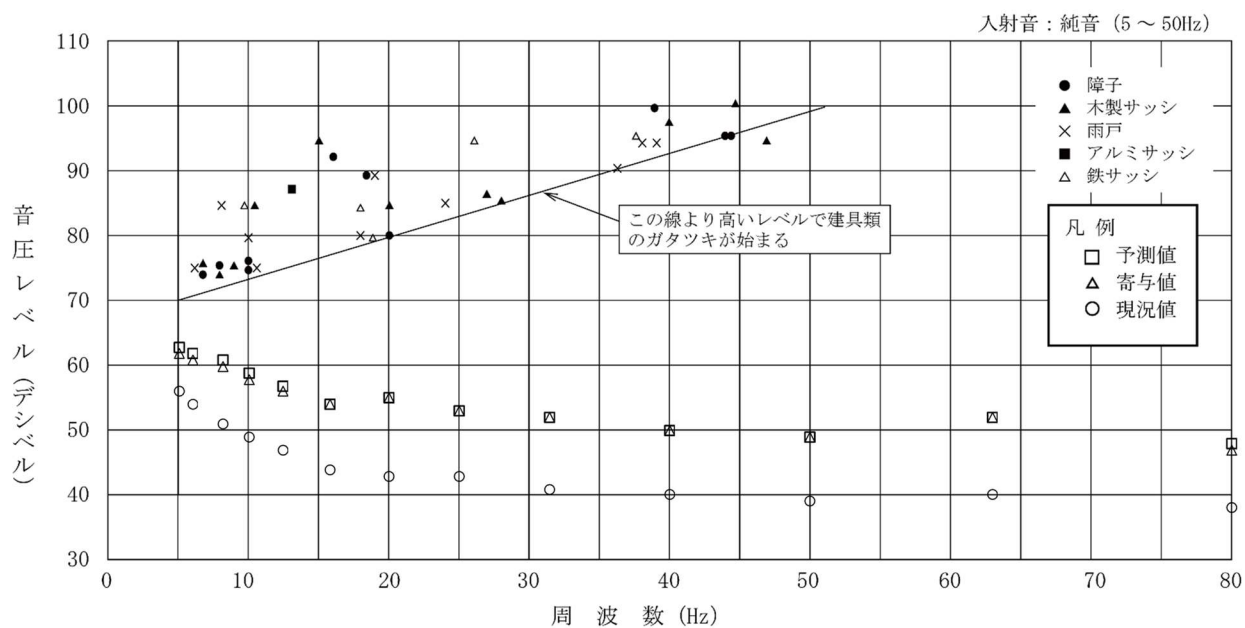
第 10.1.1-43 図(4) 建具のがたつきが始まるレベルとの比較結果 (累積的な影響：環境 4 地点、冬季 1)
