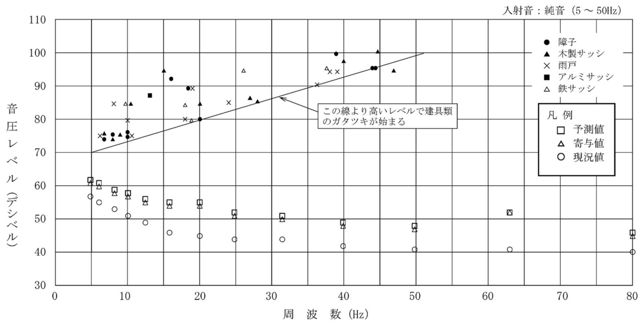
第 10.1.1-40 図(2) 建具のがたつきが始まるレベルとの比較結果 (本事業：環境2地点、冬季2)
