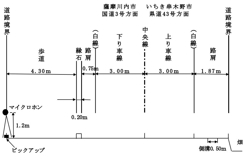
第 10. 1. 1-20 図 (2) 調査地点の道路断面構造等
