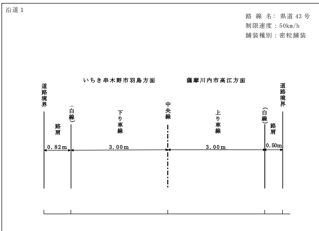
第 10.1.1-5 図(1) 道路構造
