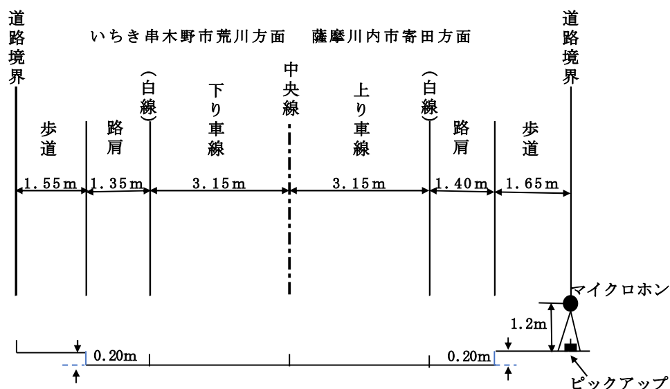
第 10. 1. 1-20 図 (1) 調査地点の道路断面構造等
