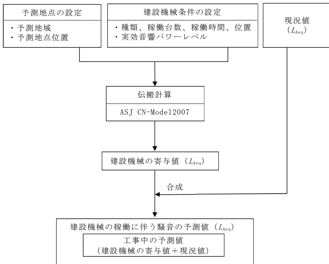
第10.1.1-27図 建設機械の稼働に伴う騒音の予測手順
