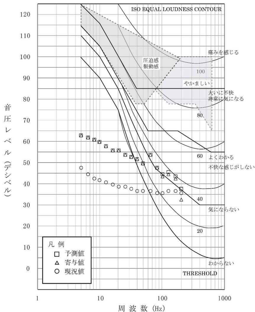
第 10.1.1-46 図(6) 圧迫感・振動感を感じる音圧レベルとの比較結果 (累積的な影響：環境 6 地点、冬季 2)
