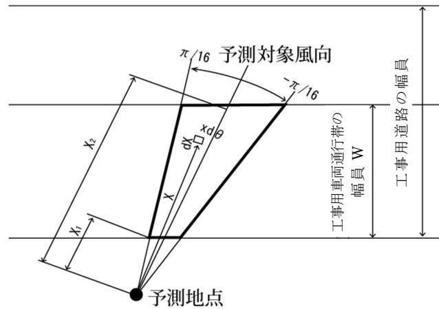
第10.1.1-10図 風向別の発生源の範囲と予測地点の距離の考え方
