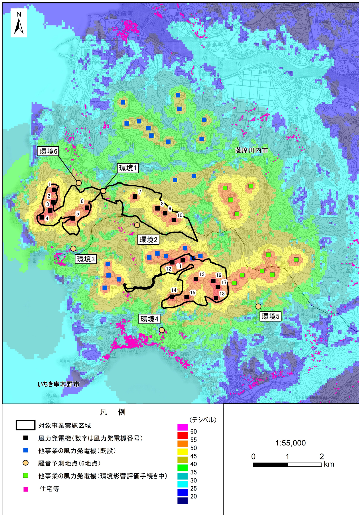
第 10.1.1-32 図(7) 風力発電機から発生する騒音の寄与の状況 (累積的な影響、冬季 2 昼間、環境 6 調査時)
