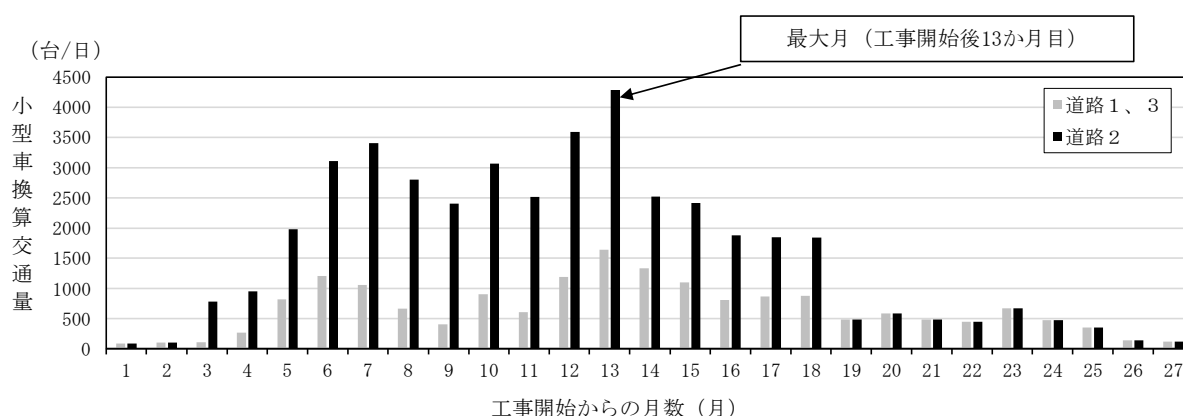
第 10.1.1-24 図 工事関係車両の小型車換算交通量
