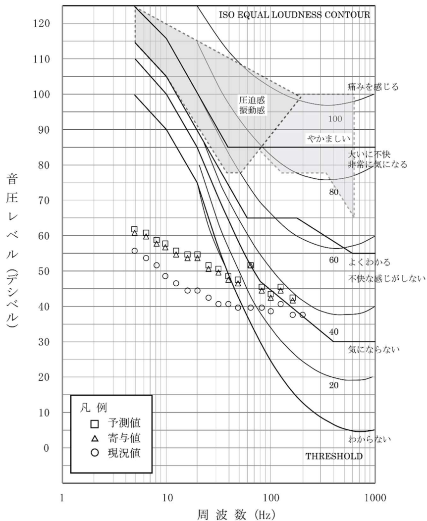
第 10.1.1-39 図(6) 圧迫感・振動感を感じる音圧レベルとの比較結果 (本事業：環境 6 地点、冬季 1)
