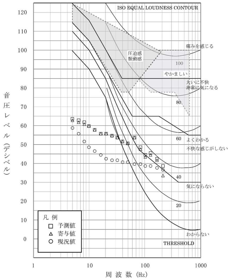
第 10.1.1-46 図(1) 圧迫感・振動感を感じる音圧レベルとの比較結果 (累積的な影響：環境地点1、冬季2)
