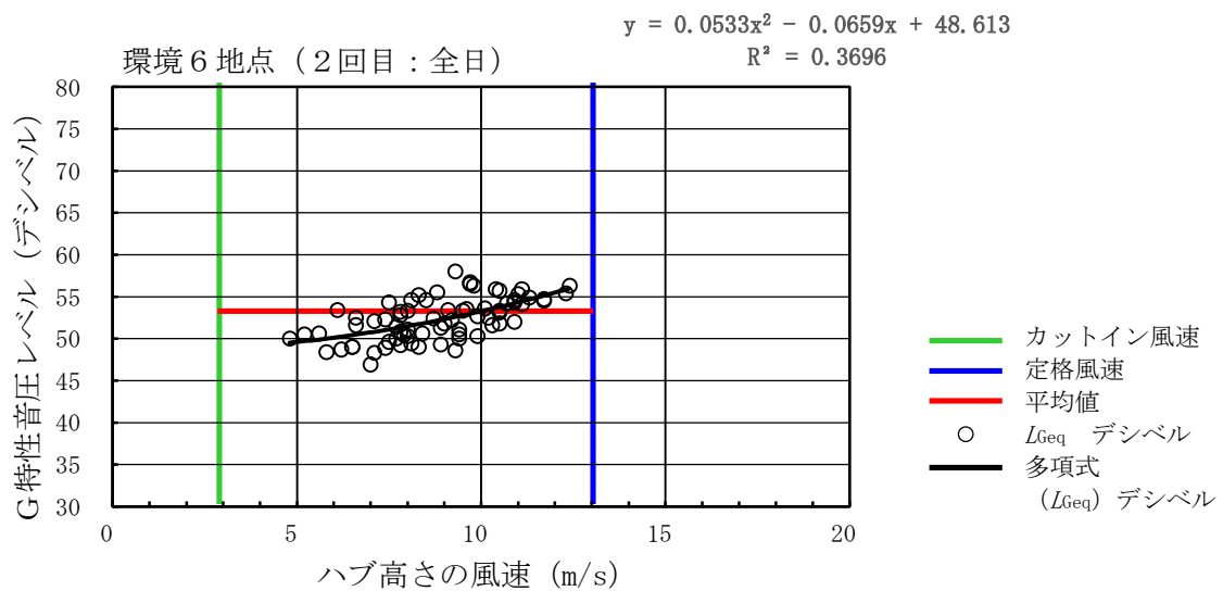
第 10. 1. 1-35 図(2) ハブ高さ風速と G 特性音圧レベル ( L_{Geq} ) (2 回目)
