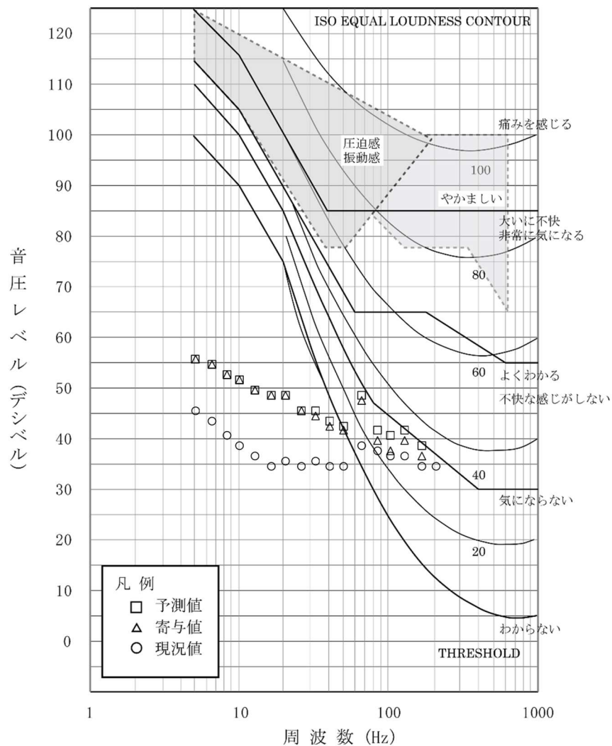
第 10. 1. 1-41 図(5) 圧迫感・振動感を感じる音圧レベルとの比較結果 (本事業：環境 5 地点、冬季 2)
