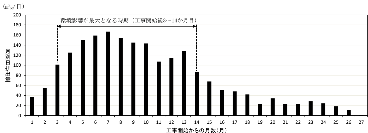
第 10. 1. 1-11 図 建設機械の稼働による窒素酸化物の月別排出量
