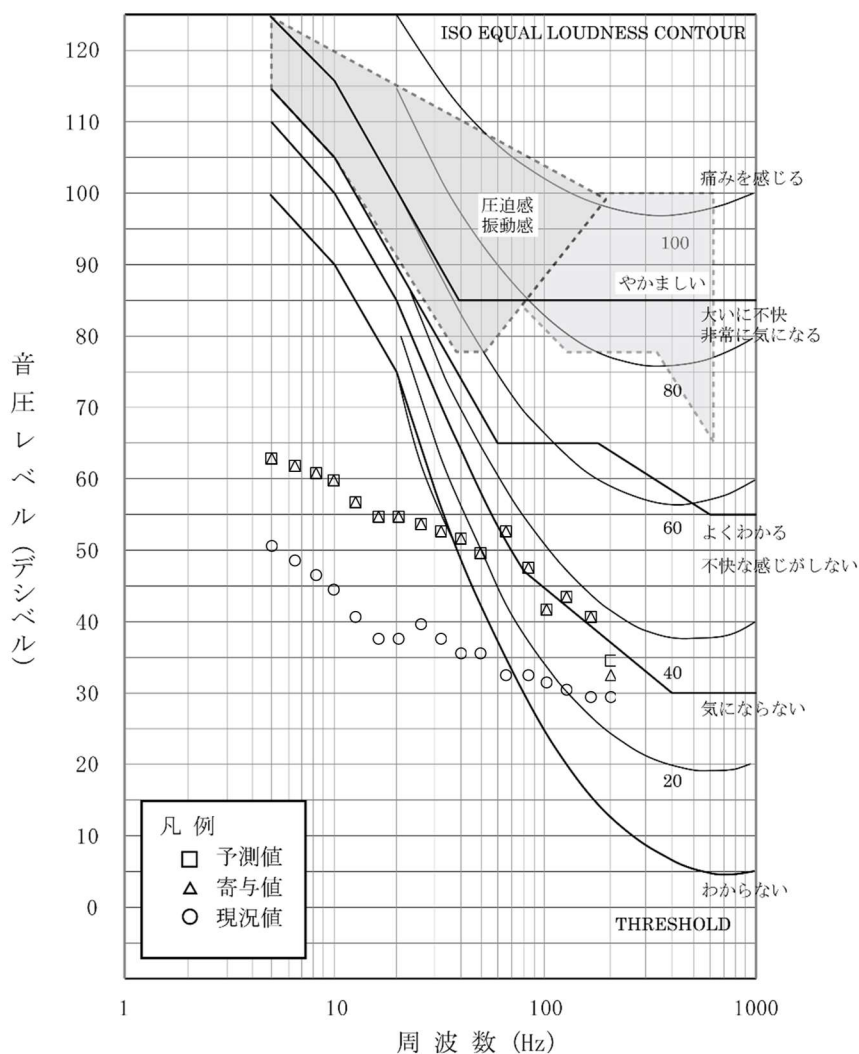
第 10.1.1-44 図 (3) 圧迫感・振動感を感じる音圧レベルとの比較結果 (累積的な影響：環境 3 地点、冬季 1)
