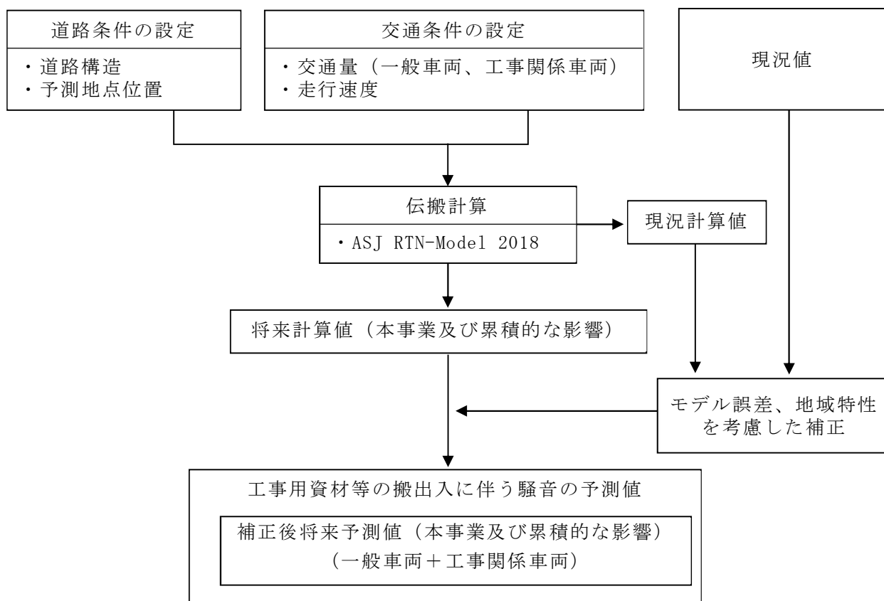
第10.1.1-25図 工事用資材等の搬出入に伴う騒音の予測手順
