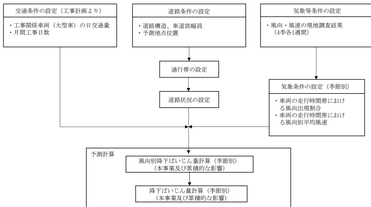
第 10.1.1-9 図 工事用資材等の搬出入に伴う粉じん等の予測手順
