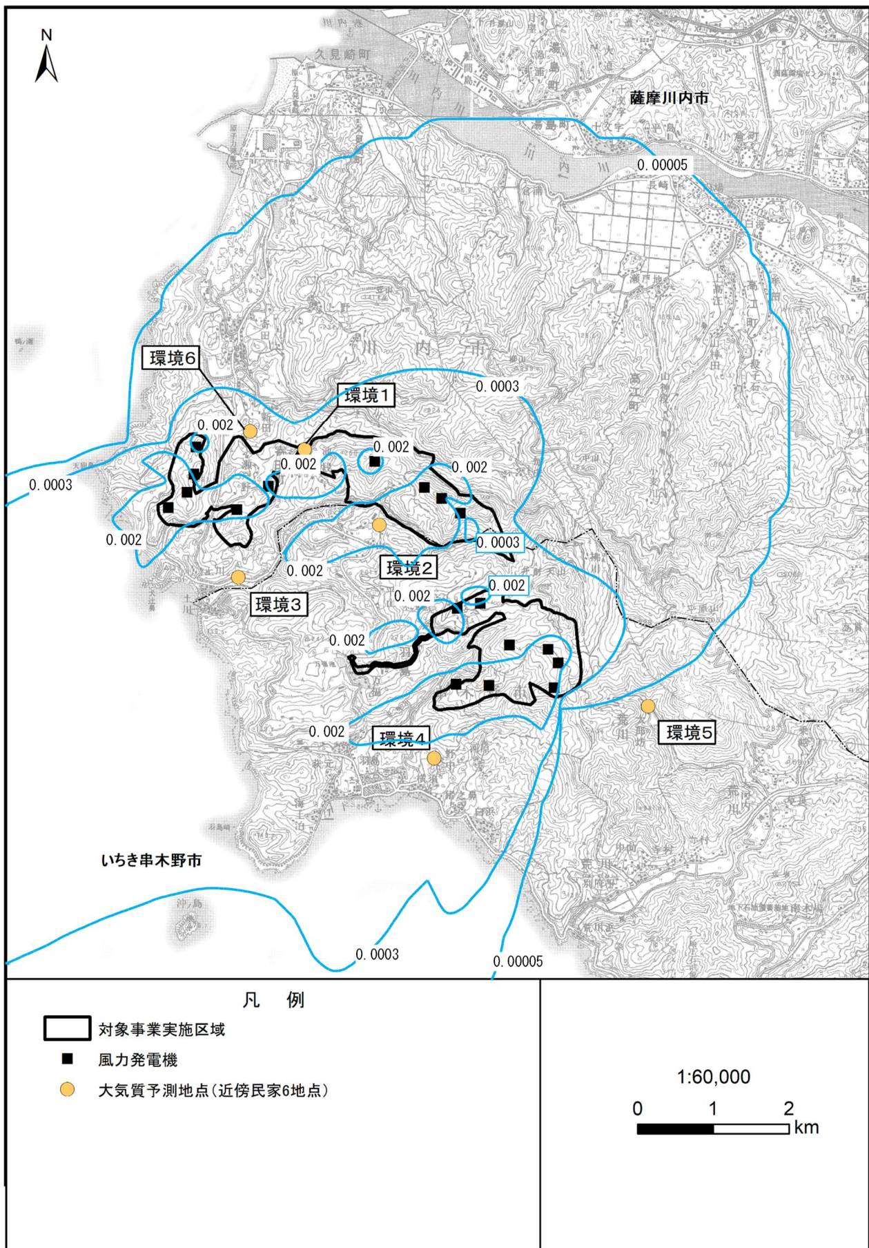
第 10.1.1-15 図(2) 建設機械の稼働に伴う二酸化窒素濃度の予測結果 (予測地点環境 2 が最大となった月：工事開始後 9 か月目、気象条件：夏季)
