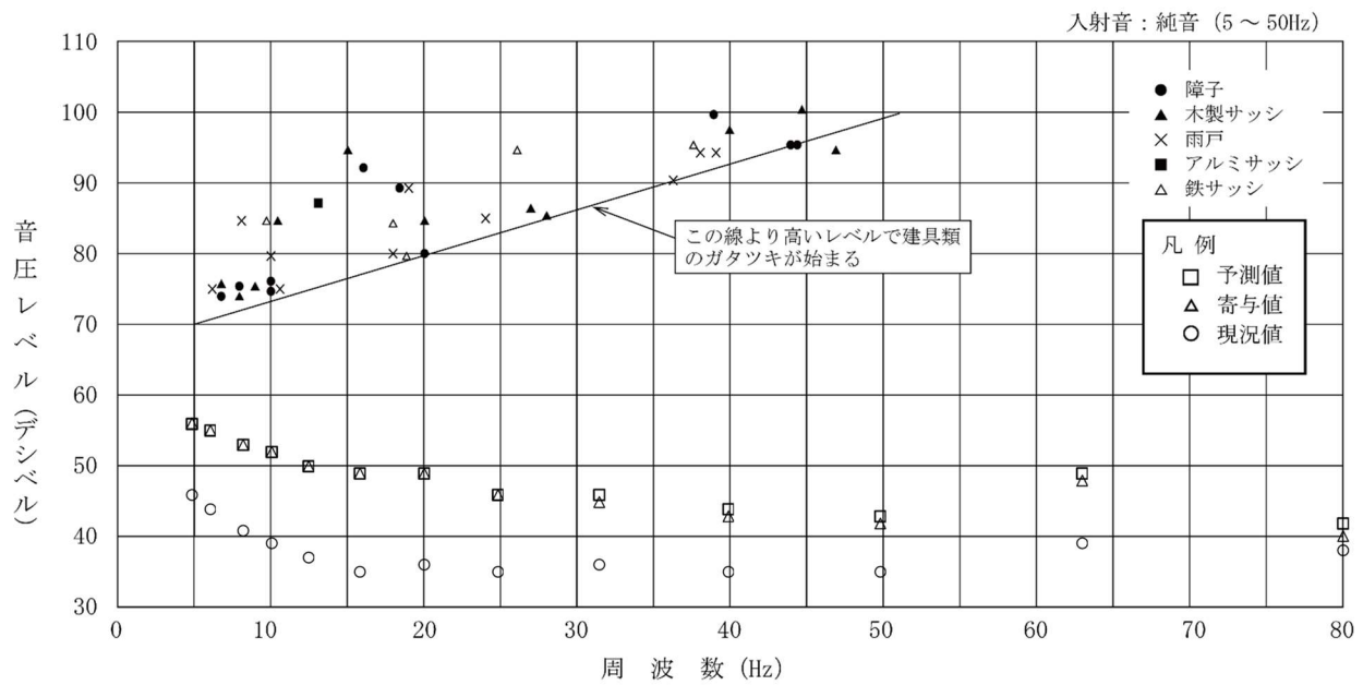
第 10. 1. 1-40 図(5) 建具のがたつきが始まるレベルとの比較結果 (本事業：環境 5 地点、冬季 2)
