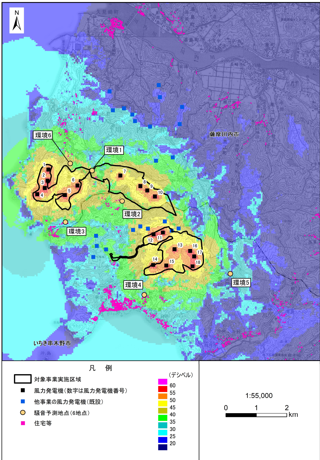
第 10.1.1-30 図(8) 風力発電機から発生する騒音の寄与の状況 (本事業、冬季2夜間、環境6 調査時)
