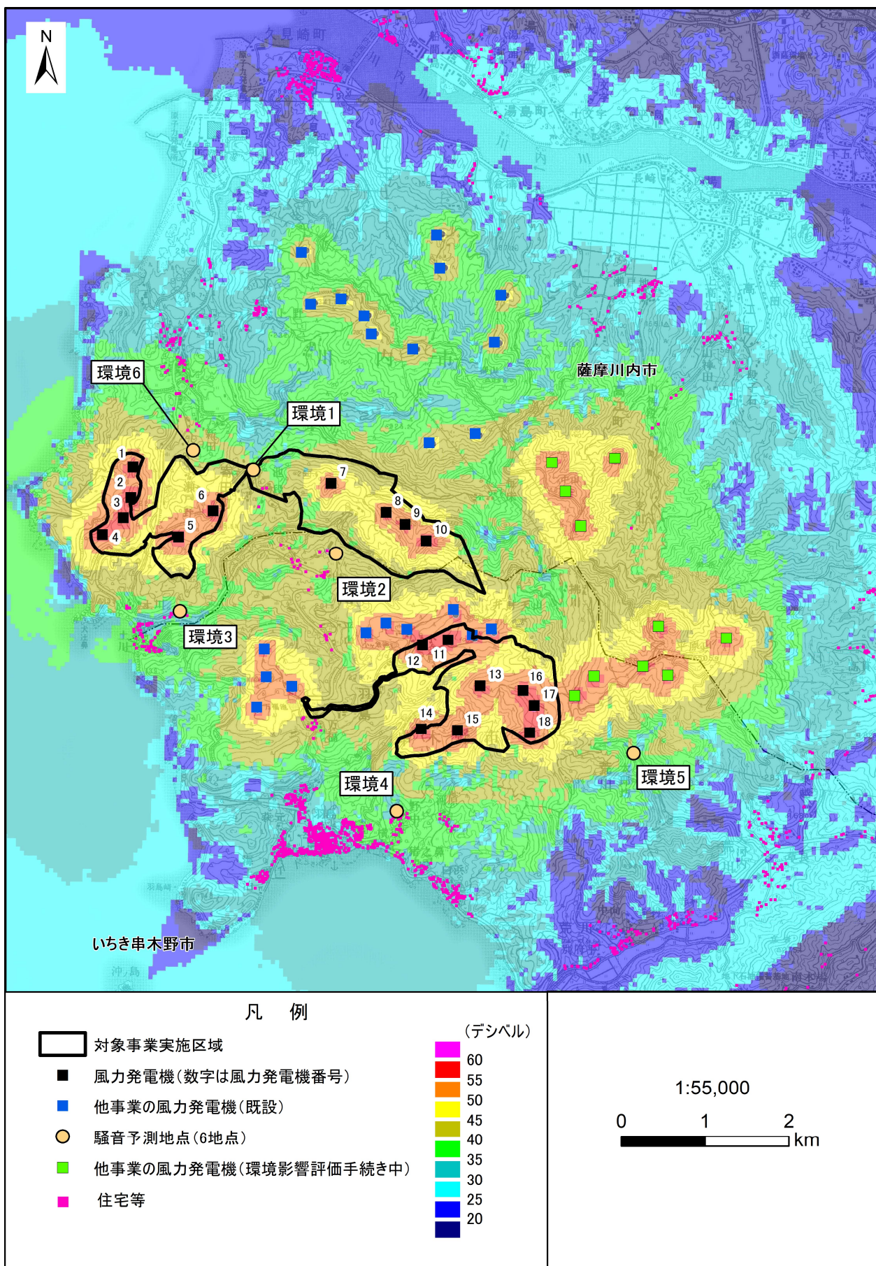
第 10.1.1-32 図(8) 風力発電機から発生する騒音の寄与の状況 (累積的な影響、冬季2夜間、環境6調査時)
