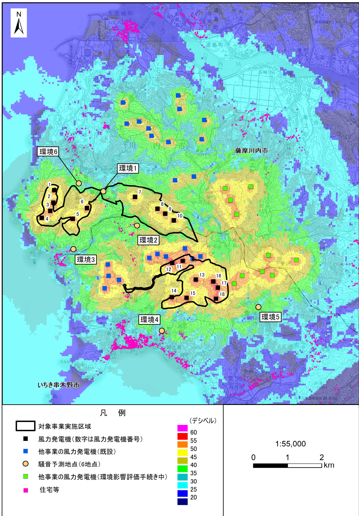
第 10.1.1-32 図(2) 風力発電機から発生する騒音の寄与の状況 (累積的な影響、冬季 1 夜間、環境 1 ～ 5 調査時)
