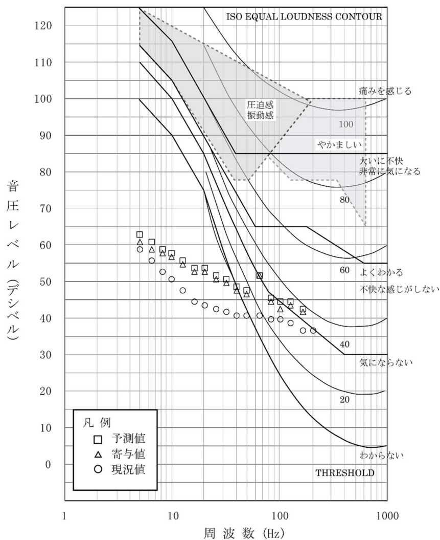
第 10.1.1-39 図(1) 圧迫感・振動感を感じる音圧レベルとの比較結果 (本事業：環境 1 地点、冬季 1)
