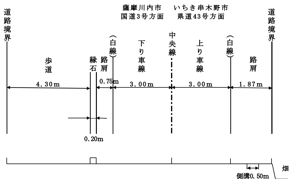
第 10.1.1-5 図(2) 道路構造
