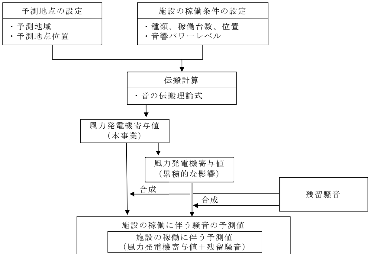
第10.1.1-28図 施設の稼働に伴う騒音の予測手順
