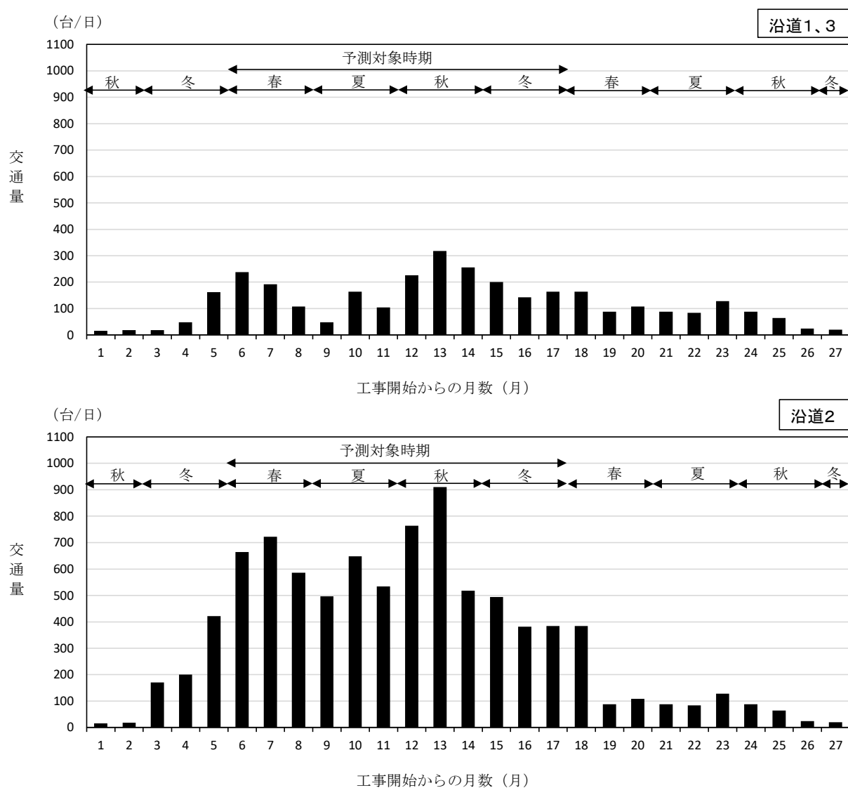
第10.1.1-8図 工事関係車両の月別日最大交通量
