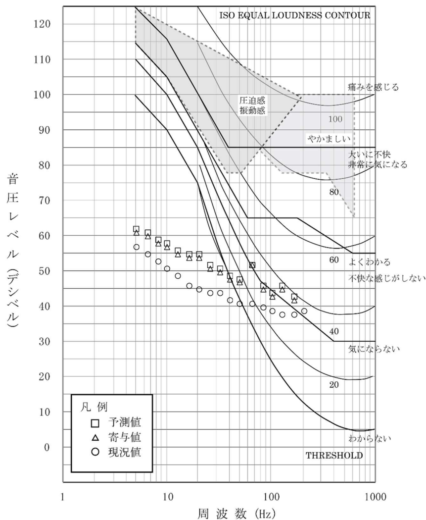
第 10.1.1-41 図(2) 圧迫感・振動感を感じる音圧レベルとの比較結果 (本事業：環境2地点、冬季2)
