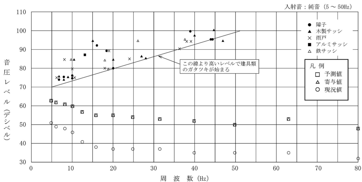
第 10.1.1-45 図 (3) 建具のがたつきが始まるレベルとの比較結果 (累積的な影響：環境 3 地点、冬季 2)
