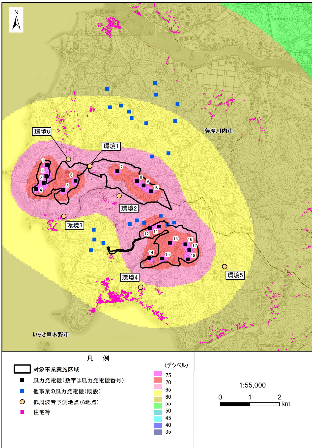
第 10.1.1-37 図 風力発電機から発生する G 特性音圧レベルの寄与値 (本事業)
