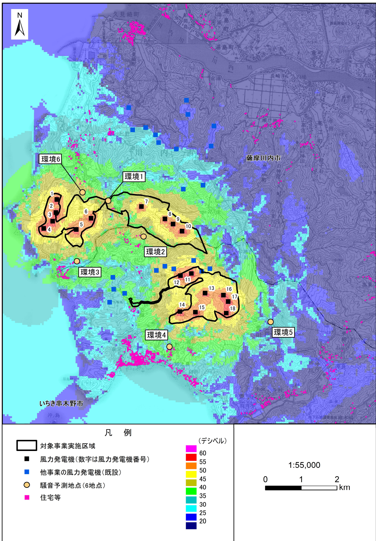
第 10.1.1-30 図(7) 風力発電機から発生する騒音の寄与の状況 (本事業、冬季2昼間、環境6 調査時)
