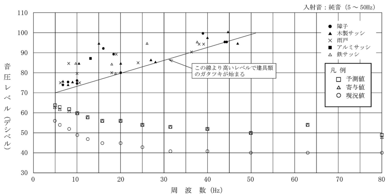
第 10.1.1-43 図(6) 建具のがたつきが始まるレベルとの比較結果 (累積的な影響：環境6地点、冬季1)
