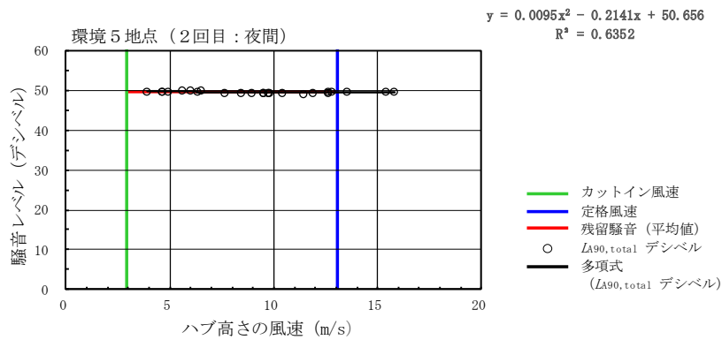
第 10.1.1-23 図(5) ハブ高さ風速と騒音レベル ( L_{A90} ) (2回目：環境5地点)
