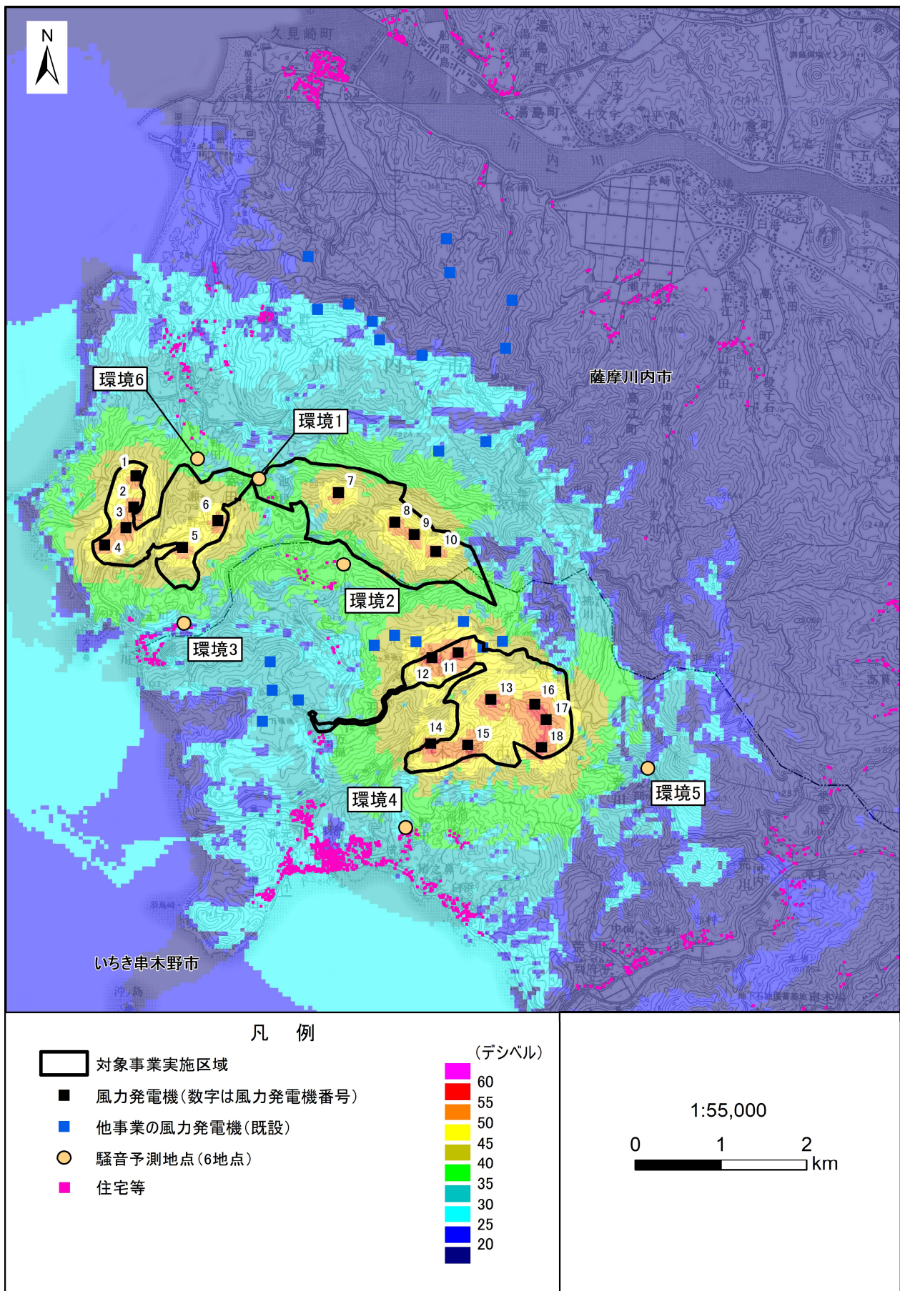
第 10.1.1-30 図(2) 風力発電機から発生する騒音の寄与の状況 (本事業、冬季1夜間、環境1～5 調査時)
