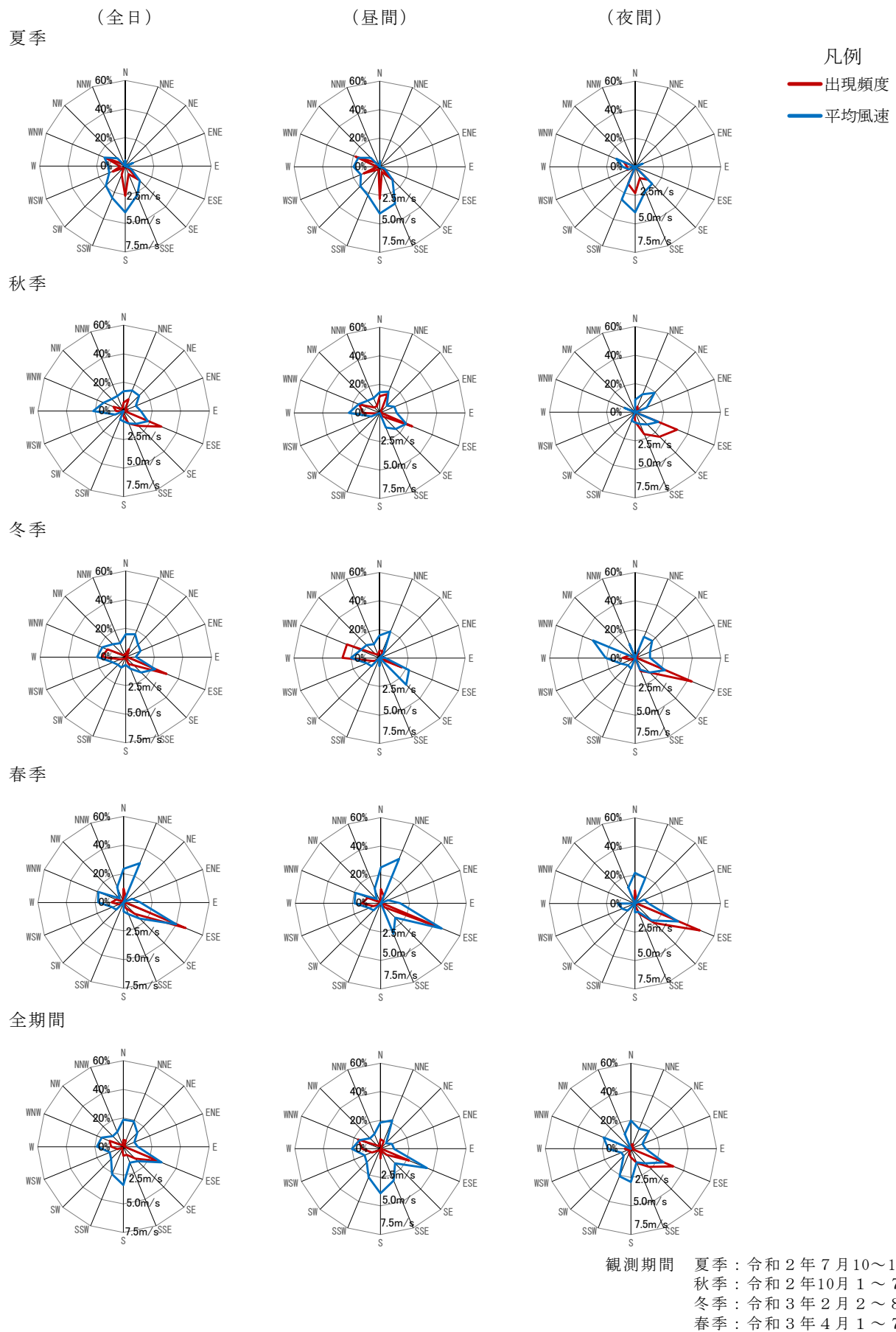
第 10.1.1-3 図(1) 風速階級別風配図 (沿道 1)
