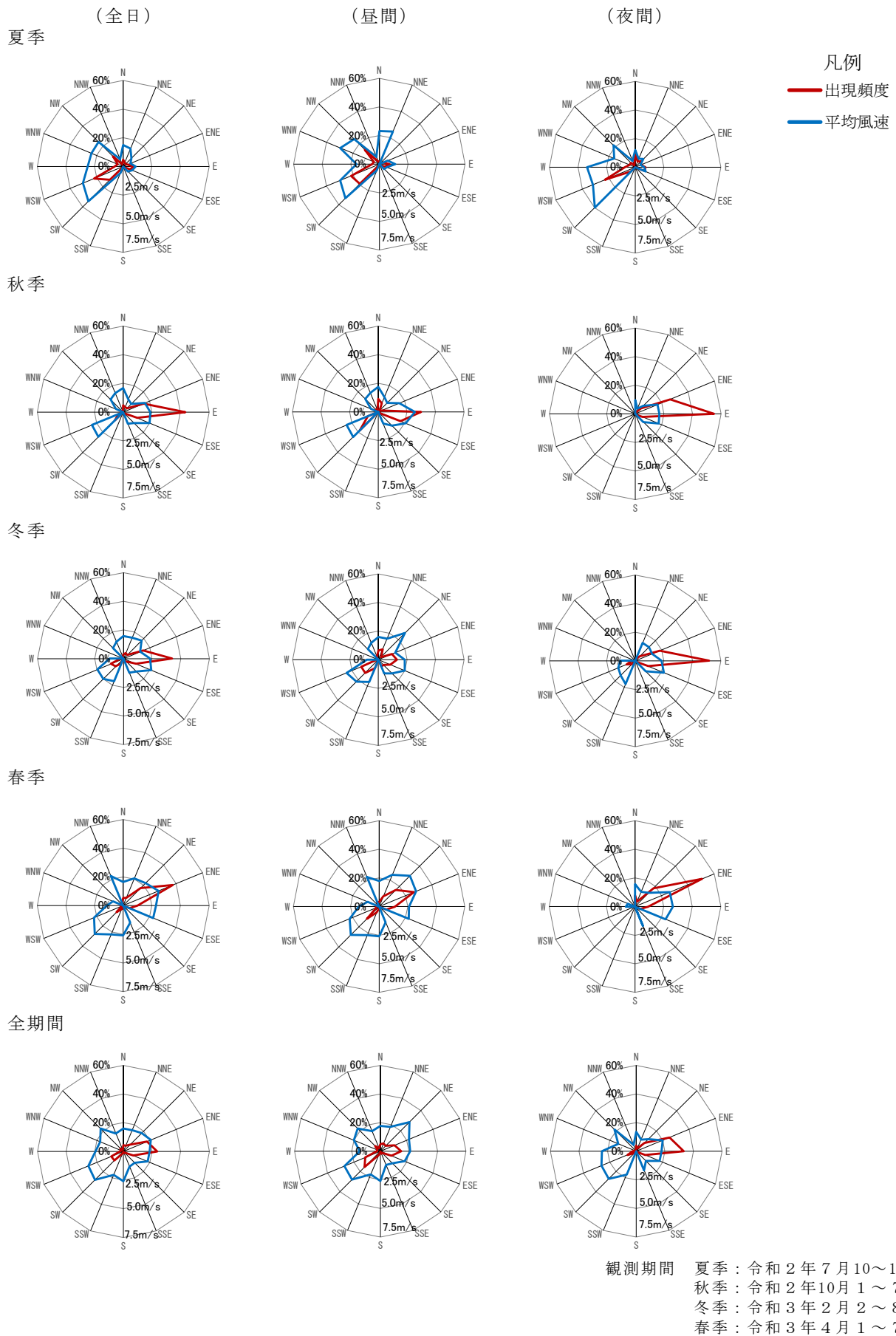
第 10.1.1-3 図(3) 風速階級別風配図 (沿道3)
