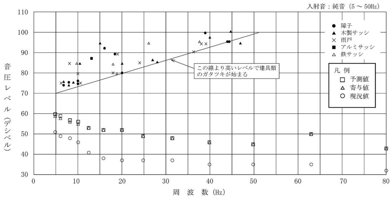
第 10. 1. 1-40 図 (3) 建具のがたつきが始まるレベルとの比較結果 （本事業：環境 3 地点、冬季 2）
