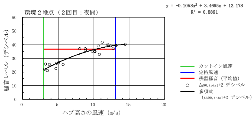
第 10. 1. 1-23 図(2) ハブ高さ風速と騒音レベル ( L_{A90}+2 ) (2 回目：環境2 地点)
