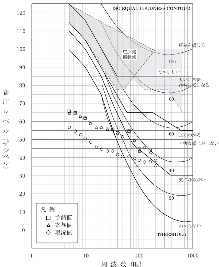
第 10.1.1-46 図(2) 圧迫感・振動感を感じる音圧レベルとの比較結果 (累積的な影響：環境2地点、冬季2)
