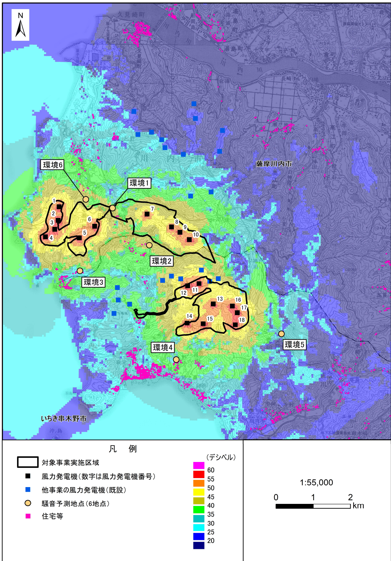
第 10.1.1-30 図(5) 風力発電機から発生する騒音の寄与の状況 (本事業、冬季 1 昼間、環境 6 調査時)
