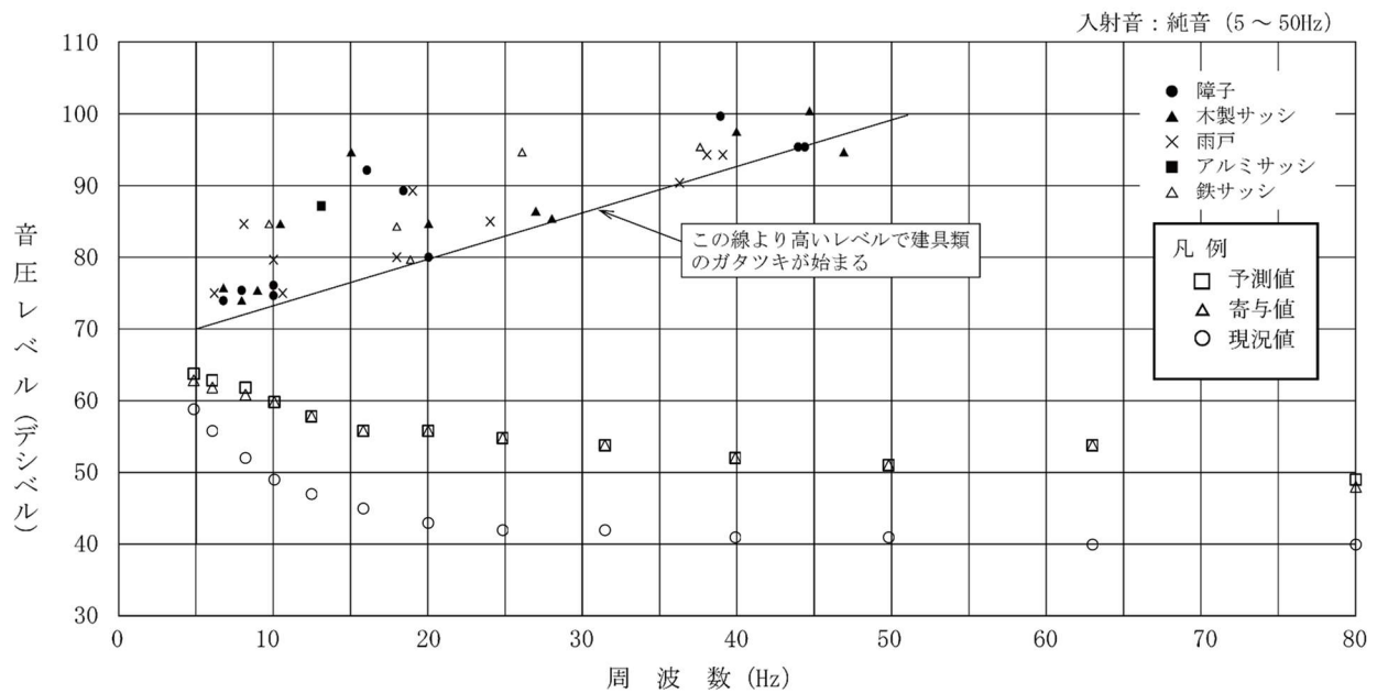
第 10.1.1-45 図(1) 建具のがたつきが始まるレベルとの比較結果 (累積的な影響：環境1地点、冬季2)
