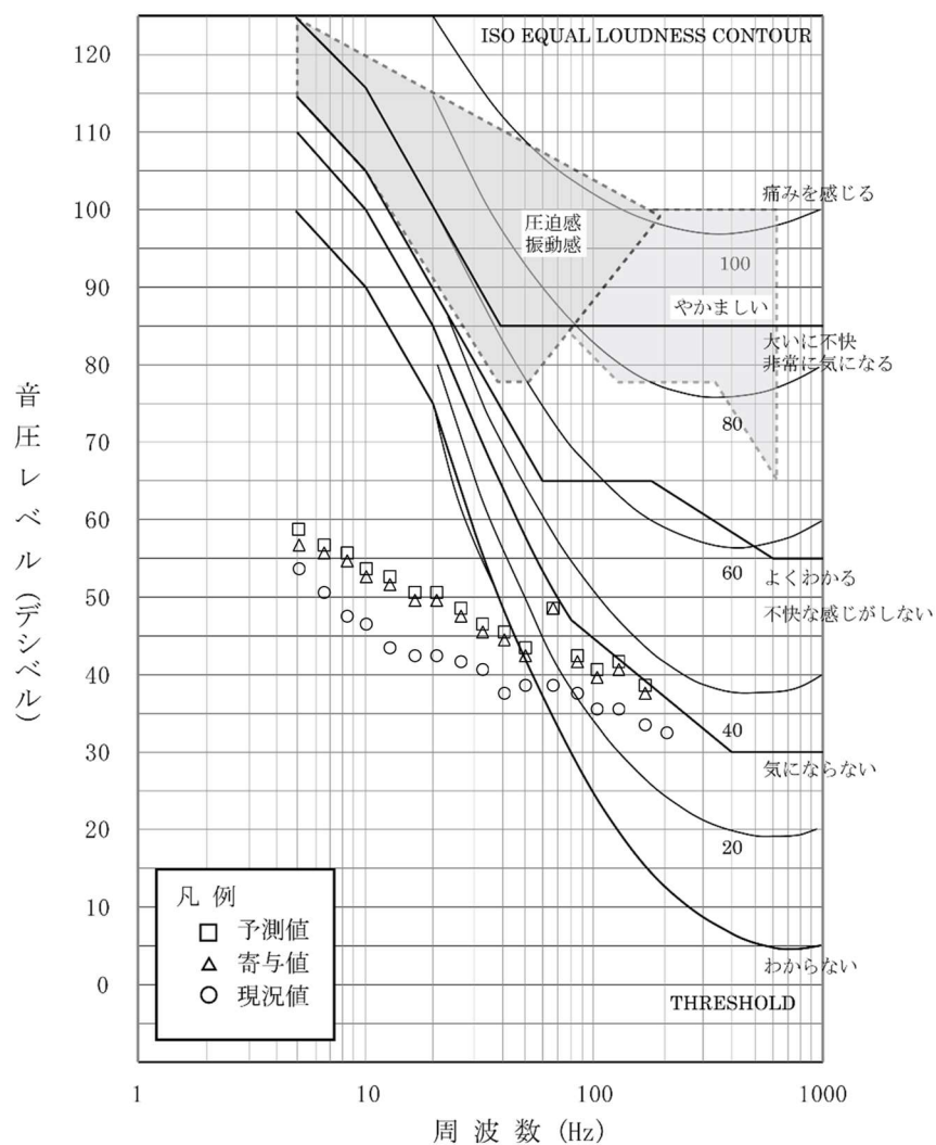
第 10.1.1-41 図(4) 圧迫感・振動感を感じる音圧レベルとの比較結果 (本事業：環境4地点、冬季2)
