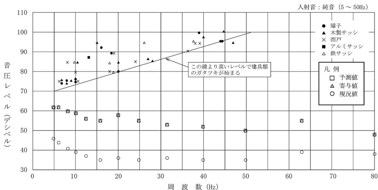
第 10.1.1-45 図(5) 建具のがたつきが始まるレベルとの比較結果 (累積的な影響：環境5地点、冬季2)
