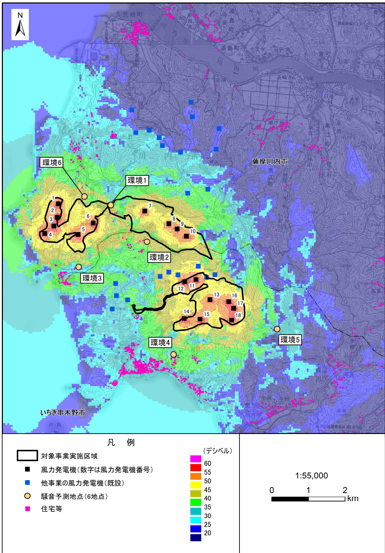
第 10.1.1-30 図(6) 風力発電機から発生する騒音の寄与の状況 (本事業、冬季1夜間、環境6 調査時)
