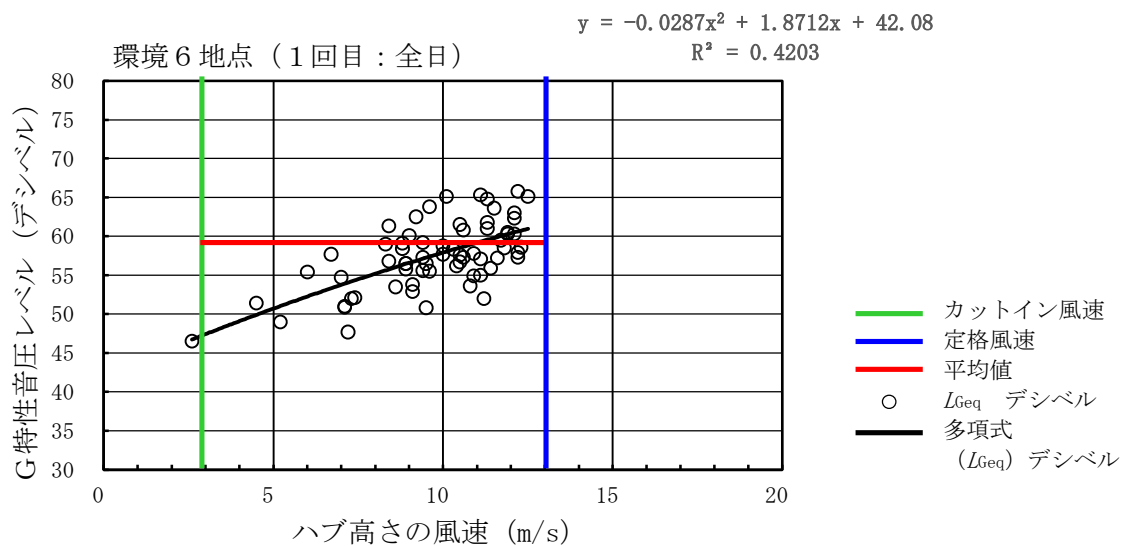
第 10.1.1-34 図(2) ハブ高さ風速と G 特性音圧レベル ( L_{Geq} ) (1 回目)
