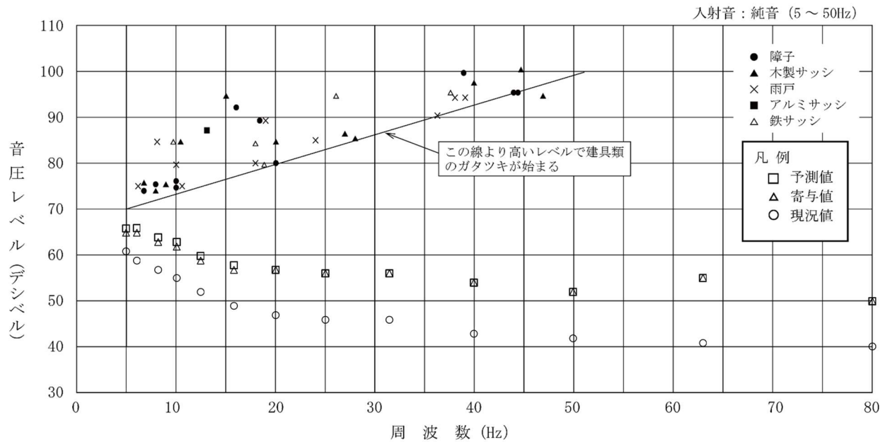
第 10. 1. 1-43 図 (2) 建具のがたつきが始まるレベルとの比較結果 (累積的な影響：環境 2 地点、冬季 1)
