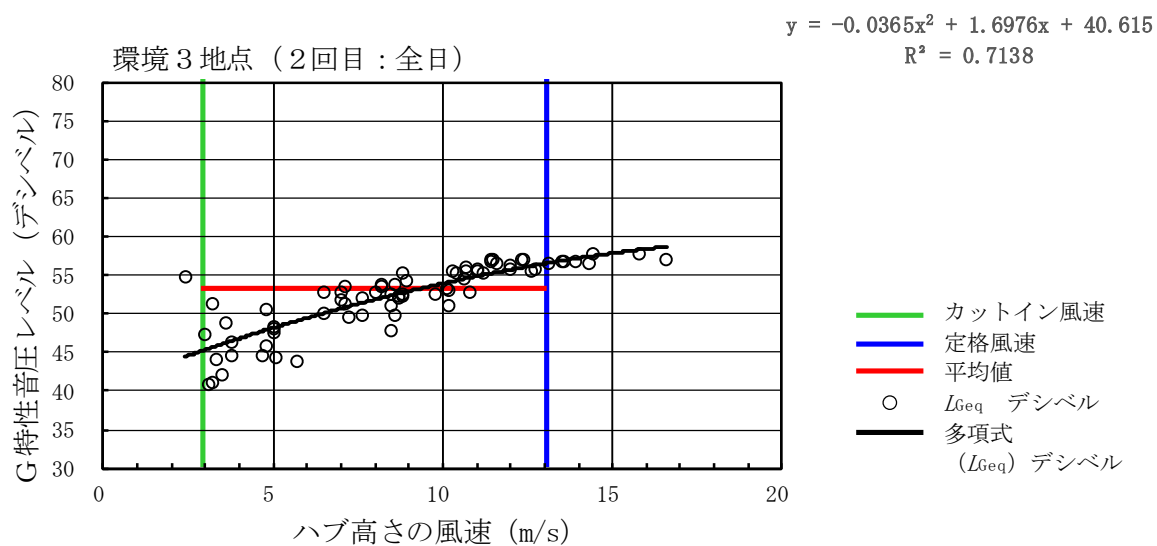
第 10. 1. 1-35 図(1) ハブ高さ風速と G 特性音圧レベル ( L_{Geq} ) (2 回目)
