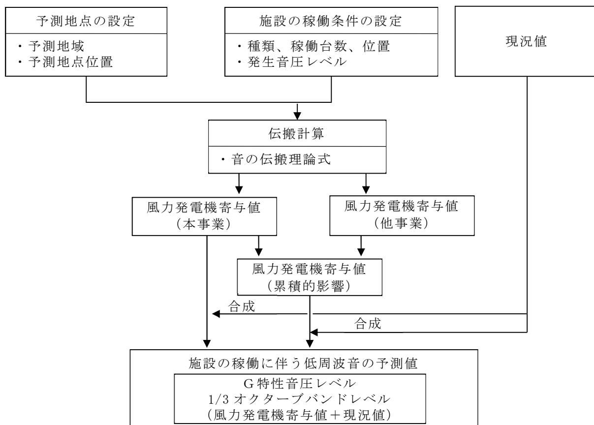
第 10.1.1-36 図 施設の稼働に伴う低周波音の予測手順
