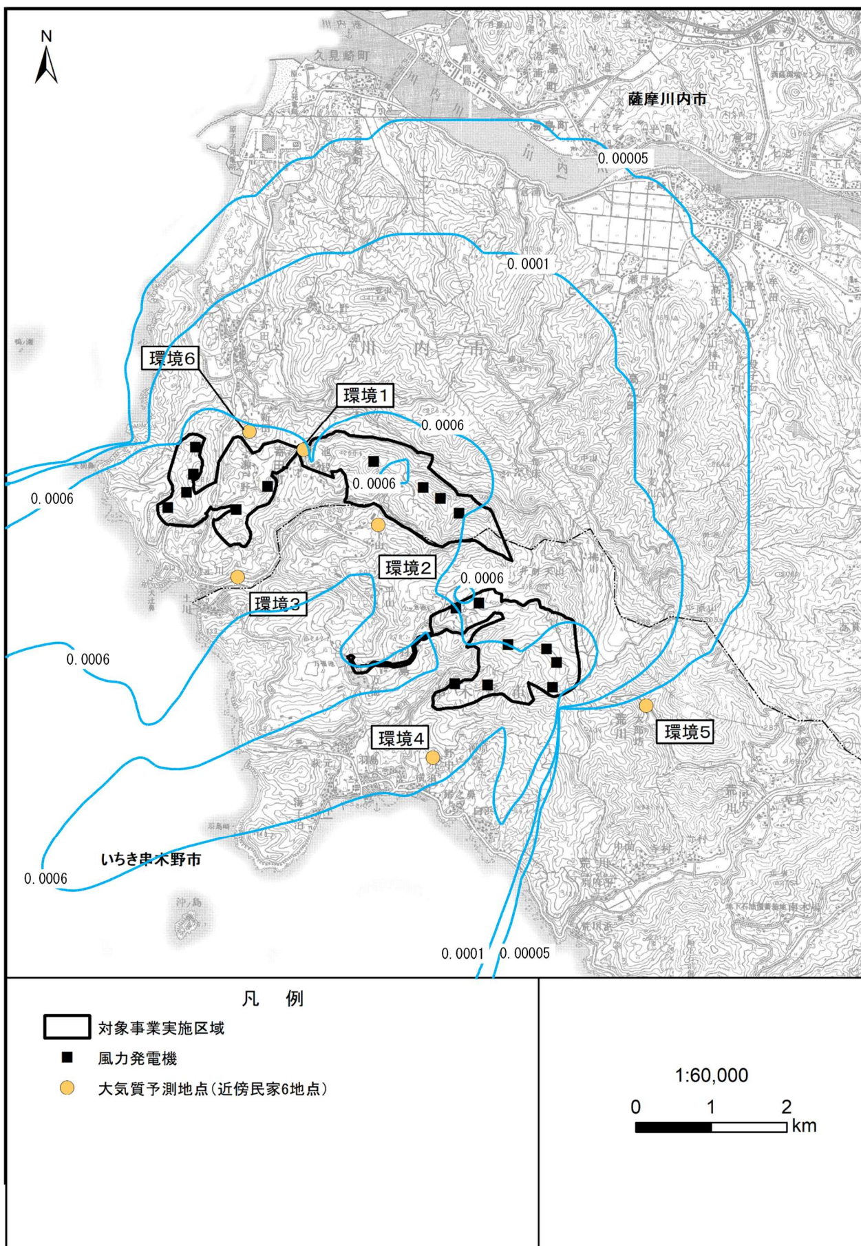
第 10.1.1-15 図(6) 建設機械の稼働に伴う二酸化窒素濃度の予測結果 (予測地点環境 6 が最大となった月：工事開始後 10 か月目、気象条件：夏季)
