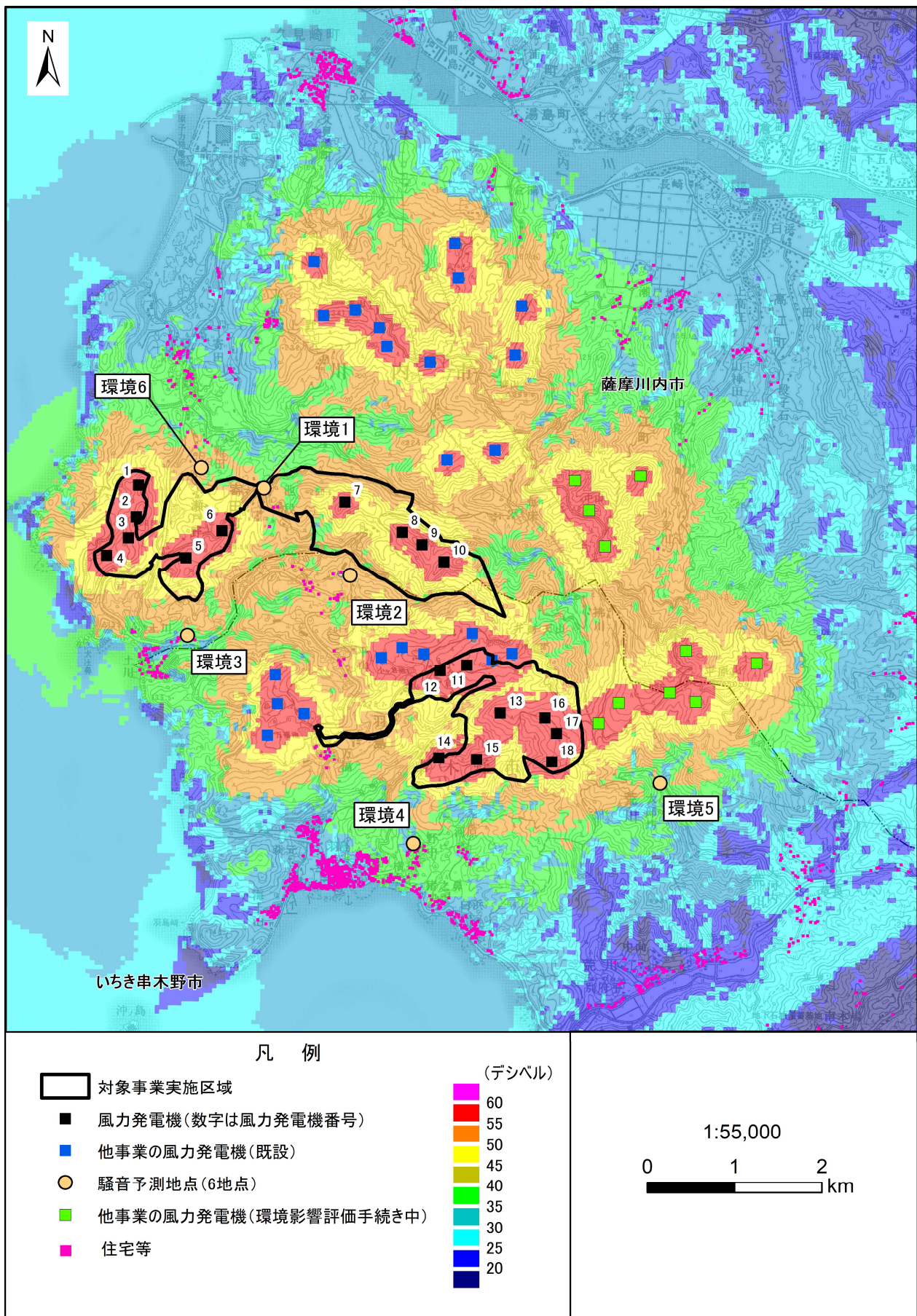
第 10.1.1-32 図(5) 風力発電機から発生する騒音の寄与の状況 (累積的な影響、冬季 1 昼間、環境 6 調査時)
