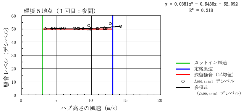
第 10.1.1-22 図(5) ハブ高さ風速と騒音レベル ( L_{A90} ) (1回目：環境5地点)
