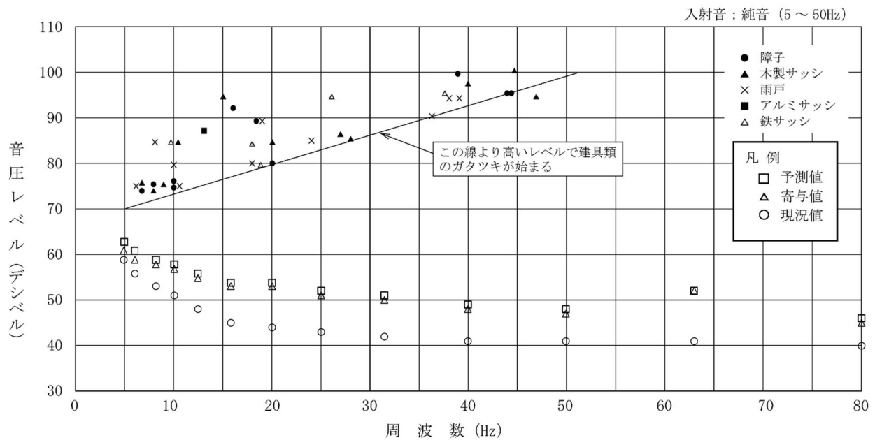
第 10.1.1-38 図(1) 建具のがたつきが始まるレベルとの比較結果 (本事業：環境 1 地点、冬季 1)
