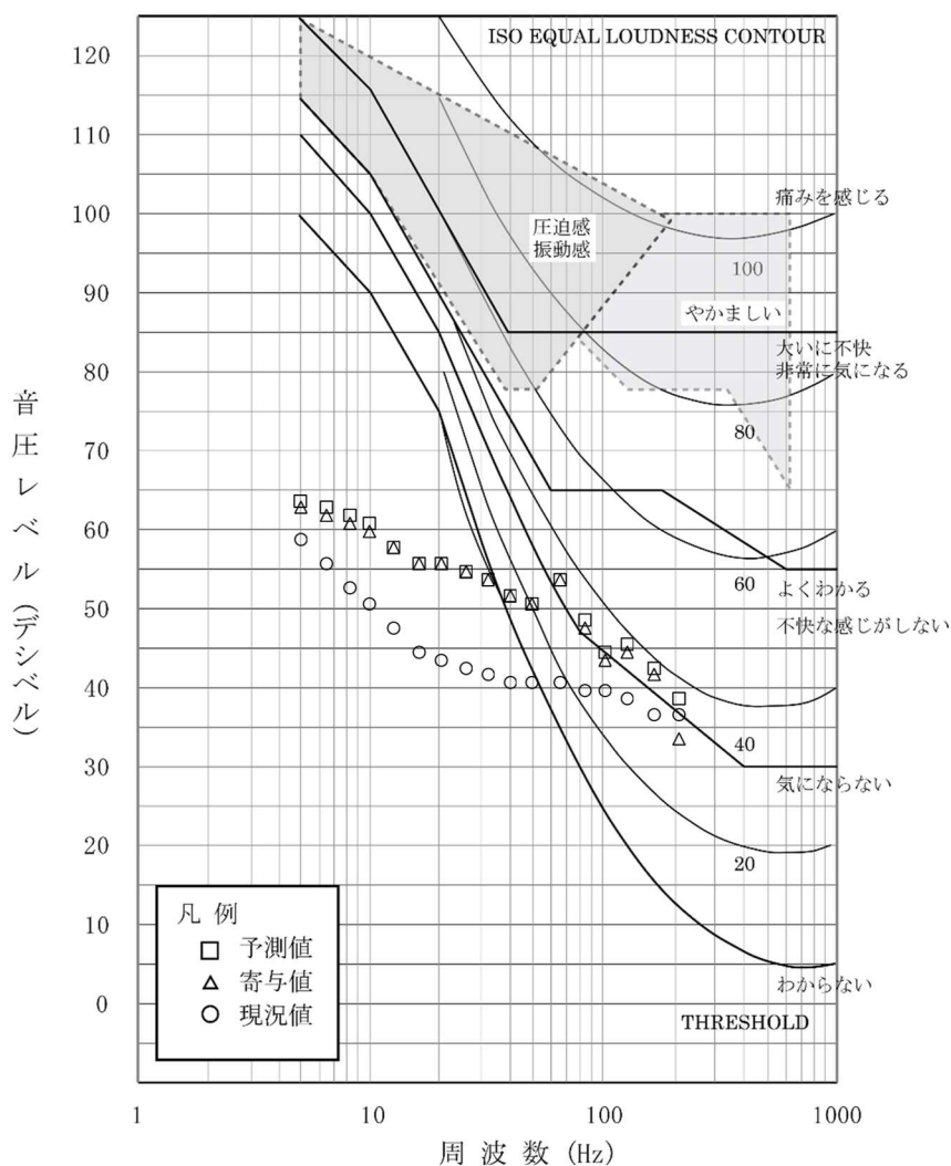
第 10.1.1-44 図(6) 圧迫感・振動感を感じる音圧レベルとの比較結果 (累積的な影響：環境6地点、冬季1)
