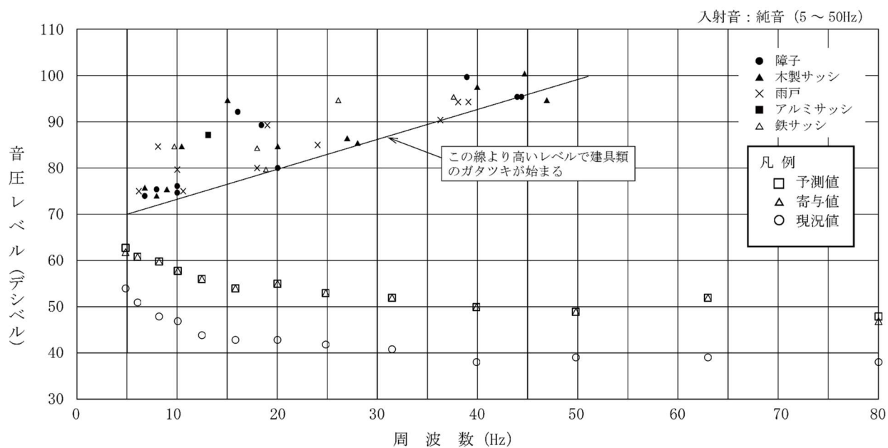
第 10.1.1-45 図(4) 建具のがたつきが始まるレベルとの比較結果 (累積的な影響：環境4地点、冬季2)
