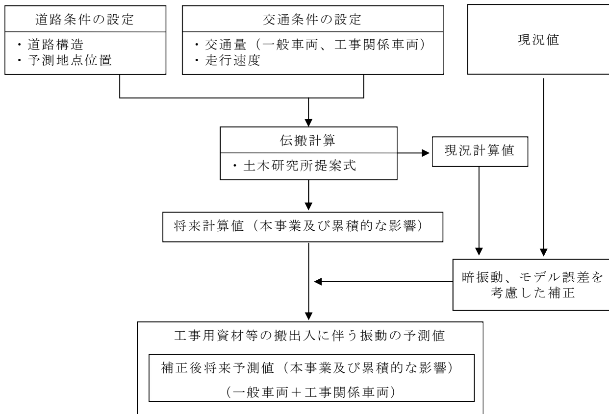
第10.1.1-48図 工事用資材等の搬出入に伴う振動の予測手順
