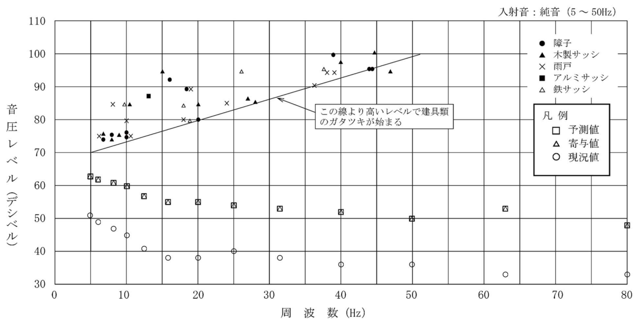
第 10.1.1-43 図 (3) 建具のがたつきが始まるレベルとの比較結果 (累積的な影響：環境 3 地点、冬季 1)
