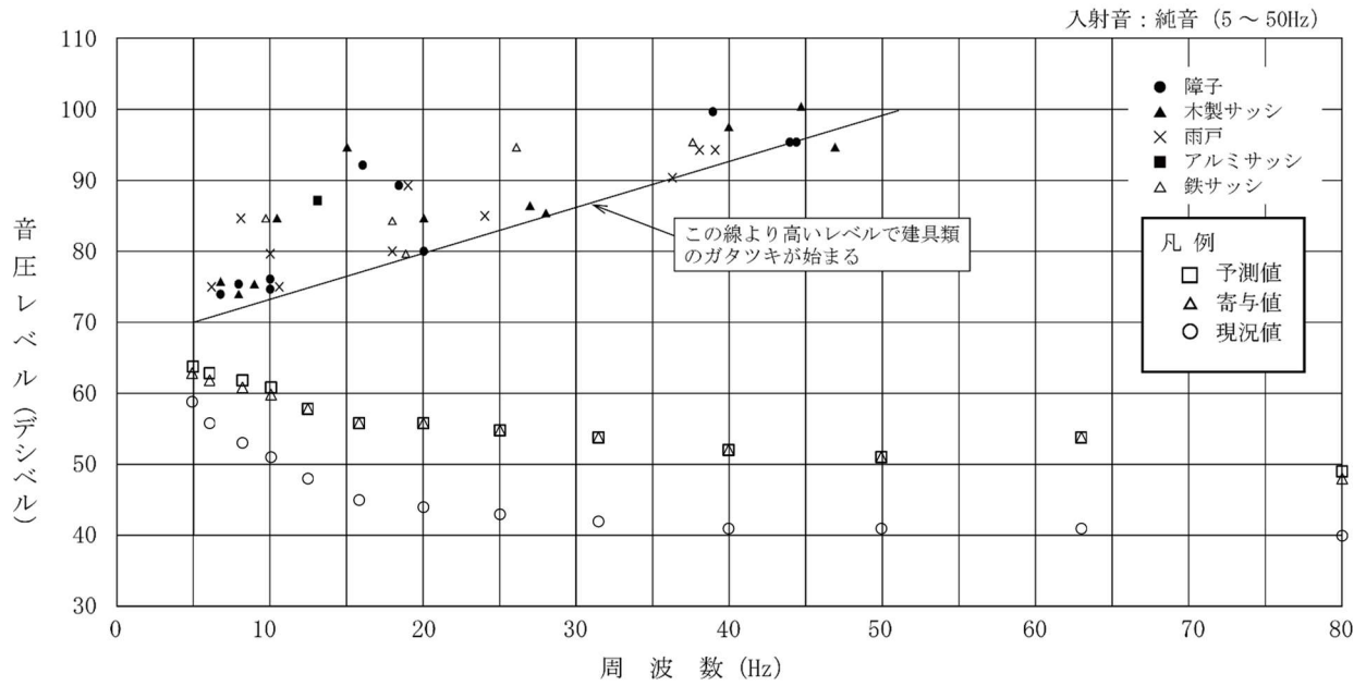
第 10.1.1-43 図(1) 建具のがたつきが始まるレベルとの比較結果 （累積的な影響：環境 1 地点、冬季 1）
