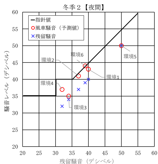
10.1.1-31 図 残留騒音、風車騒音（予測値）、指針値の関係（本事業）
