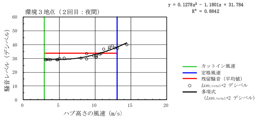
第 10.1.1-23 図(3) ハブ高さ風速と騒音レベル ( L_{A90}+2 ) (2回目：環境3地点)
