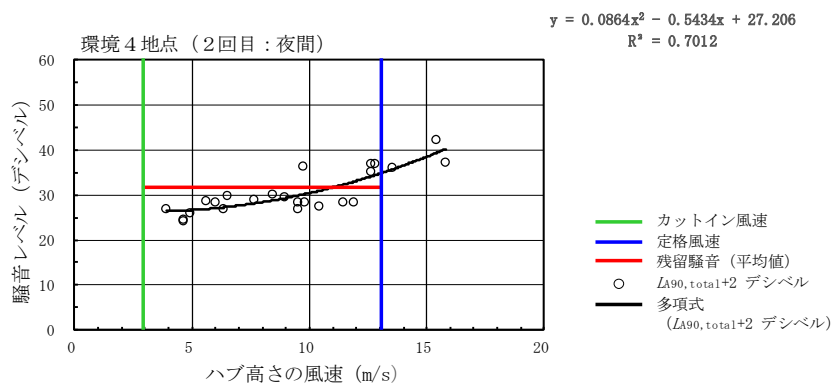
第 10.1.1-23 図(4) ハブ高さ風速と騒音レベル ( L_{A90}+2 ) (2回目：環境4地点)
