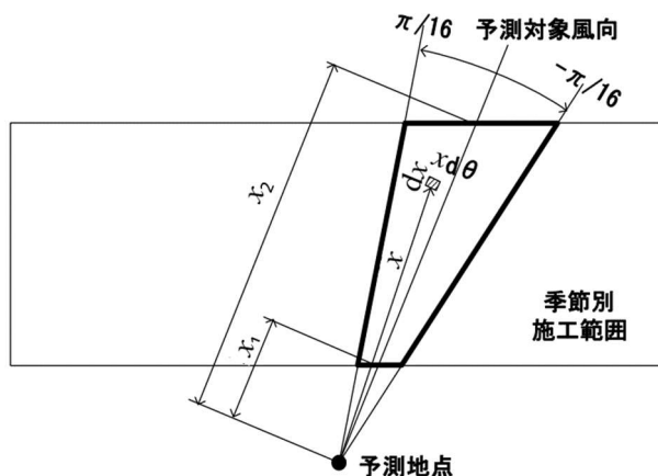
第 10.1.1-18 図 風向別の発生源の範囲と予測地点の距離の考え方
