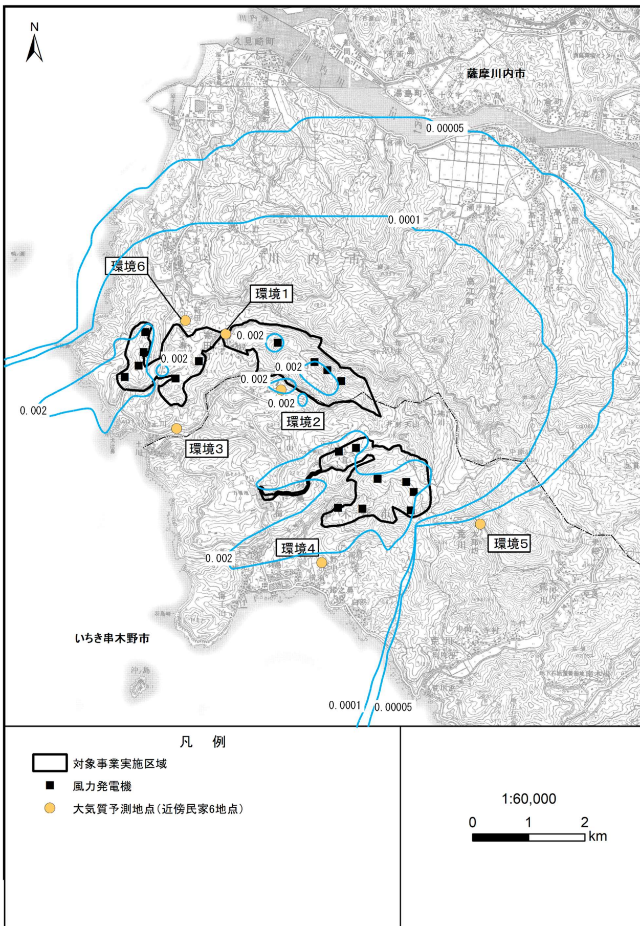
第 10.1.1-15 図(4) 建設機械の稼働に伴う二酸化窒素濃度の予測結果 (予測地点環境 4 が最大となった月：工事開始後 6 か月目、気象条件：夏季)
