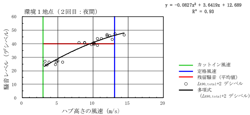
第 10. 1. 1-23 図(1) ハブ高さ風速と騒音レベル ( L_{A90}+2 ) (2 回目：環境1 地点)
