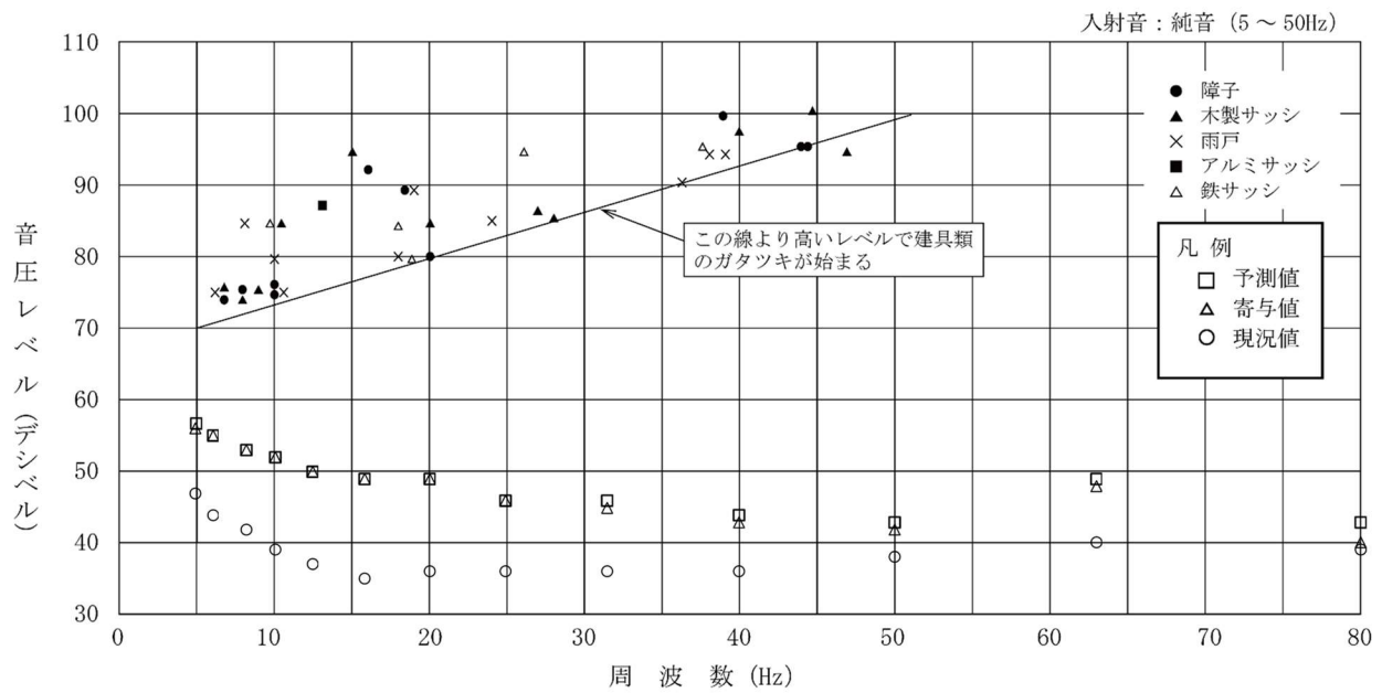
第 10.1.1-38 図(5) 建具のがたつきが始まるレベルとの比較結果 (本事業：環境 5 地点、冬季 1)
