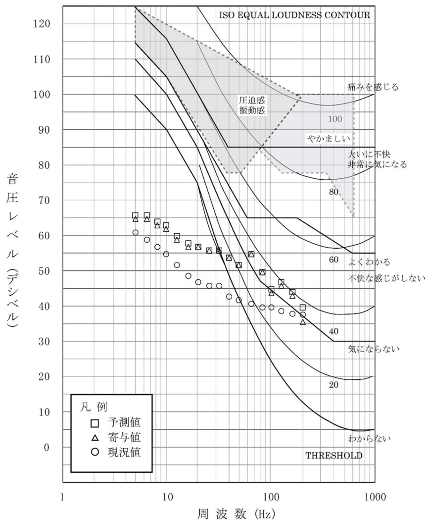
第 10. 1. 1-44 図 (2) 圧迫感・振動感を感じる音圧レベルとの比較結果 (累積的な影響：環境 2 地点、冬季 1)
