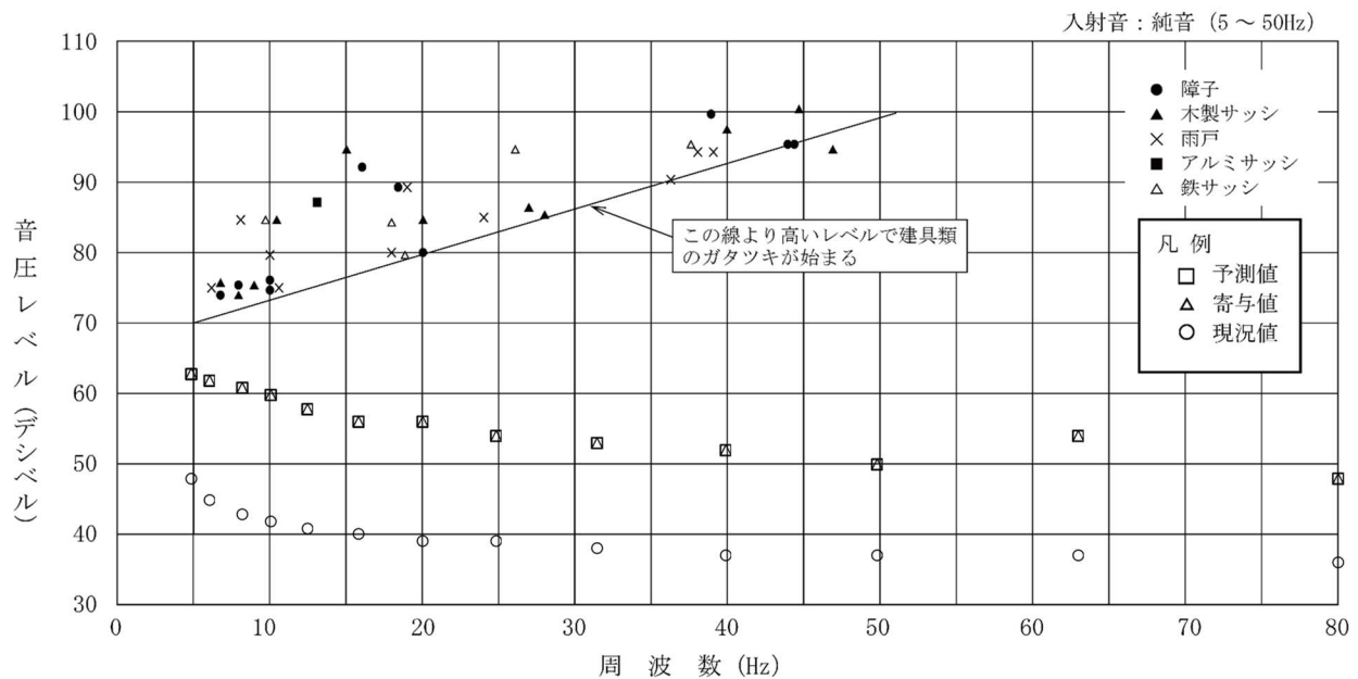
第 10.1.1-45 図(6) 建具のがたつきが始まるレベルとの比較結果 (累積的な影響：環境 6 地点、冬季 2)
