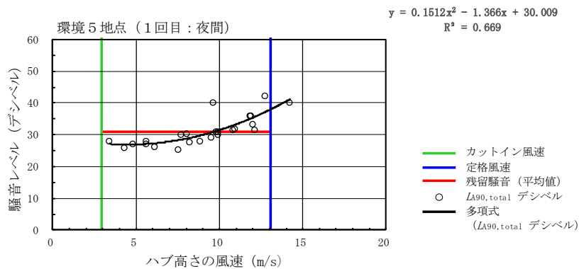
第 10.1.1-22 図(4) ハブ高さ風速と騒音レベル ( L_{A90+2} ) (1 回目：環境4地点)
