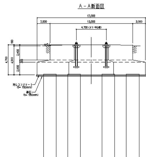
図 2.2-6(2) 風力発電機の基礎構造図 (参考)
