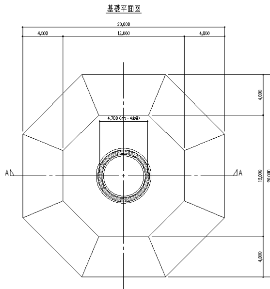
図 2.2-6(1) 風力発電機の基礎構造図 (参考)
