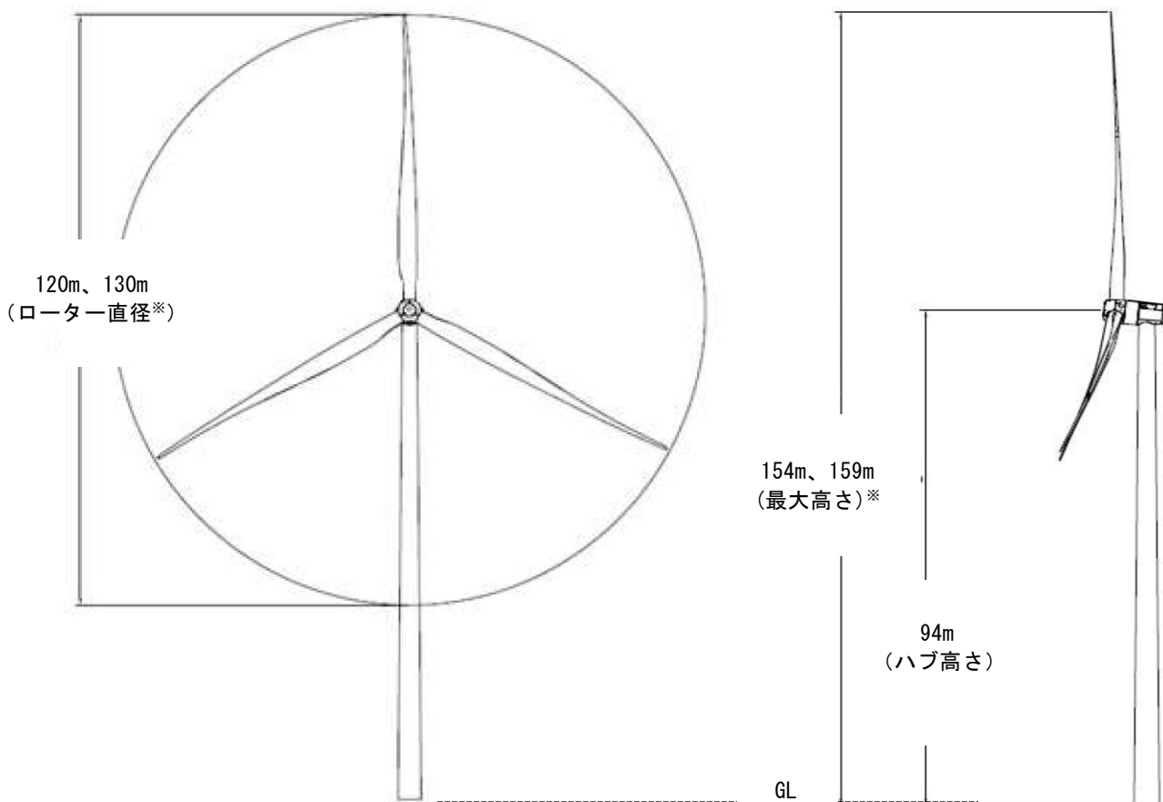
図 2.2-5 風力発電機の外形図
