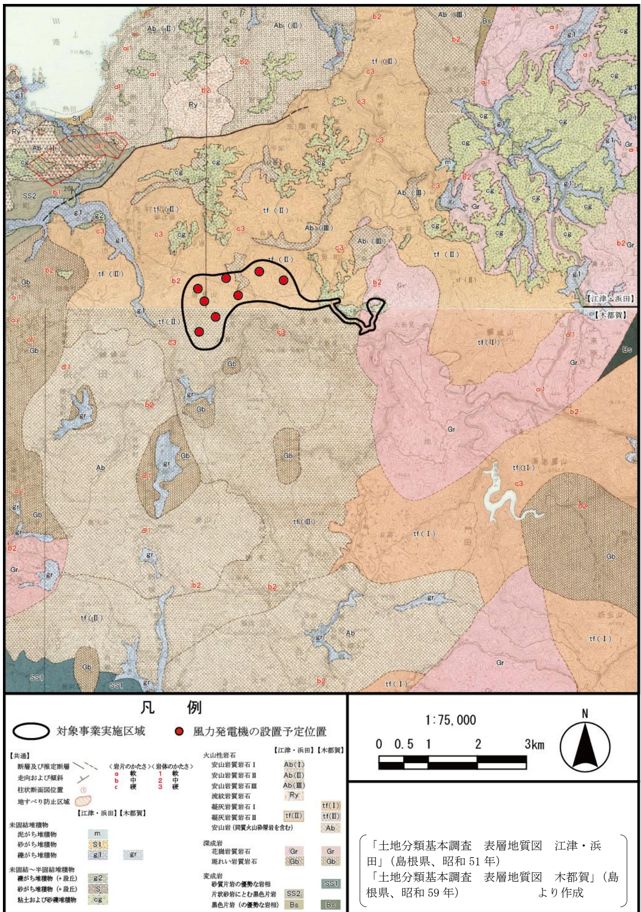
図 3.1-13 表層地質
