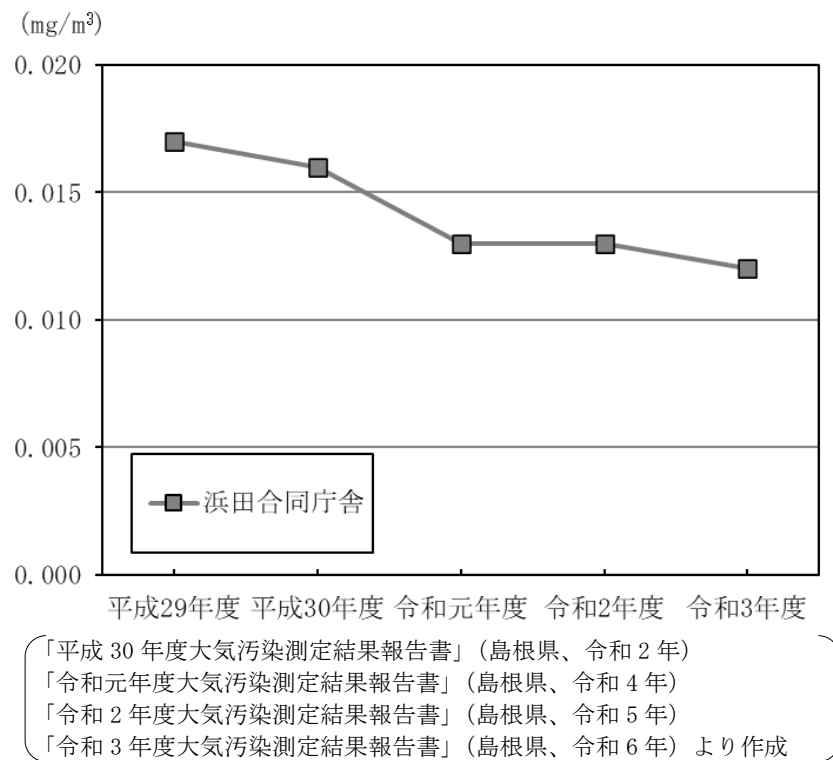
図 3.1-6 浮遊粒子状物質の年平均値の経年変化
