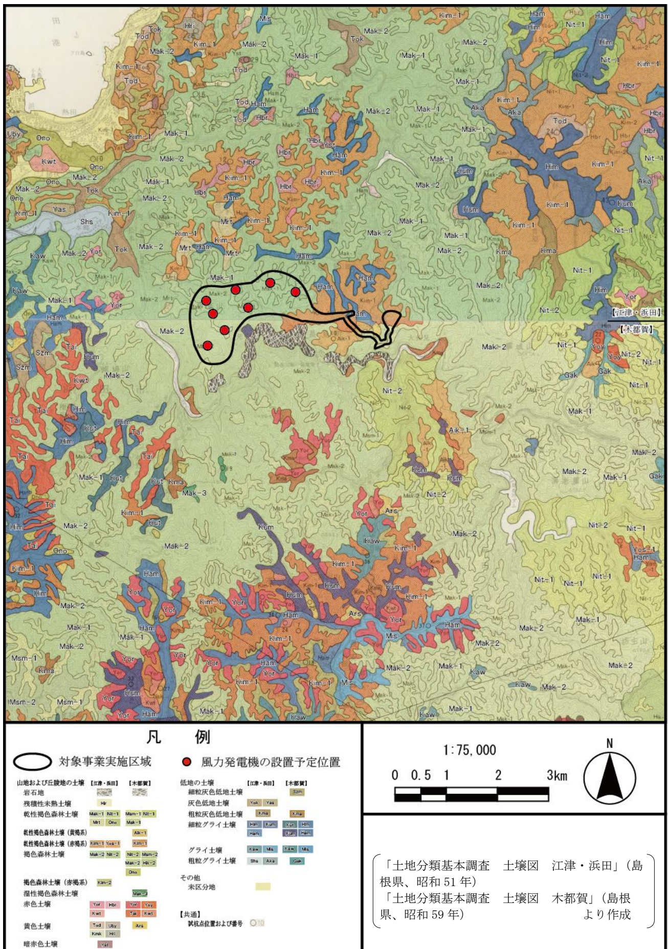
図 3.1-10 土壌図
