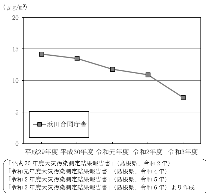
図 3.1-7 微小粒子状物質の年平均値の経年変化
