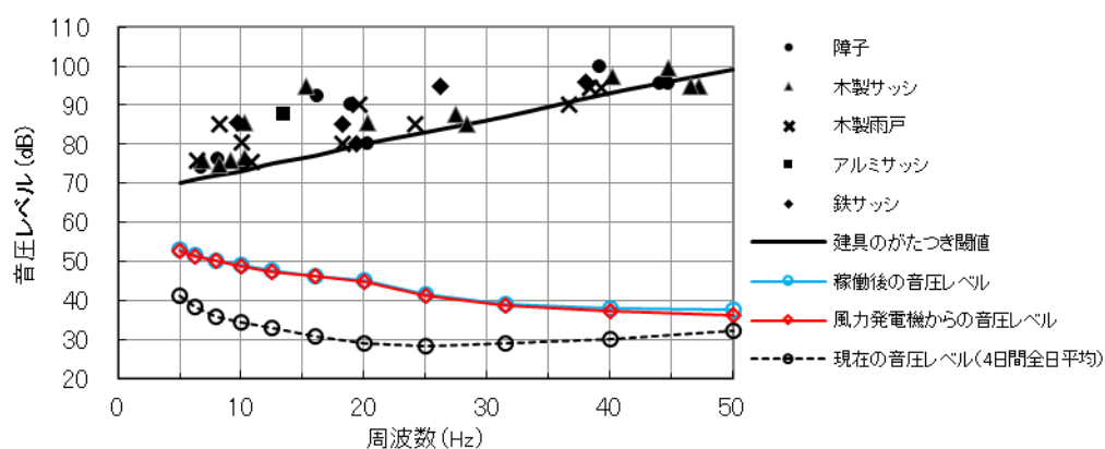
図 10.1.1.4-8(3) 建具のがたつきが始まるレベルとの比較結果 (秋季全日平均：環境 3)
