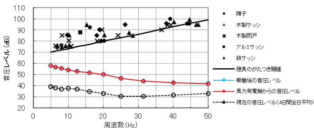
図 10.1.1.4-8(4) 建具のがたつきが始まるレベルとの比較結果
