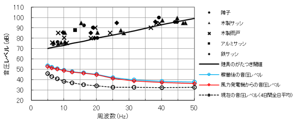
図 10.1.1.4-6(3) 建具のがたつきが始まるレベルとの比較結果 (春季全日平均：環境 3)
