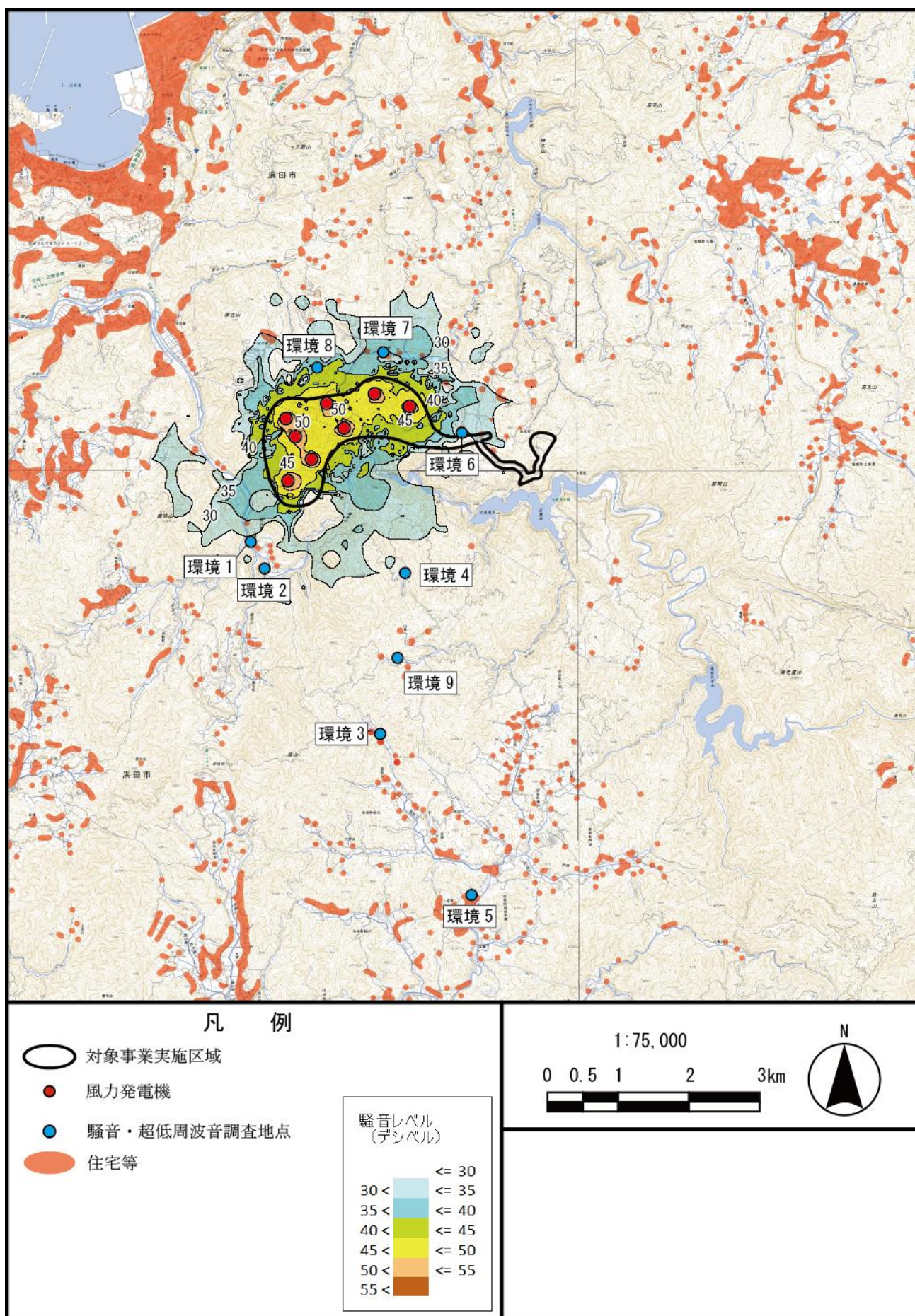
図 10.1.1.3-10(6) 風力発電機から発生する騒音の寄与値（秋季夜間環境 9、平均的な気象条件）
