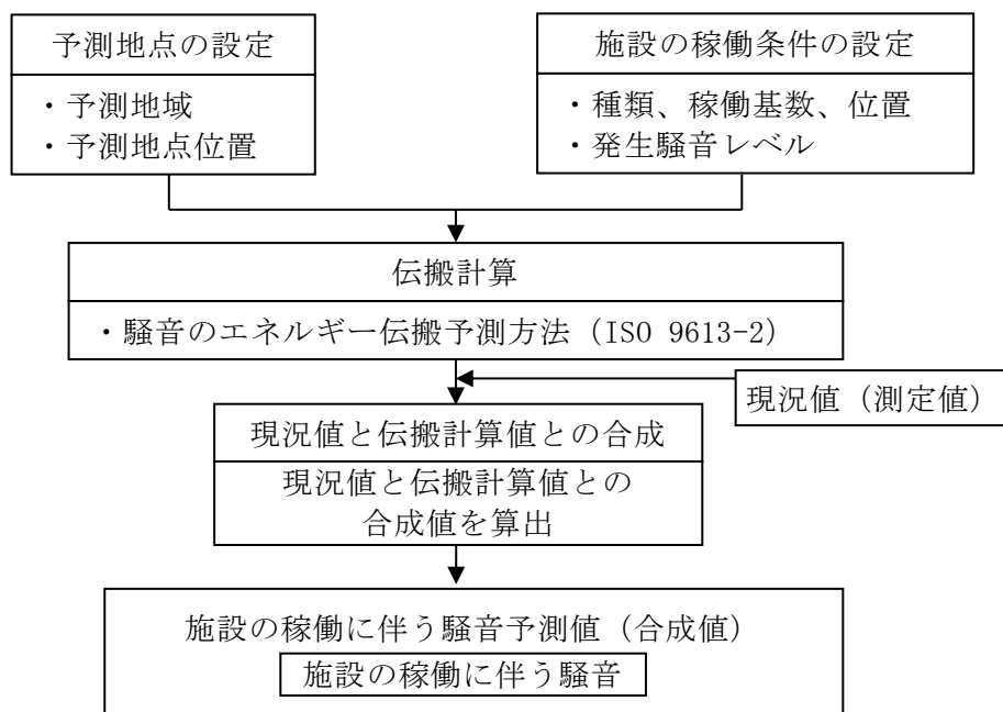
図 10. 1. 1. 3-9 施設の稼働に伴う騒音の予測手順
