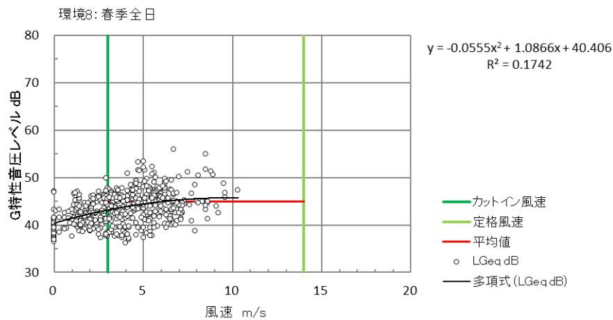
図 10.1.1.4-3(8) ハブ高さ風速（10 分間値）と G 特性等価音圧レベル（10 分間値）の関係 （秋季：環境 8）
