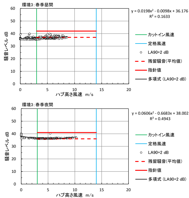
図 10.1.1.3-5(3) ハブ高さの風速と残留騒音レベル（春季：環境 3）
