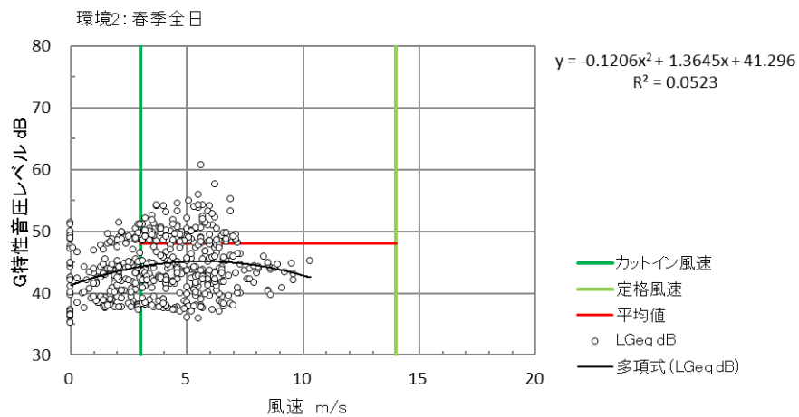
図 10.1.1.4-3(2) ハブ高さ風速（10 分間値）と G 特性等価音圧レベル（10 分間値）の関係 （春季：環境 2）
