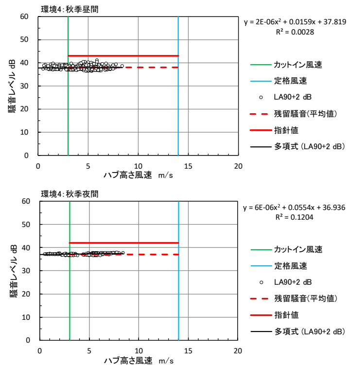
図 10.1.1.3-4(4) ハブ高さの風速と残留騒音レベル（秋季：環境 4）
