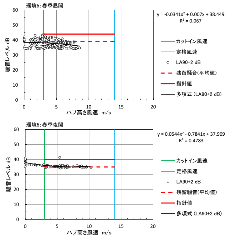
図 10.1.1.3-5(5) ハブ高さの風速と残留騒音レベル（春季：環境 5）
