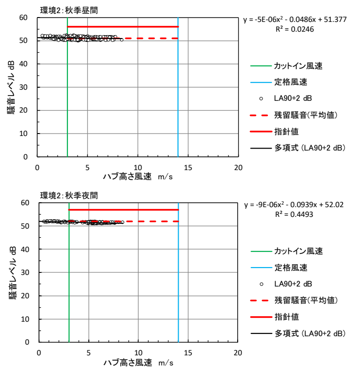
図 10.1.1.3-4(2) ハブ高さの風速と残留騒音レベル（秋季：環境 2）
