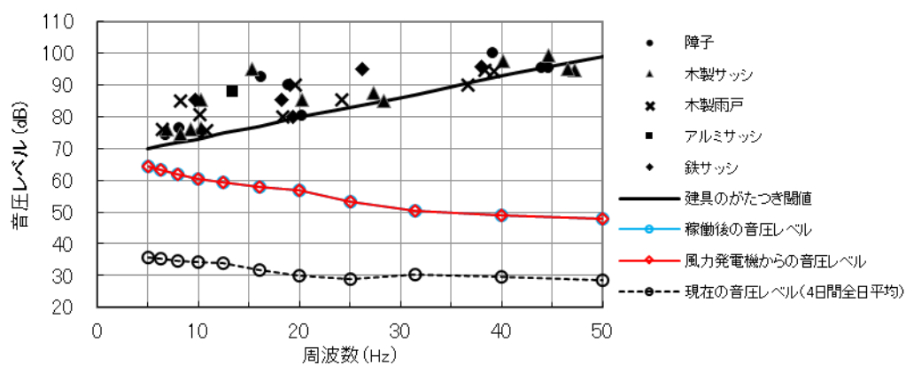
図 10.1.1.4-8(7) 建具のがたつきが始まるレベルとの比較結果 (秋季全日平均：環境 7)
