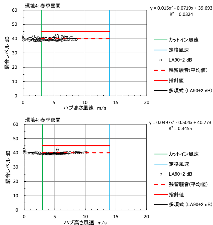
図 10.1.1.3-5(4) ハブ高さの風速と残留騒音レベル（春季：環境 4）
