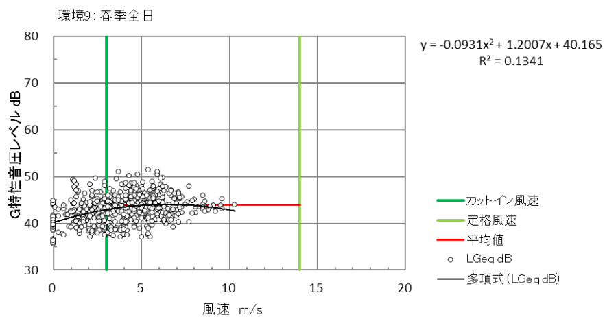
図 10.1.1.4-3(9) ハブ高さ風速（10 分間値）と G 特性等価音圧レベル（10 分間値）の関係 （春季：環境 9）
