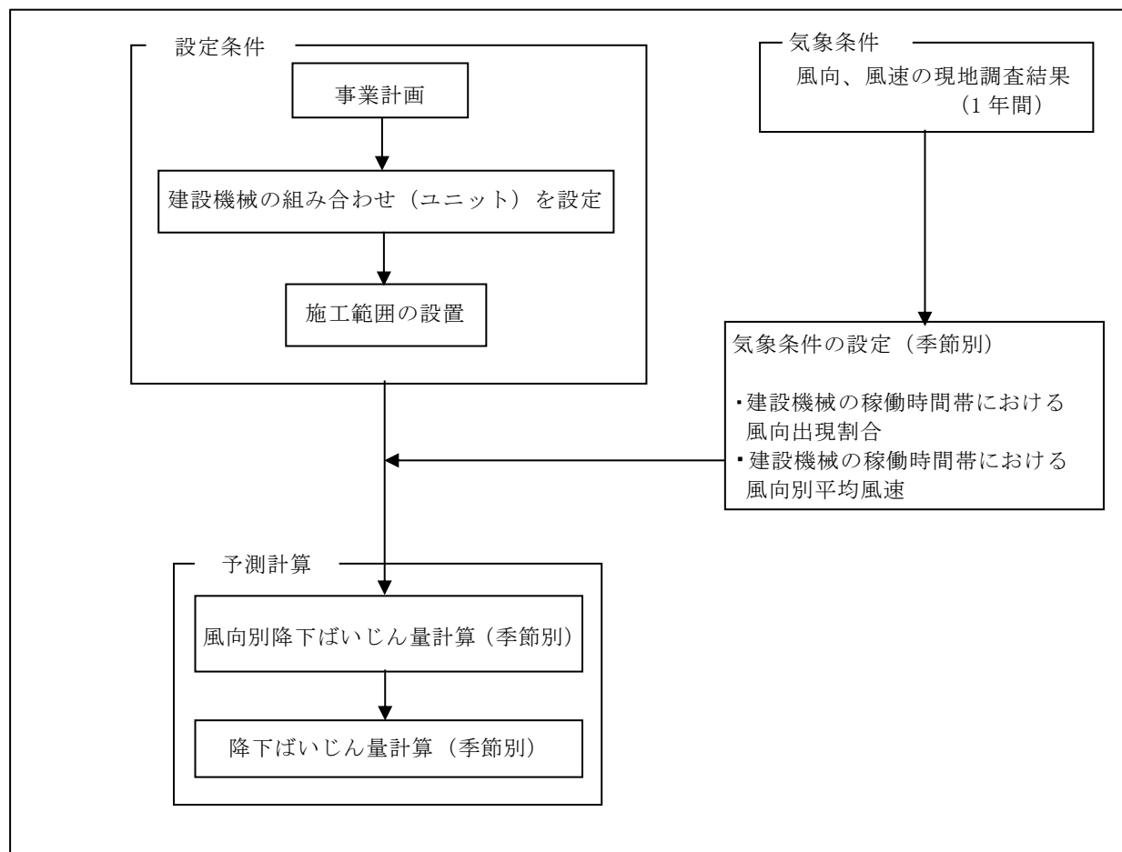
図 10.1.1.2-4 建設機械の稼働に伴う粉じん等の予測手順
