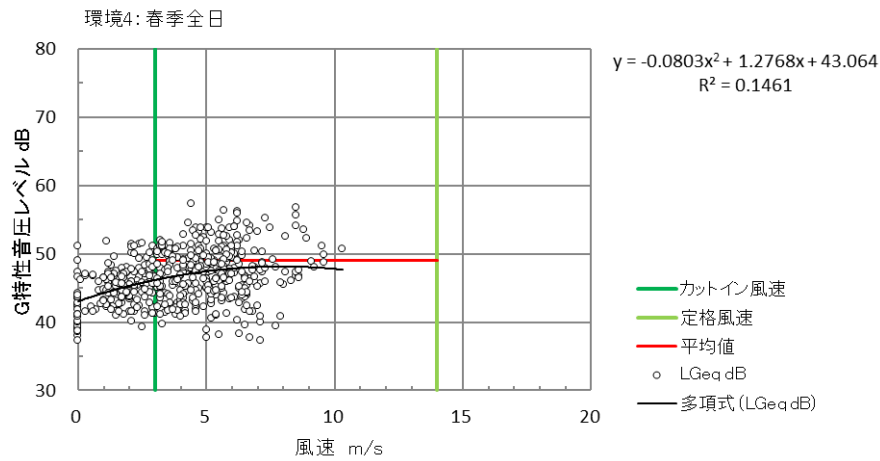
図 10.1.1.4-3(4) ハブ高さ風速（10 分間値）と G 特性等価音圧レベル（10 分間値）の関係 （春季：環境 4）
