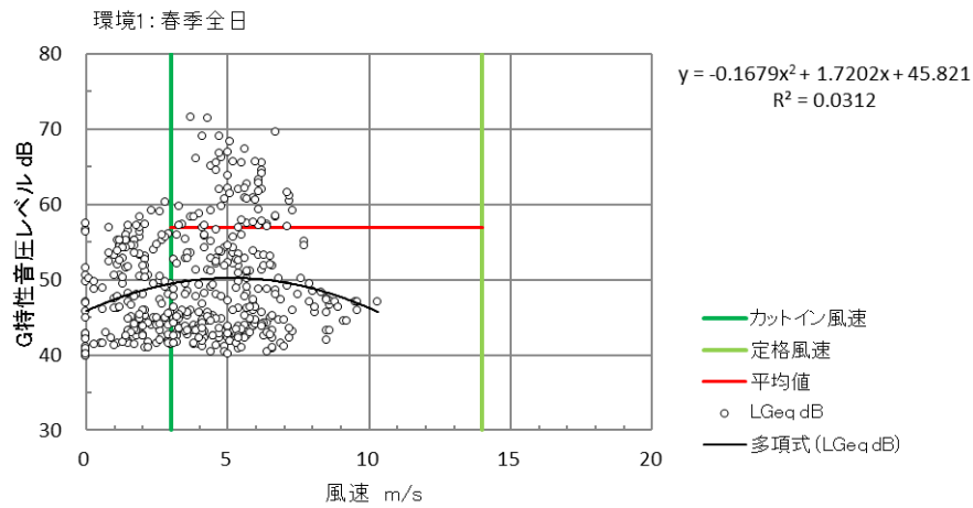
図 10.1.1.4-3(1) ハブ高さ風速（10 分間値）と G 特性等価音圧レベル（10 分間値）の関係 （春季：環境 1）
