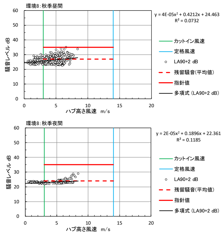
図 10.1.1.3-4(8) ハブ高さの風速と残留騒音レベル（秋季：環境 8）
