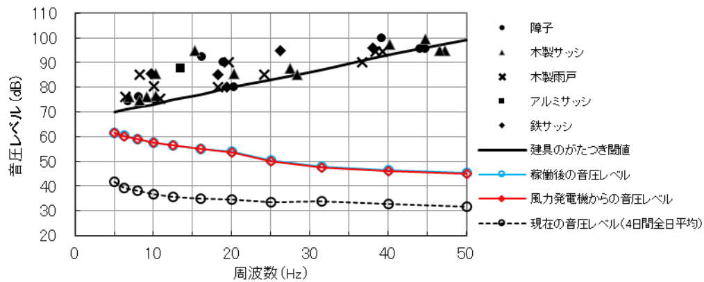
図 10.1.1.4-6(6) 建具のがたつきが始まるレベルとの比較結果 (春季全日平均：環境 6)
