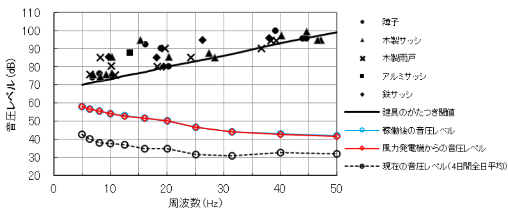
図 10.1.1.4-6(4) 建具のがたつきが始まるレベルとの比較結果 (春季全日平均：環境 4)
