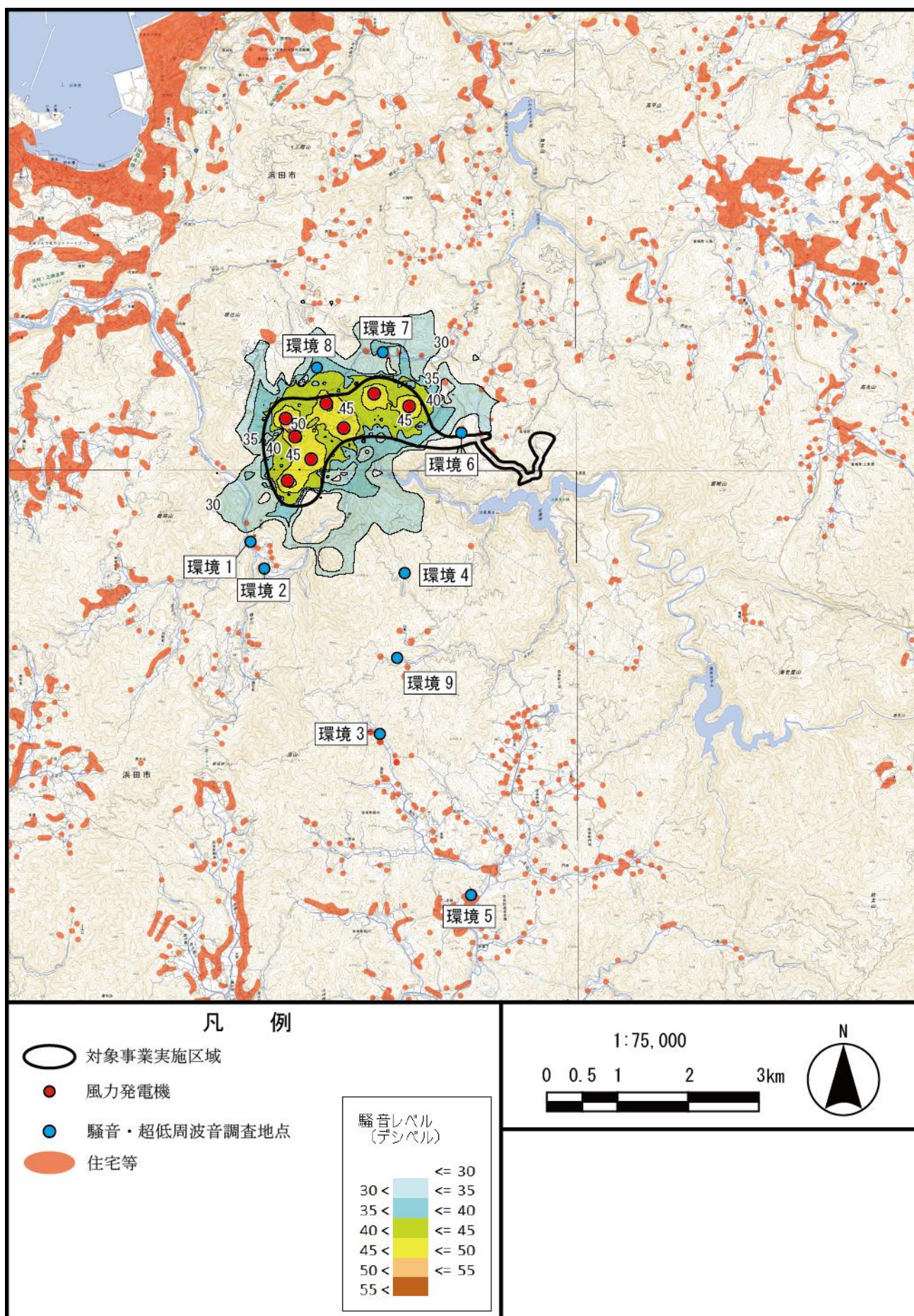
図 10.1.1.3-10(1) 風力発電機から発生する騒音の寄与値（春季昼間、平均的な気象条件）
