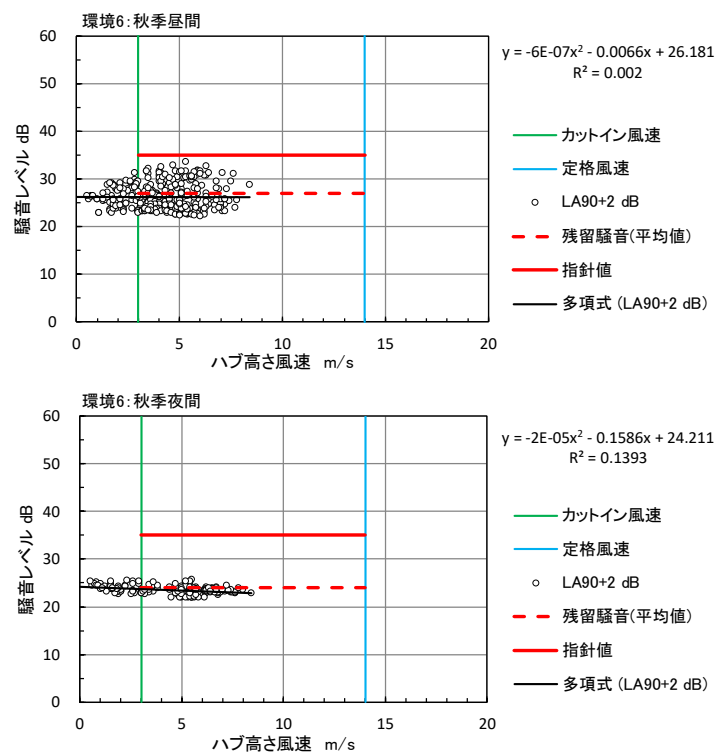
図 10.1.1.3-4(6) ハブ高さの風速と残留騒音レベル（秋季：環境 6）
