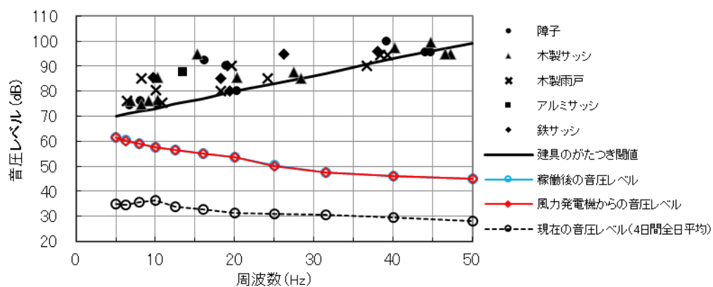
図 10.1.1.4-8(6) 建具のがたつきが始まるレベルとの比較結果
