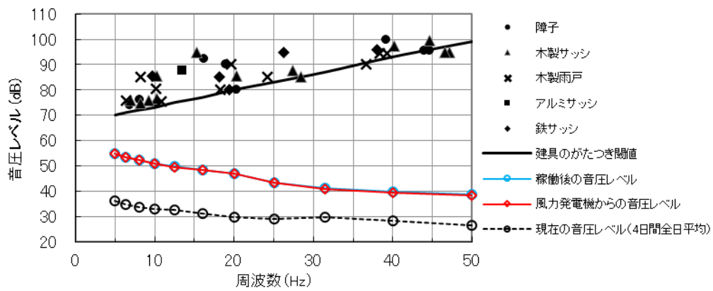
図 10.1.1.4-6(8) 建具のがたつきが始まるレベルとの比較結果
