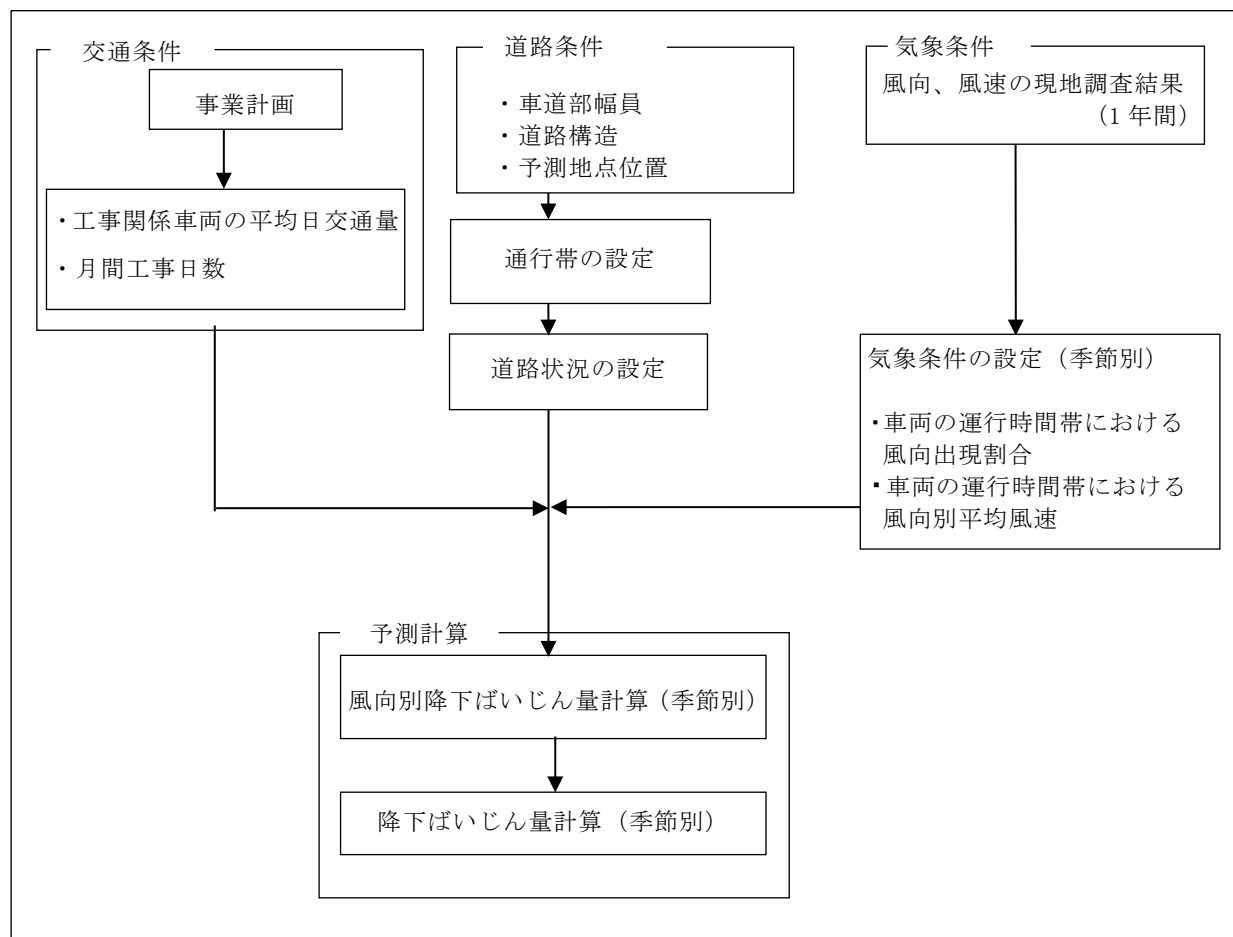
図 10.1.1.2-1 工事用資材等の搬出入に伴う粉じん等の予測手順
