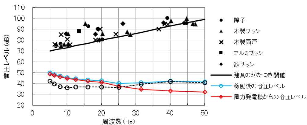
図 10.1.1.4-8(5) 建具のがたつきが始まるレベルとの比較結果
