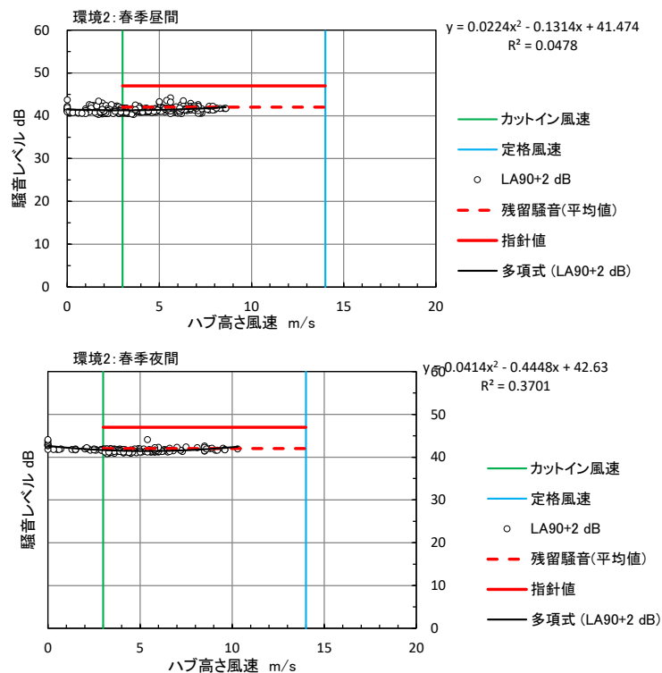
図 10.1.1.3-5(2) ハブ高さの風速と残留騒音レベル（春季：環境 2）
