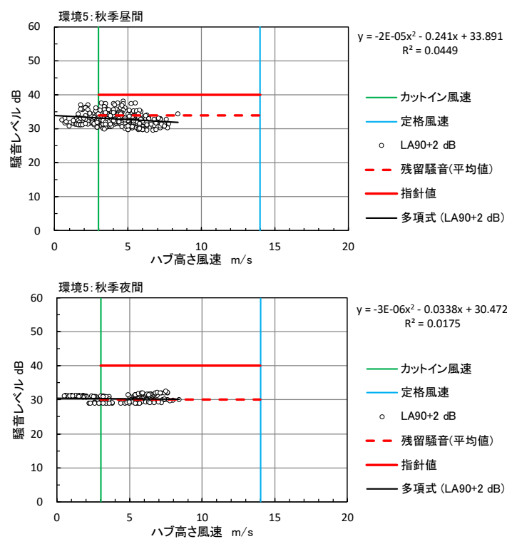
図 10.1.1.3-4(5) ハブ高さの風速と残留騒音レベル（秋季：環境 5）
