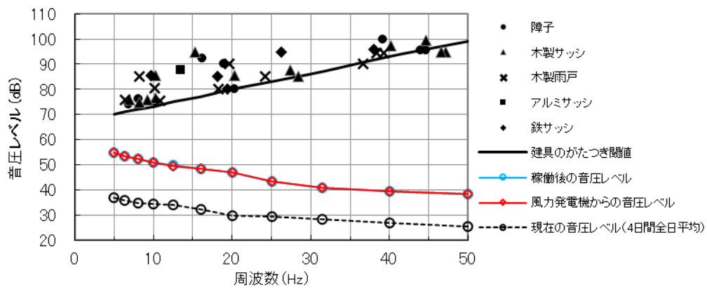
図 10.1.1.4-8(8) 建具のがたつきが始まるレベルとの比較結果
