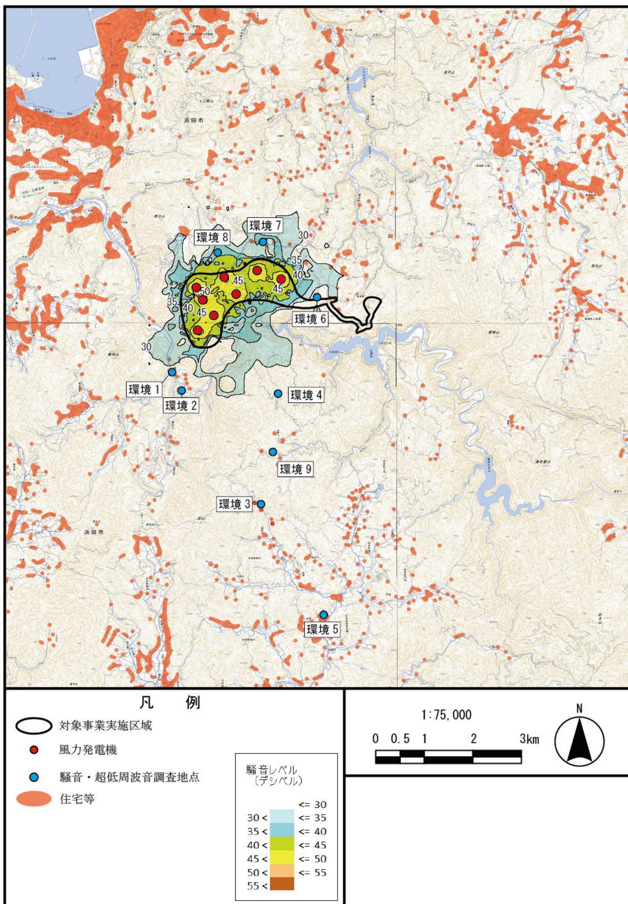
図 10.1.1.3-10(2) 風力発電機から発生する騒音の寄与値（春季夜間、平均的な気象条件）
