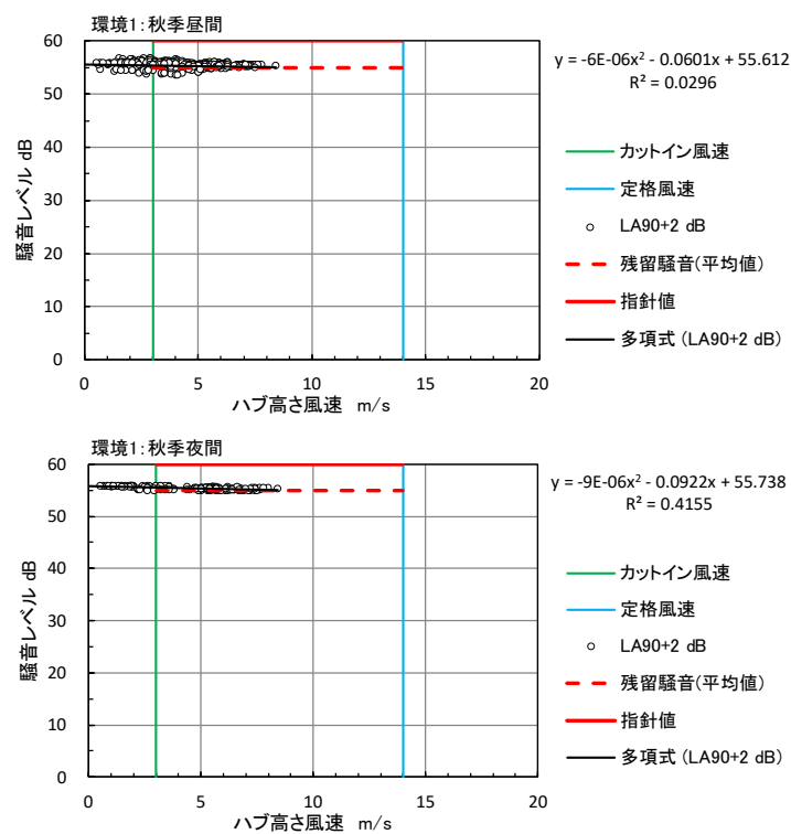
図 10.1.1.3-4(1) ハブ高さの風速と残留騒音レベル（秋季：環境 1）
