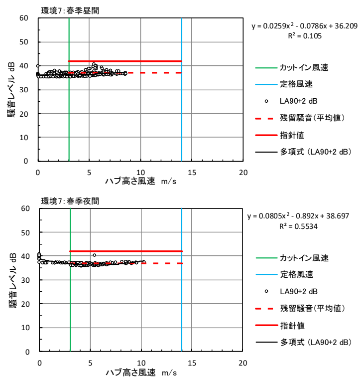
図 10.1.1.3-5(7) ハブ高さの風速と残留騒音レベル（春季：環境 7）
