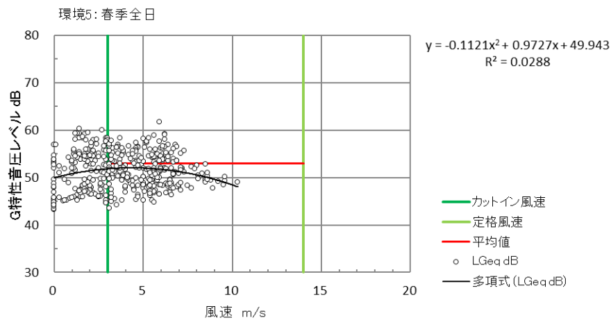
図 10.1.1.4-3(5) ハブ高さ風速（10 分間値）と G 特性等価音圧レベル（10 分間値）の関係 （春季：環境 5）
