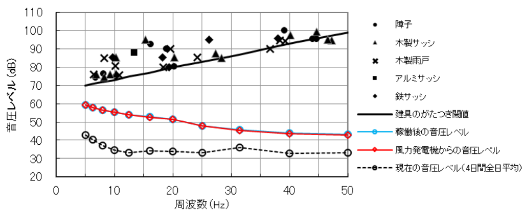
図 10.1.1.4-6(2) 建具のがたつきが始まるレベルとの比較結果 (春季全日平均：環境 2)
