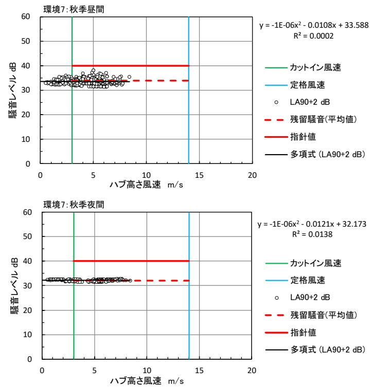
図 10.1.1.3-4(7) ハブ高さの風速と残留騒音レベル（秋季：環境 7）
