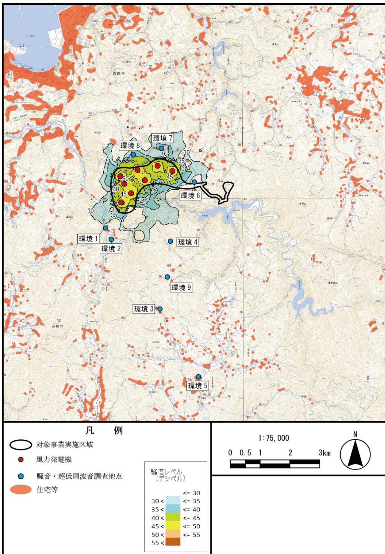
図 10.1.1.3-10(5) 風力発電機から発生する騒音の寄与値 (秋季夜間環境1～環境8、平均的な気象条件)
