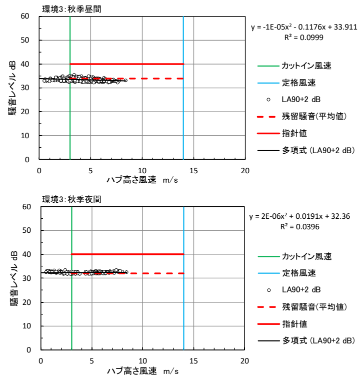
図 10.1.1.3-4(3) ハブ高さの風速と残留騒音レベル（秋季：環境 3）
