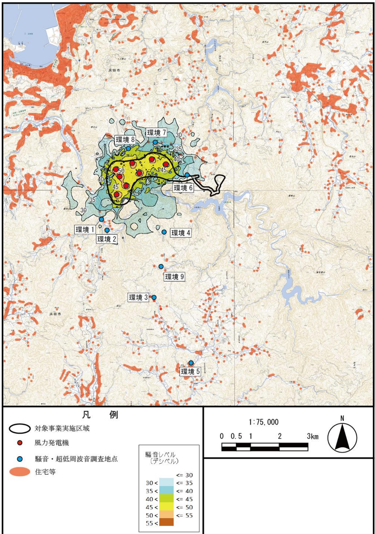
図 10.1.1.3-10(4) 風力発電機から発生する騒音の寄与値（秋季昼間環境 9、平均的な気象条件）
