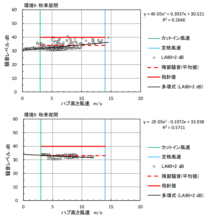
図 10.1.1.3-4(9) ハブ高さの風速と残留騒音レベル（秋季：環境 9）
