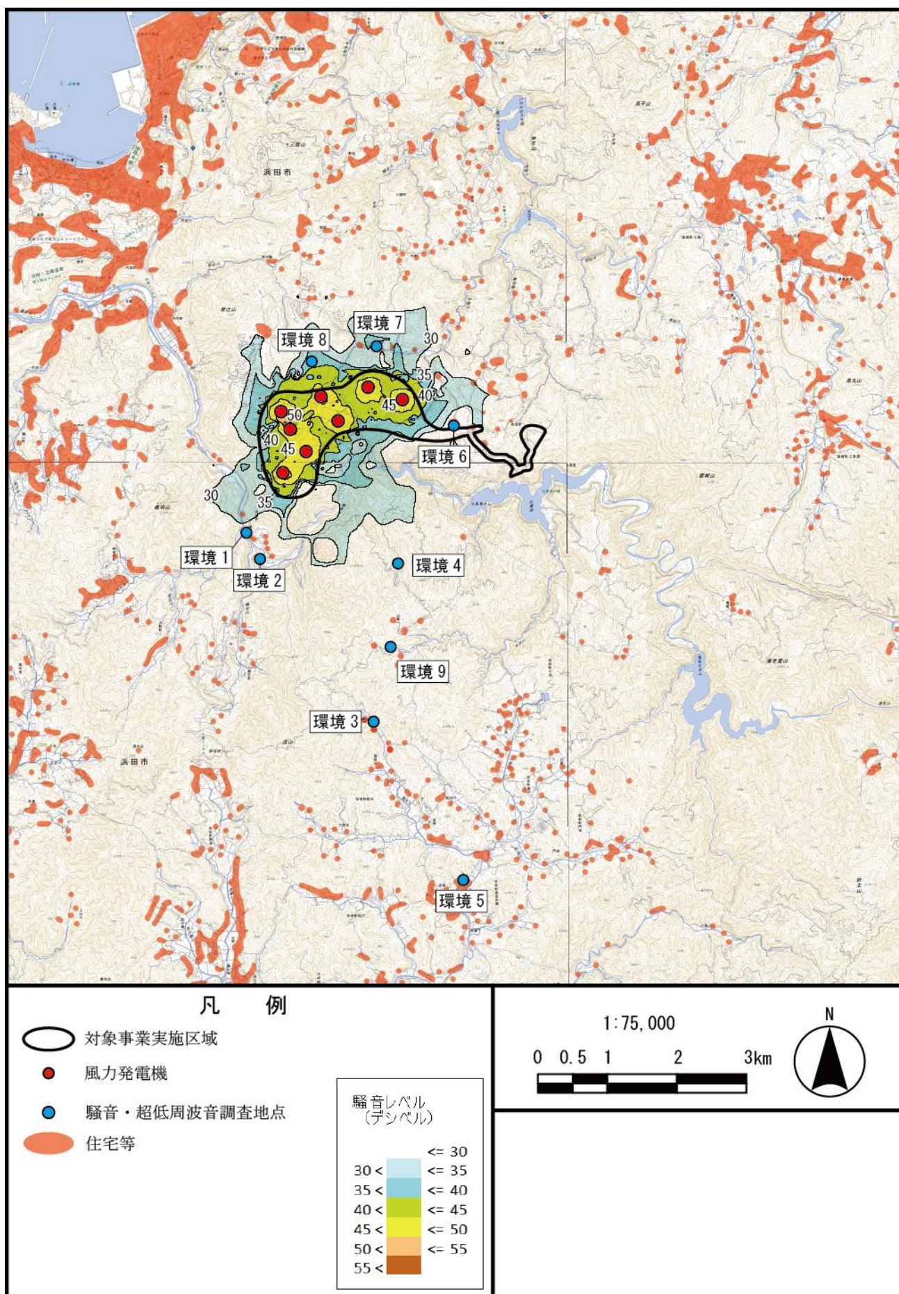
図 10.1.1.3-10(3) 風力発電機から発生する騒音の寄与値 (秋季昼間環境1～環境8、平均的な気象条件)
