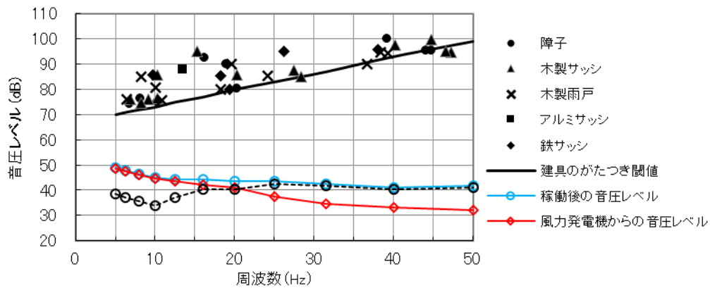
図 10.1.1.4-6(5) 建具のがたつきが始まるレベルとの比較結果
