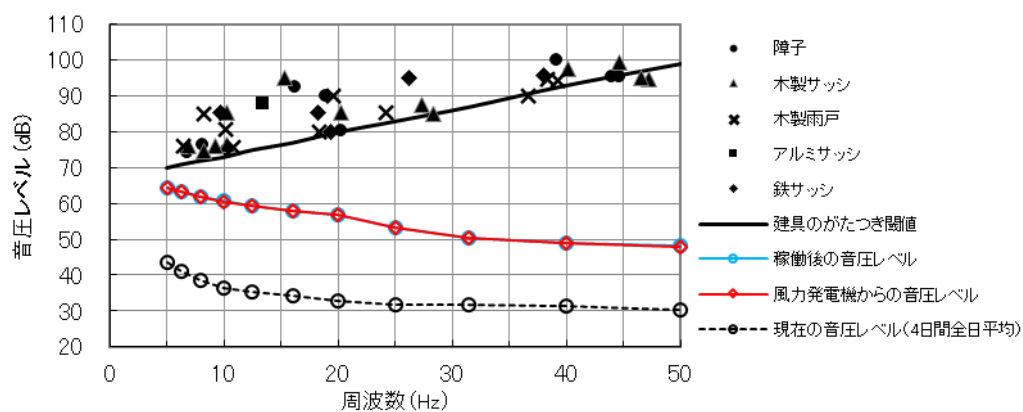
図 10.1.1.4-6(7) 建具のがたつきが始まるレベルとの比較結果 (春季全日平均：環境 7)
