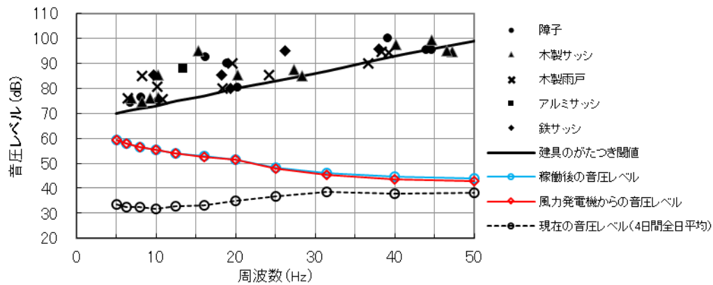
図 10.1.1.4-8(2) 建具のがたつきが始まるレベルとの比較結果 (秋季全日平均：環境 2)
