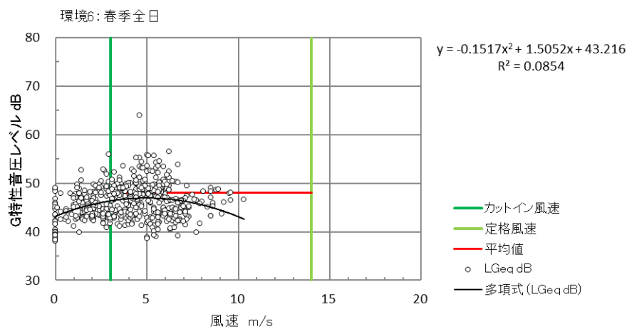
図 10.1.1.4-3(6) ハブ高さ風速（10 分間値）と G 特性等価音圧レベル（10 分間値）の関係 （春季：環境 6）
