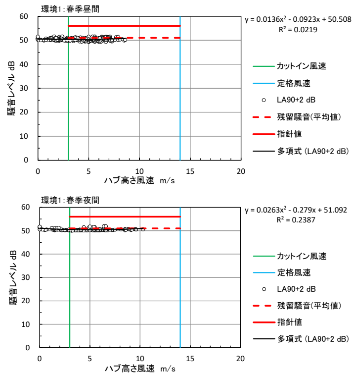
図 10.1.1.3-5(1) ハブ高さの風速と残留騒音レベル（春季：環境 1）
