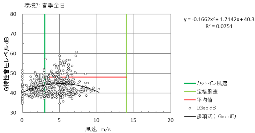
図 10.1.1.4-3(7) ハブ高さ風速（10 分間値）と G 特性等価音圧レベル（10 分間値）の関係 （春季：環境 7）
