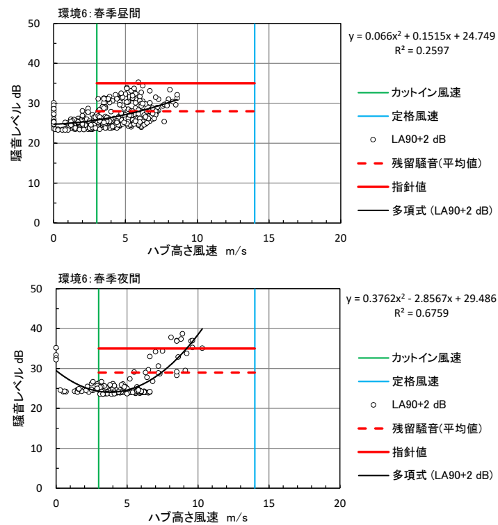
図 10.1.1.3-5(6) ハブ高さの風速と残留騒音レベル（春季：環境 6）
