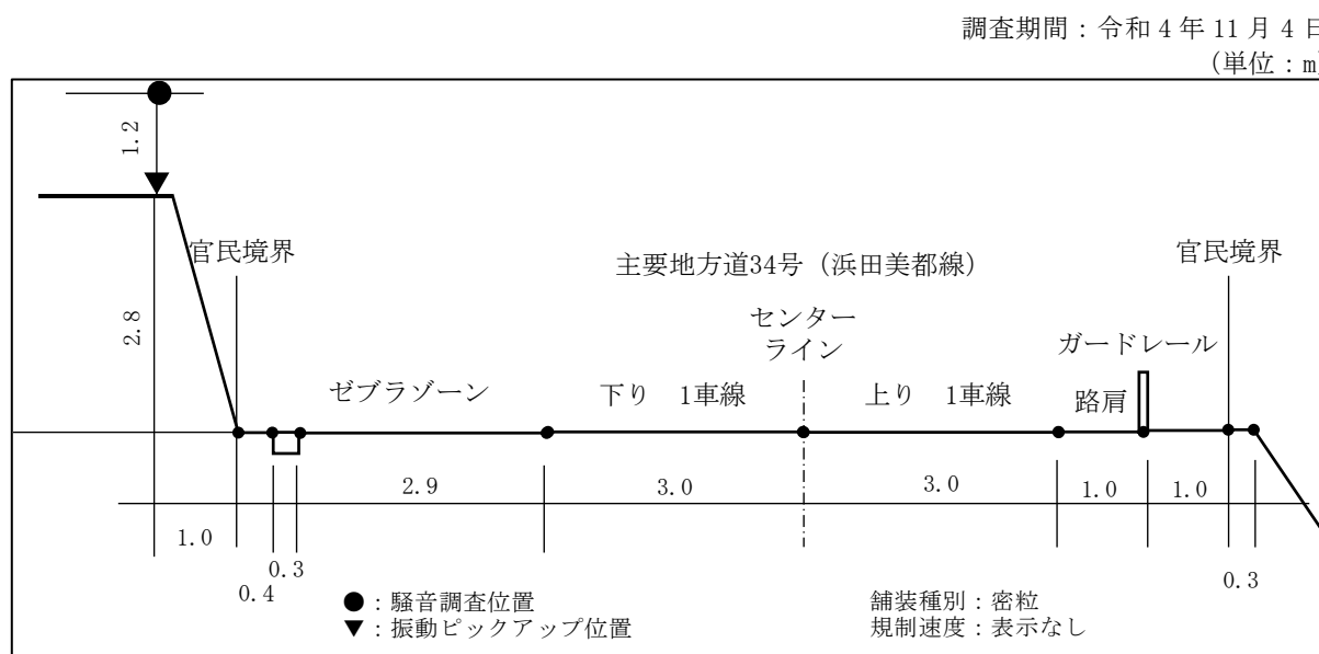
図 10.1.1.1-3(1) 調査地点の道路断面構造等（沿道 1 主要地方道 34 号(浜田美都線)）
