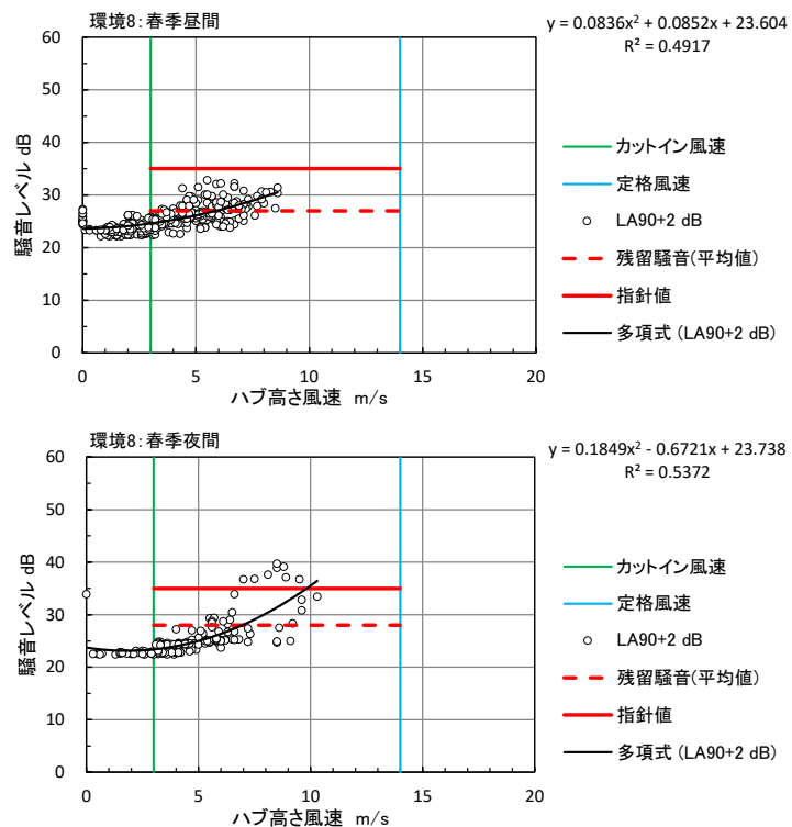
図 10.1.1.3-5(8) ハブ高さの風速と残留騒音レベル（春季：環境 8）
