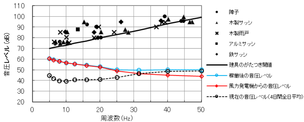
図 10.1.1.4-8(1) 建具のがたつきが始まるレベルとの比較結果 (秋季全日平均：環境 1)
