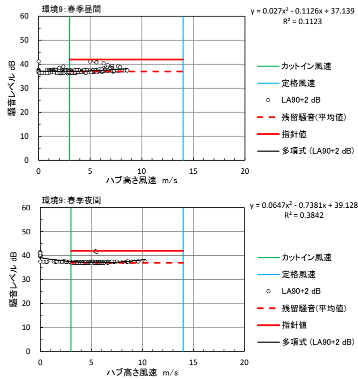
図 10.1.1.3-5(9) ハブ高さの風速と残留騒音レベル（春季：環境 9）
