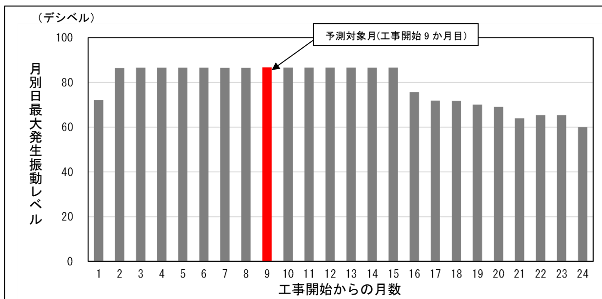
図 12.1.1-26 建設機械の月別発生振動レベル
