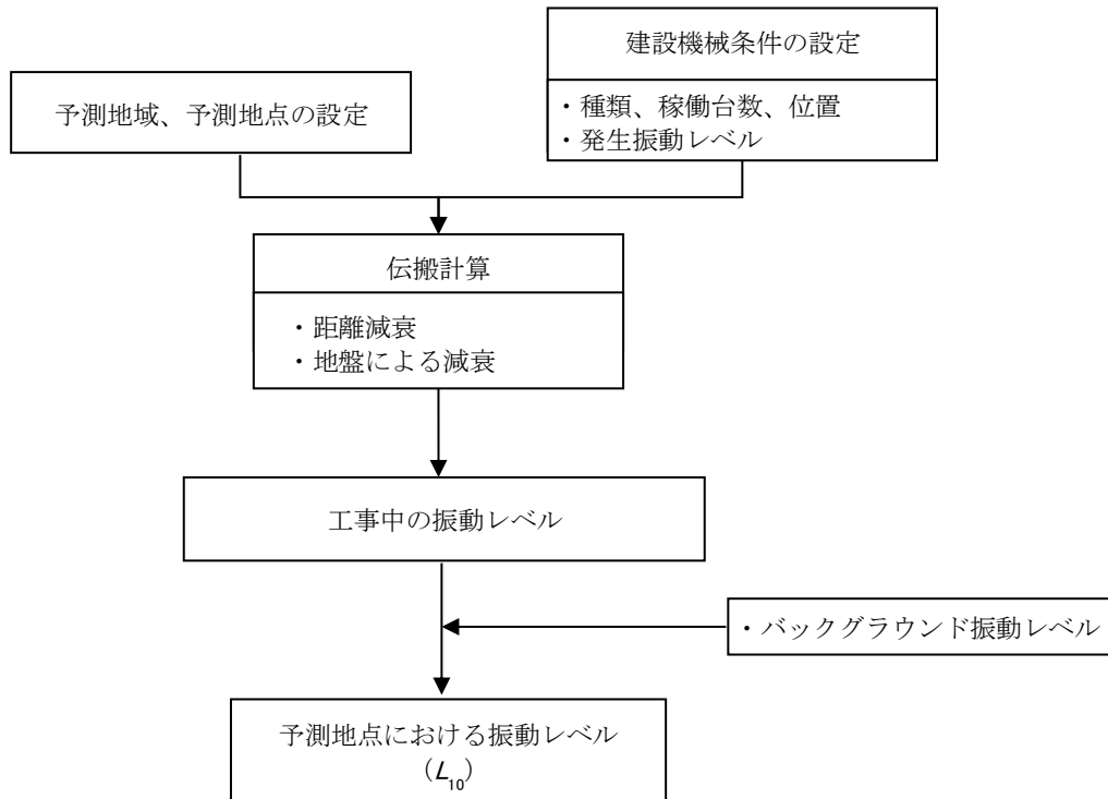
図 12. 1. 1-28 建設機械の稼働に伴う振動の予測手順
