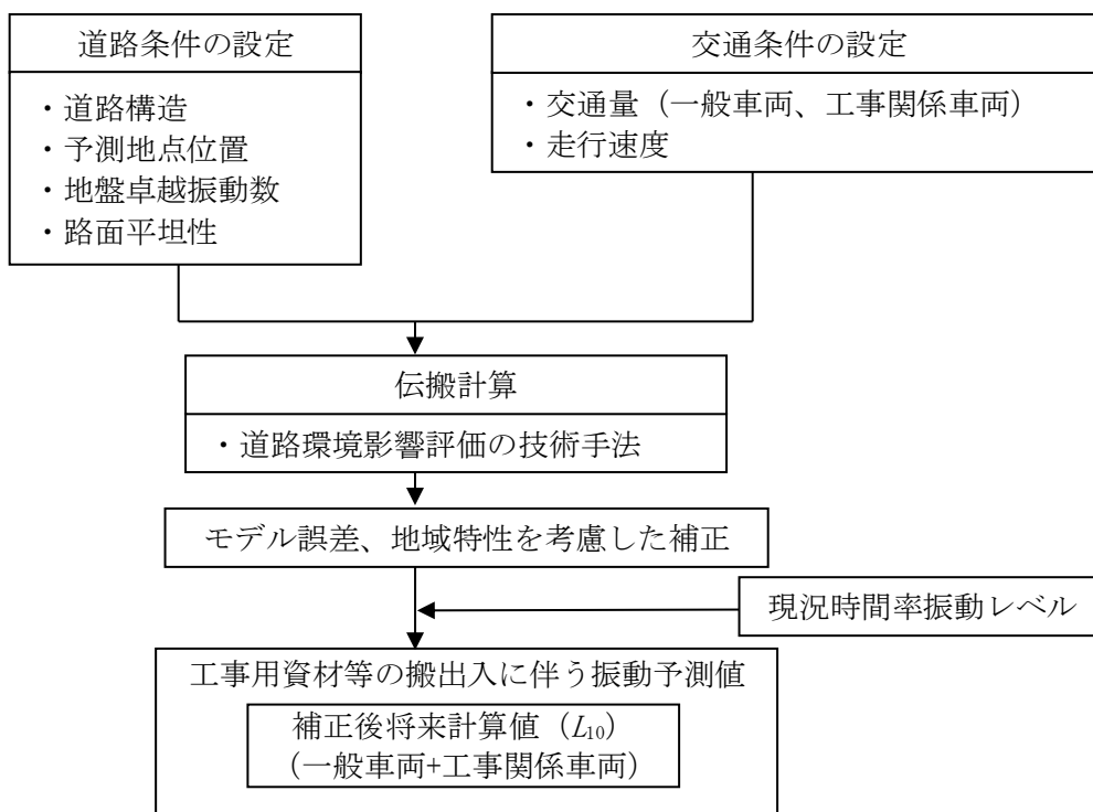
図 12.1.1-25 工事関係車両による振動の予測手順
