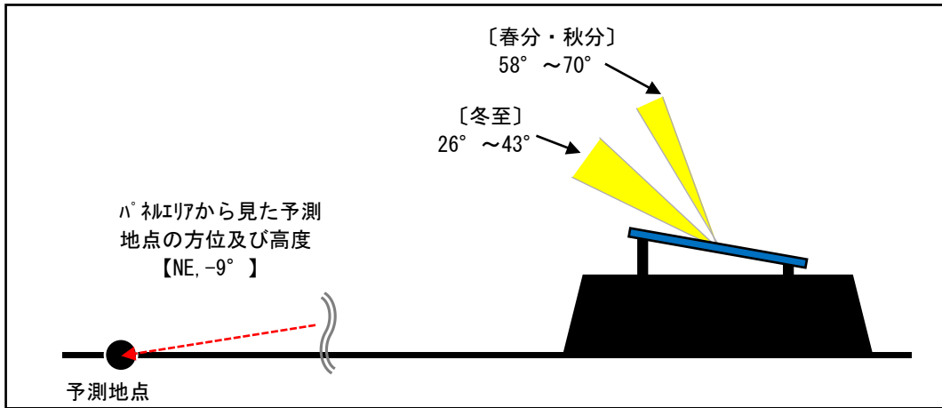
図 12.1.3-25 (1) 反射光高度及び予測地点高度のイメージ (福谷地区 断面②)
