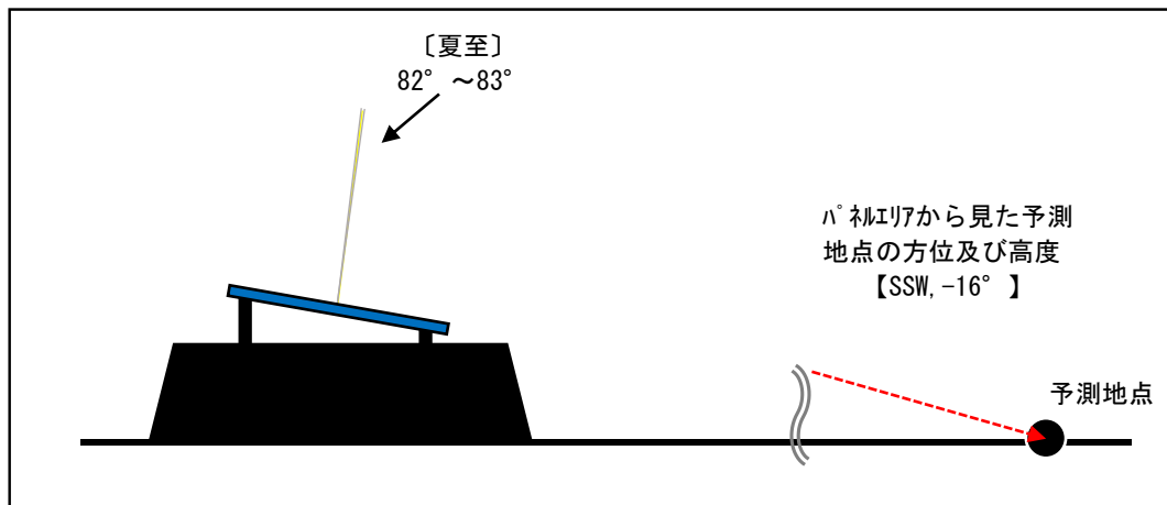
図 12.1.3-25 (3) 反射光高度及び予測地点高度のイメージ (荒田地区 断面⑤)
