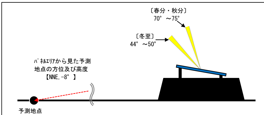
図 12.1.3-25 (2) 反射光高度及び予測地点高度のイメージ (福谷地区 断面③)
