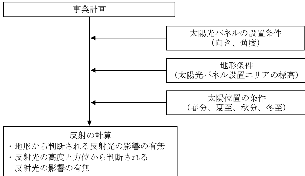
図 12.1.3-21 反射光の予測手順
