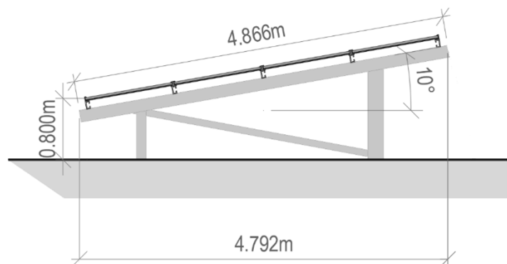
図 12.1.3-22 太陽光パネルの設置模式図
