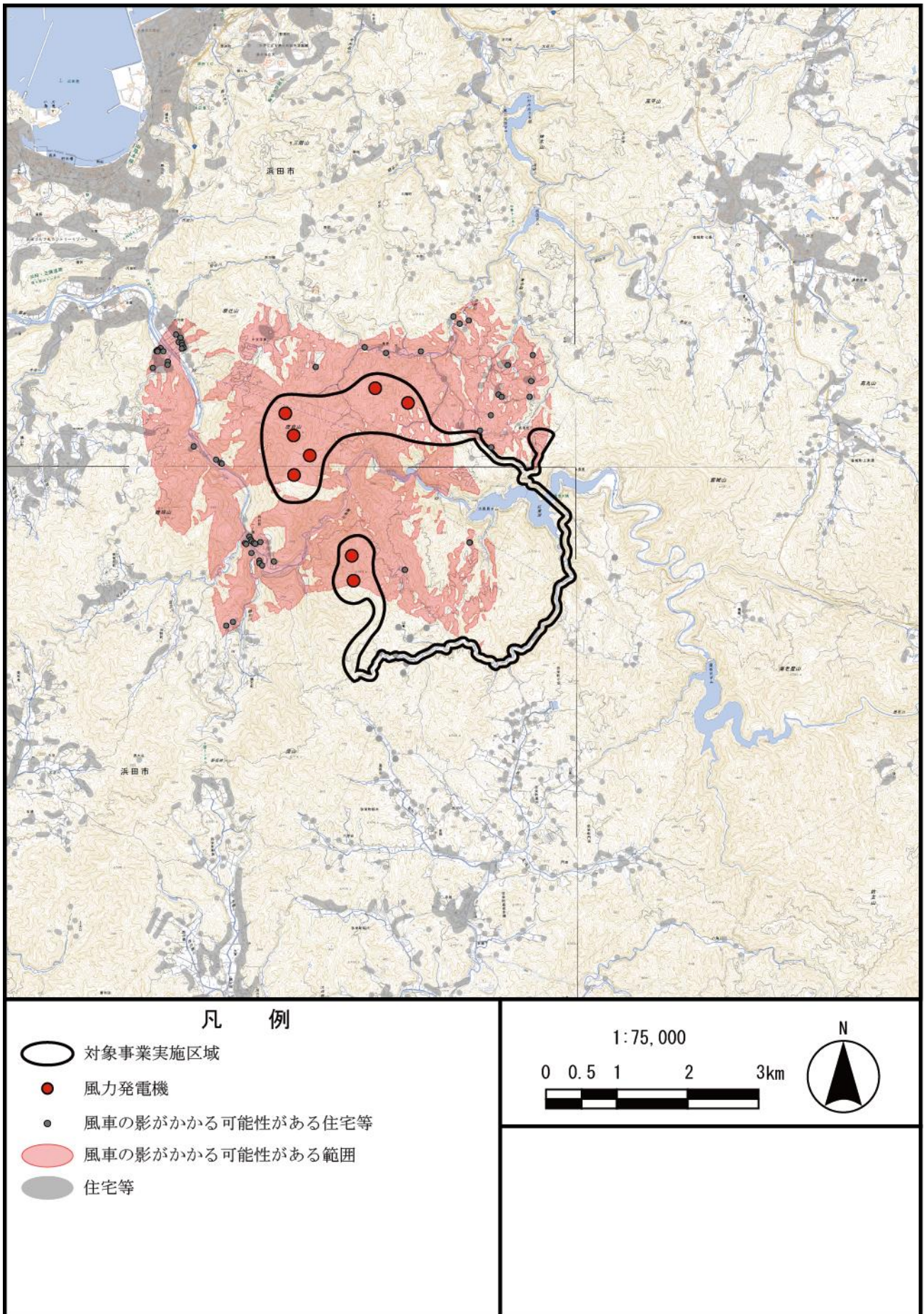
図 10.1.3.2-4 本事業の風力発電機により風車の影がかかる可能性がある範囲
