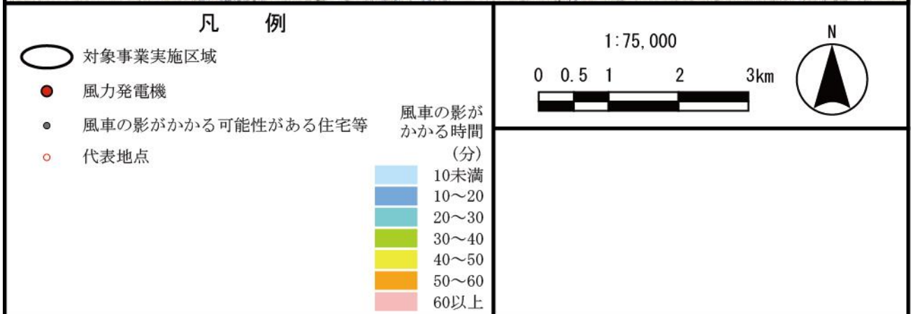
図 10.1.3.2-6(1) 等時間日影図 (冬至)
