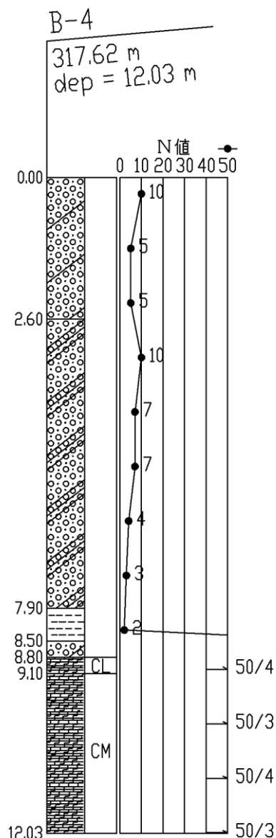
図 12.1.3-6(4) ボーリング柱状図 (B-4)
