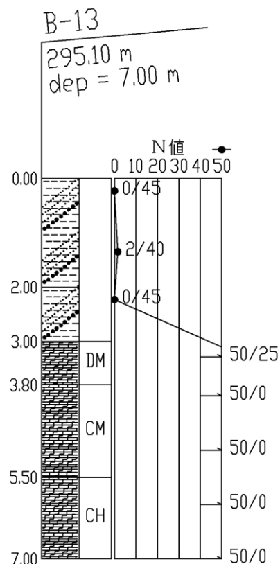
図 12.1.3-6(13) ボーリング柱状図 (B-13)
