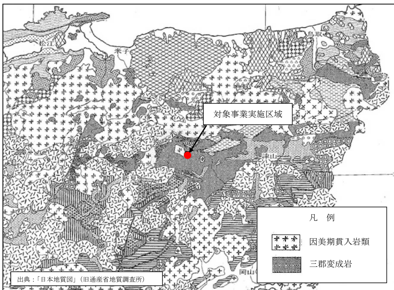
図 12.1.3-3 地質図
