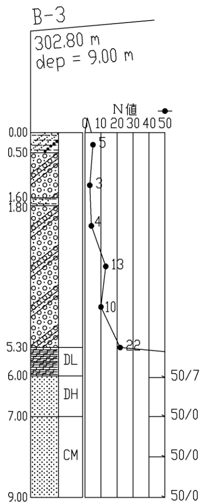
図 12.1.3-6(3) ボーリング柱状図 (B-3)
