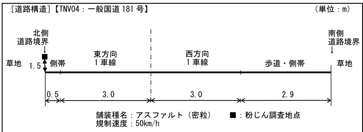
図 12.1.1-4 交通量調査地点及び粉じん等調査・予測地点の道路断面構造
