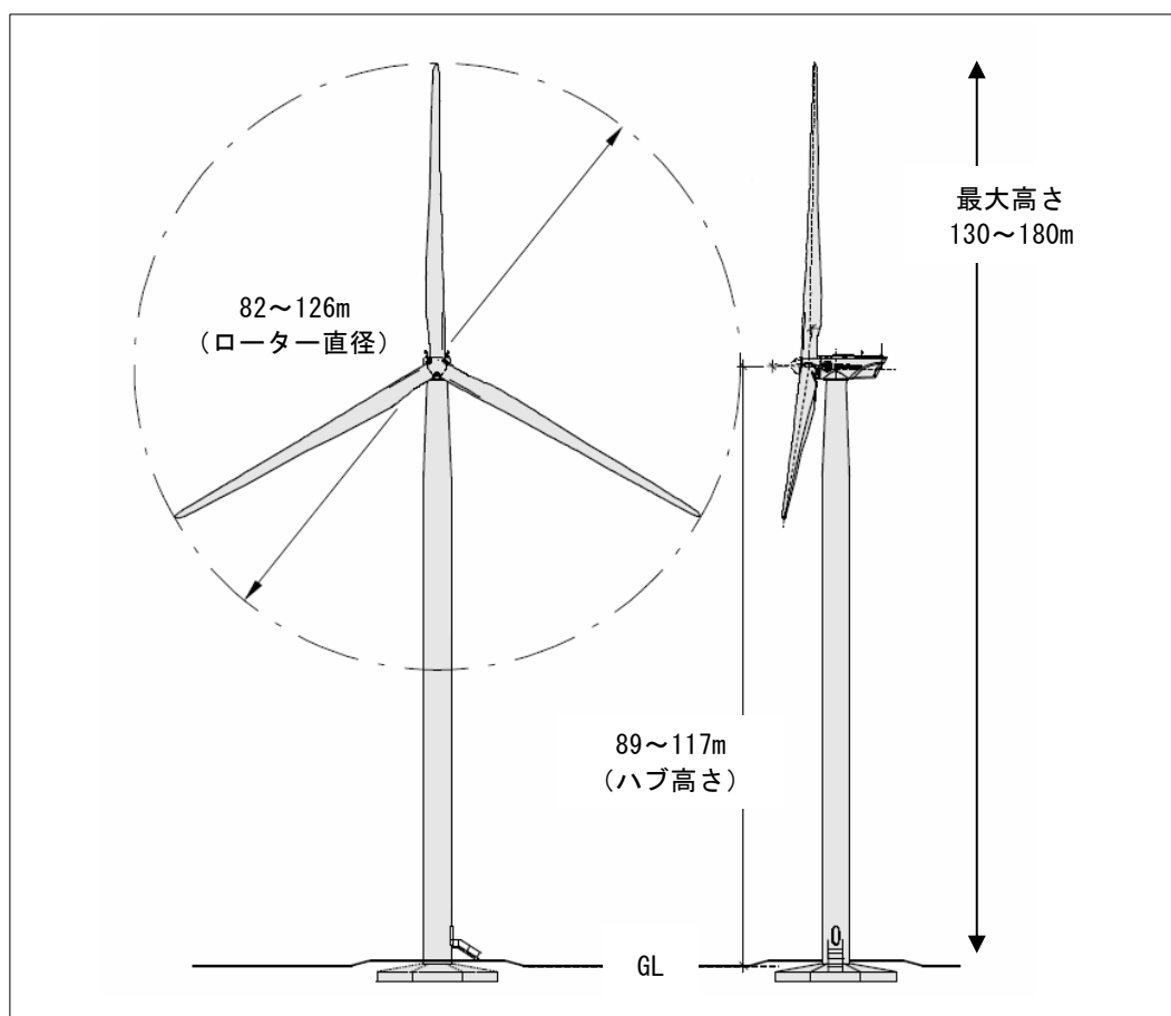
図 12. 2-9 風力発電機の概略図
