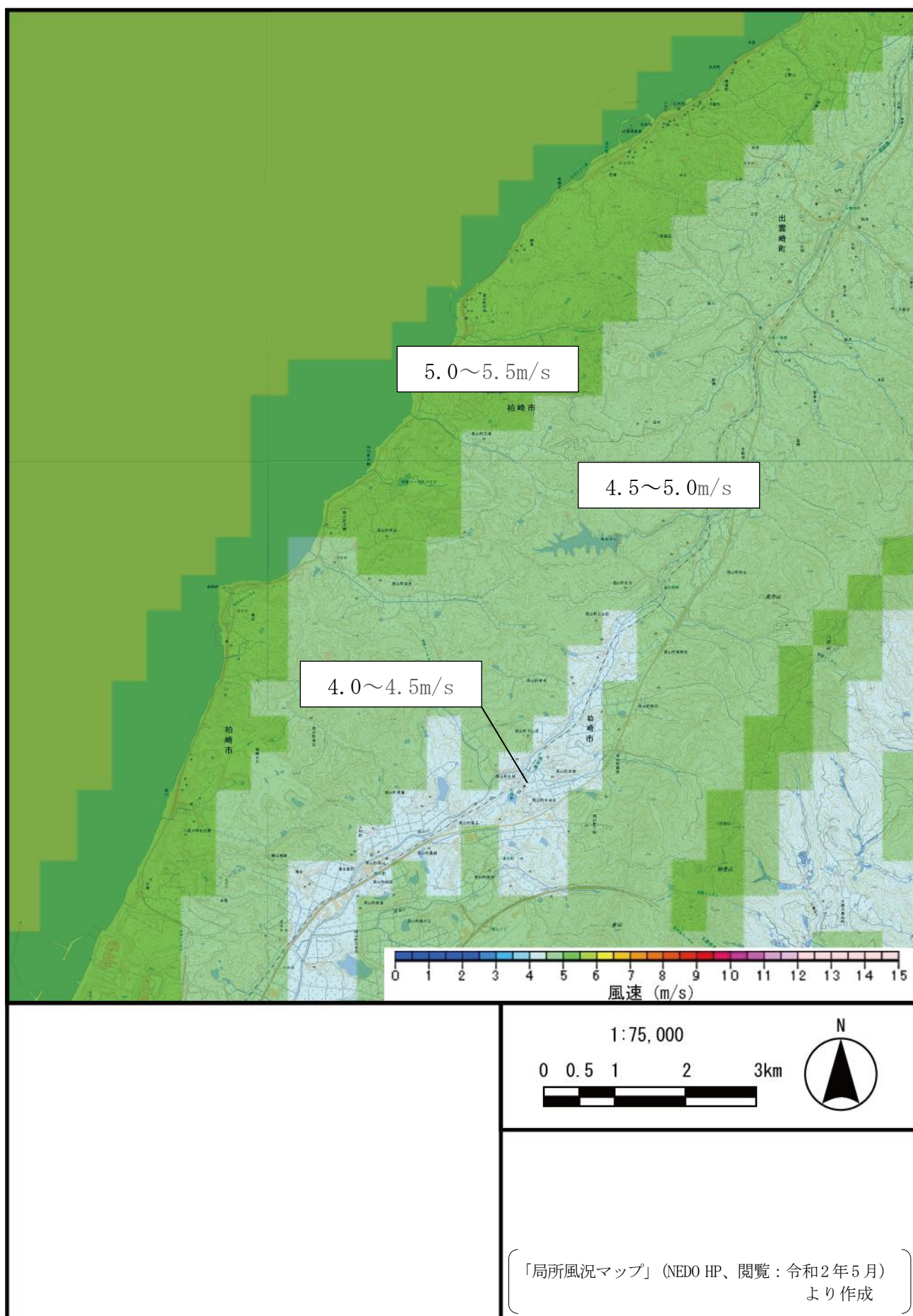
図 7.2-4(2) 検討対象エリアの風況（地上高 30m）
