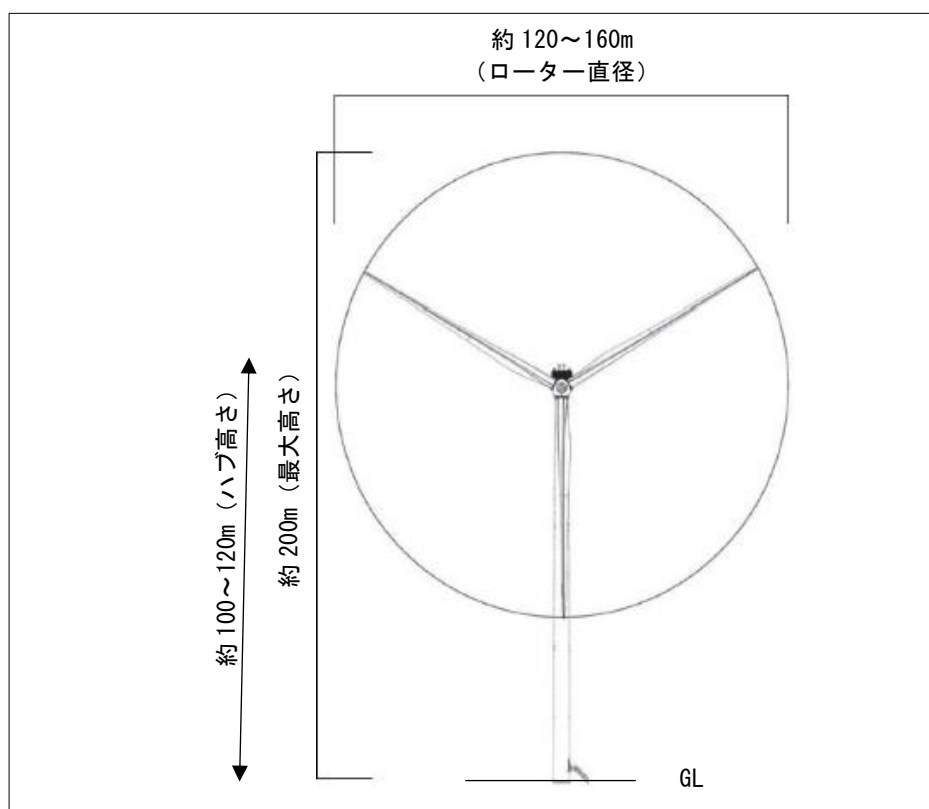
図 7.2-9 風力発電機の概略図
