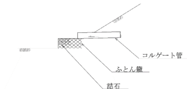
図2.2-7 沈砂池及びふとん籠の構造（例）
