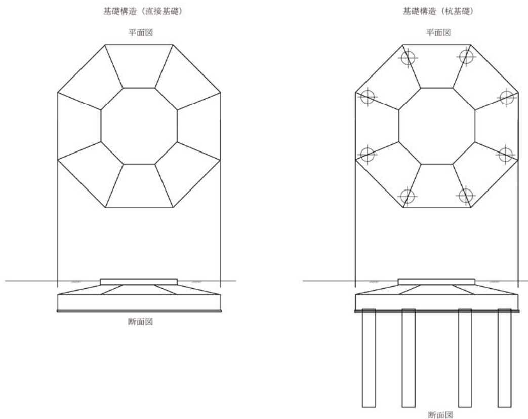
図2.2-4 風力発電機の基礎構造（例）
