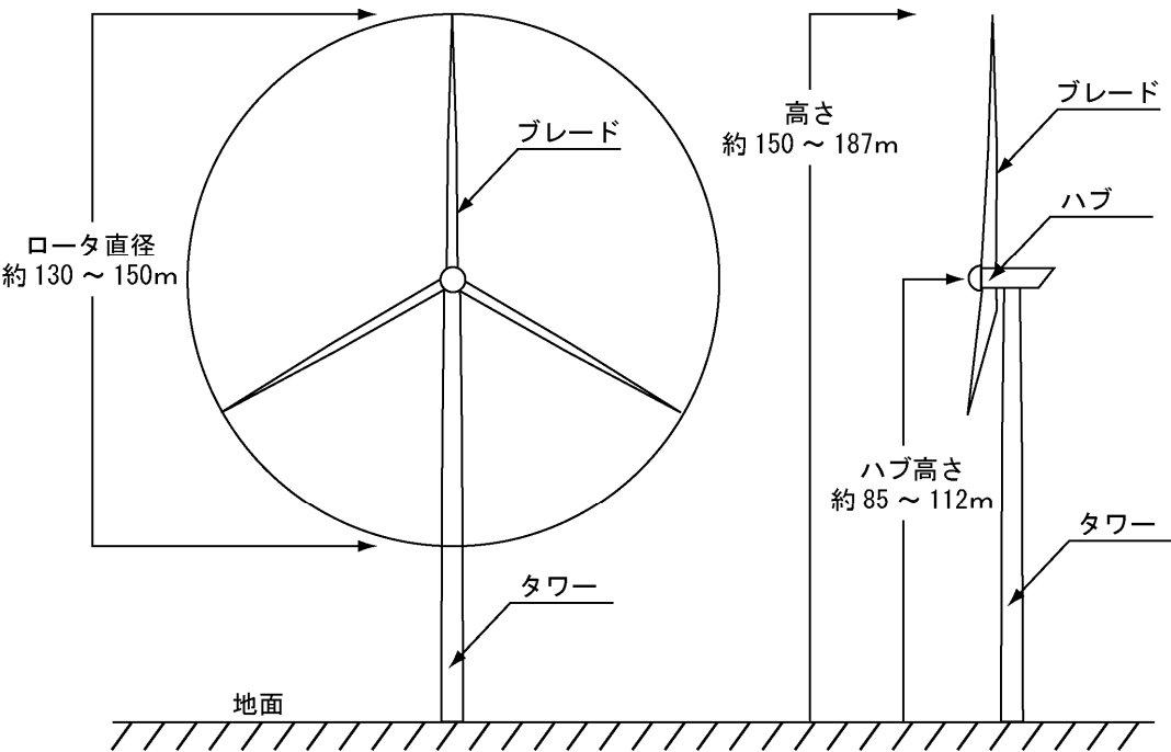
図2.2-3 風力発電機の概略図
