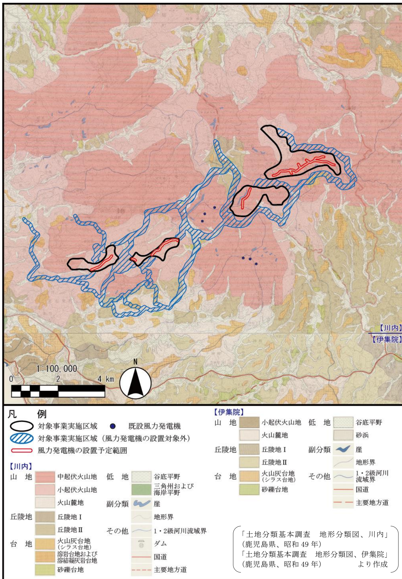
図 3.1-15 地形分類図
