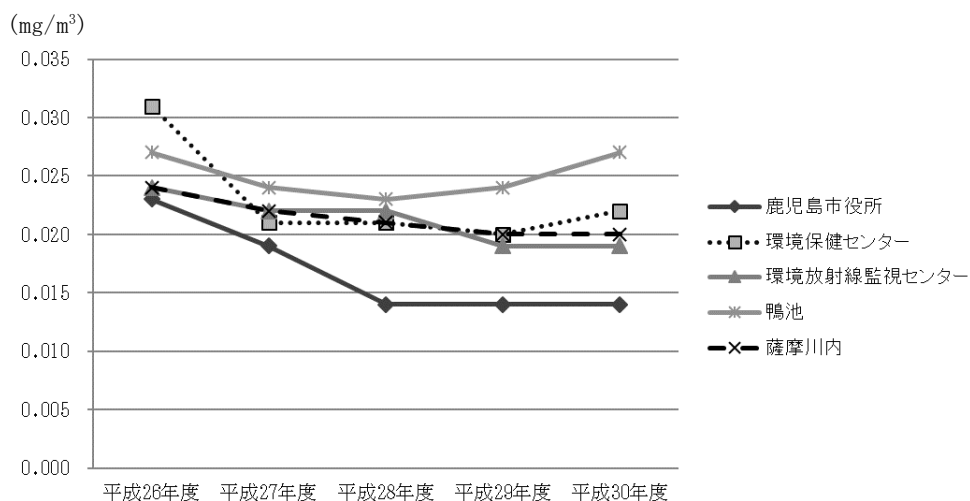
図 3. 1-7 浮遊粒子状物質の経年変化（平成 26～30 年度）
