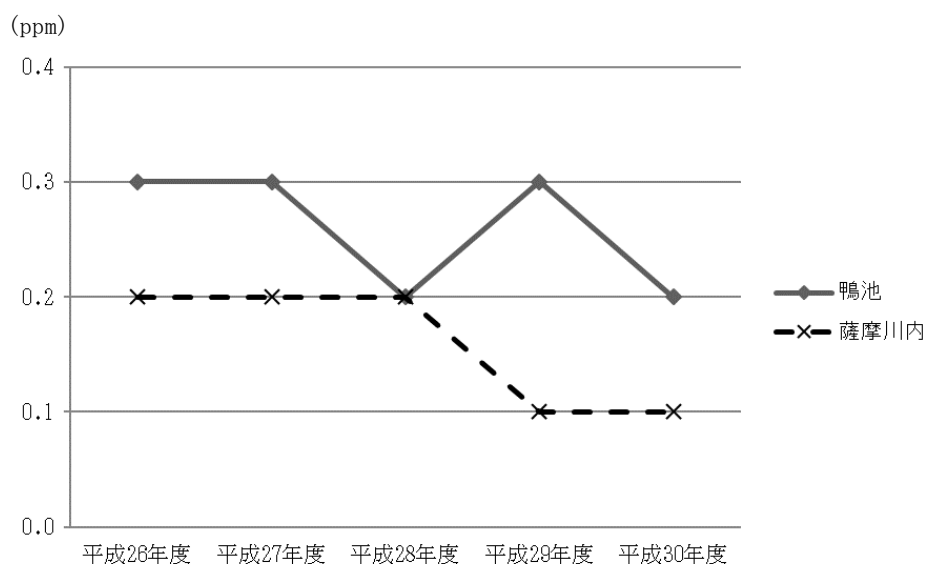
図 3.1-8 一酸化炭素の経年変化（平成 26～30 年度）
