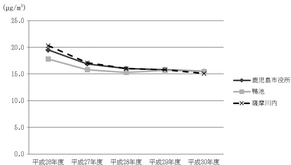
図 3.1-9 微小粒子状物質の経年変化（平成 26～30 年度）
