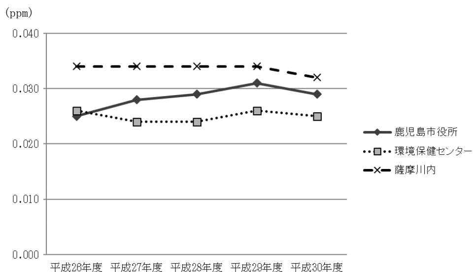
図 3.1-10 光化学オキシダントの経年変化（平成 26～30 年度）
