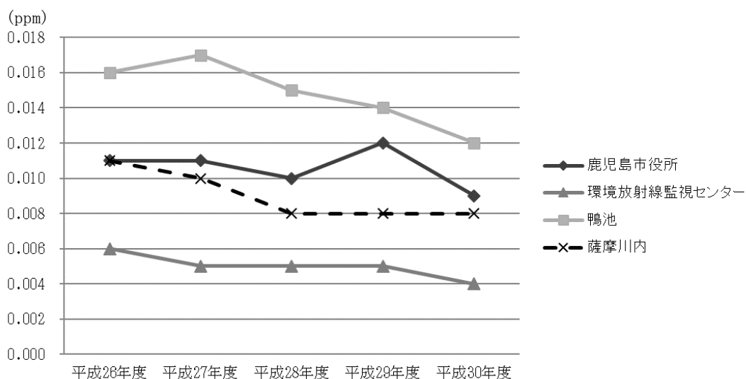
図 3.1-6 二酸化窒素の経年変化（平成 26～30 年度）
