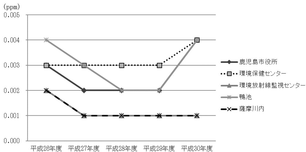
図 3.1-5 二酸化硫黄の経年変化（平成 26～30 年度）
