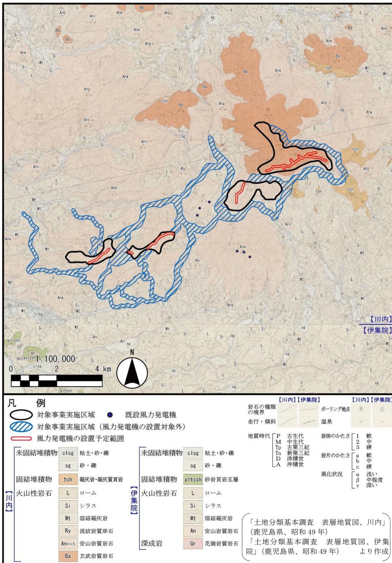
図 3.1-16 表層地質図
